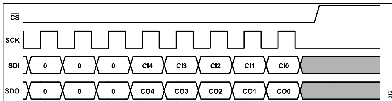
Figure 13. CRC Byte
