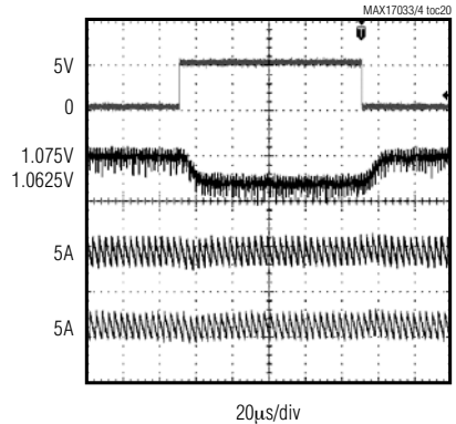
MAX17034 D0 12.5mV DYNAMIC VID CODE CHANGE
