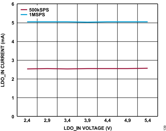
Figure 34. LDO_IN Current vs. LDO_IN Voltage
