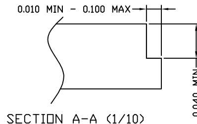
SECTION A-A (1/10)
