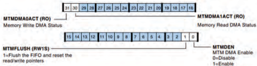
Figure A-7. MTMCTL Register (RW)
