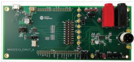
图58. MAX22513评估套件
