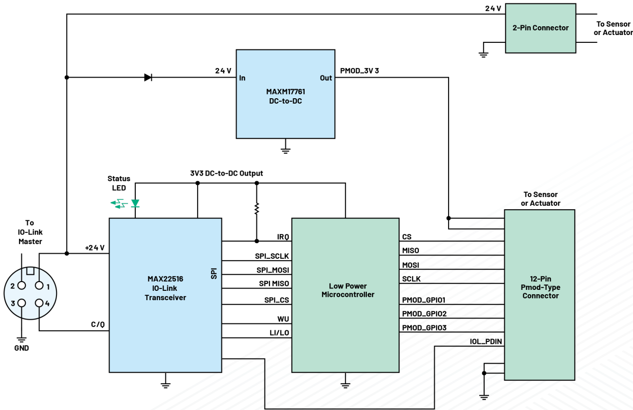
图25. MAXREFDES281#/MAXREFDES284#系统框图
