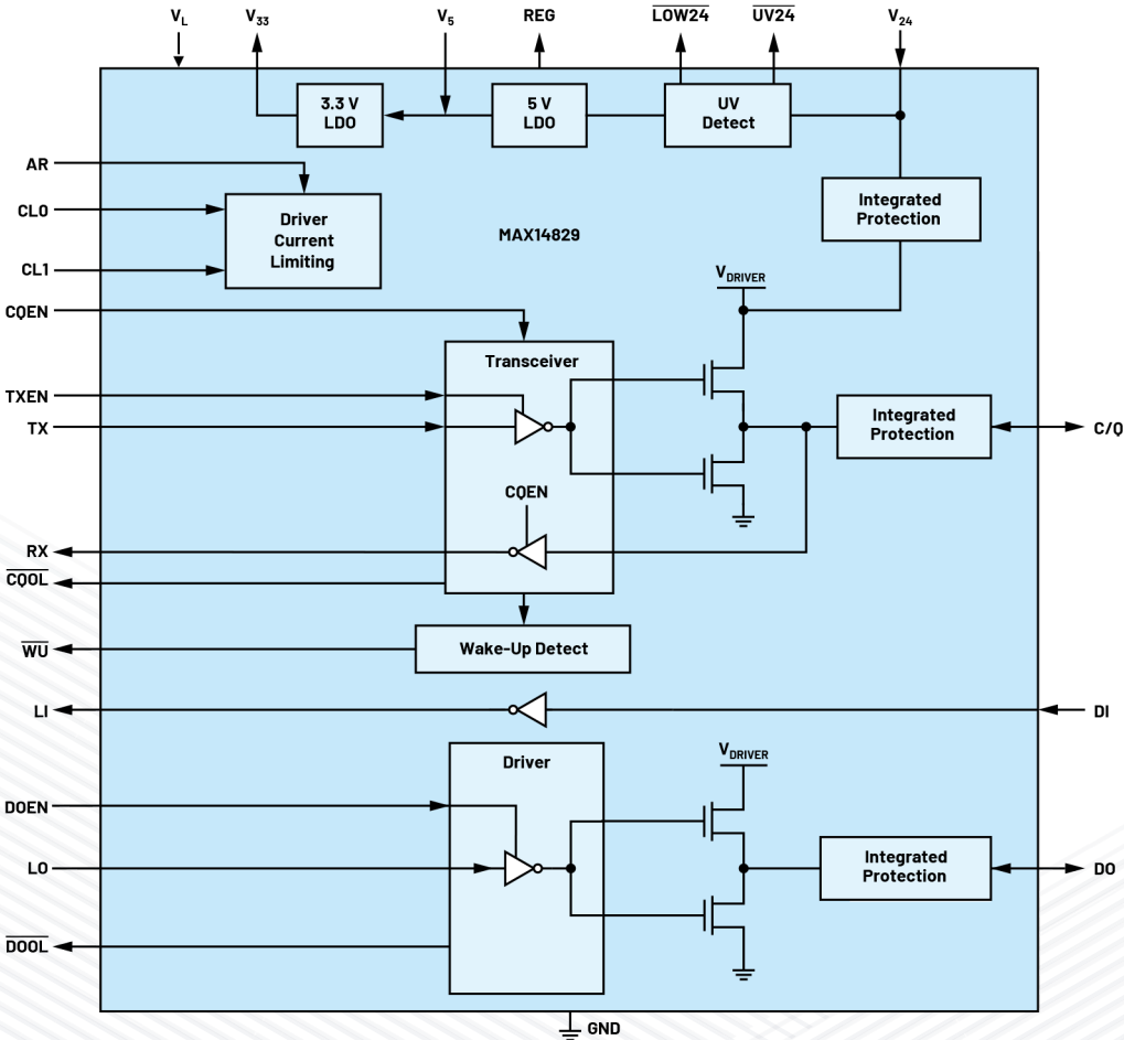
图53. MAX14829引脚控制、双通道IO-Link收发器
