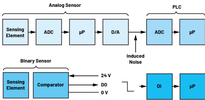
图1. “老式”传感器：模拟和二进制
