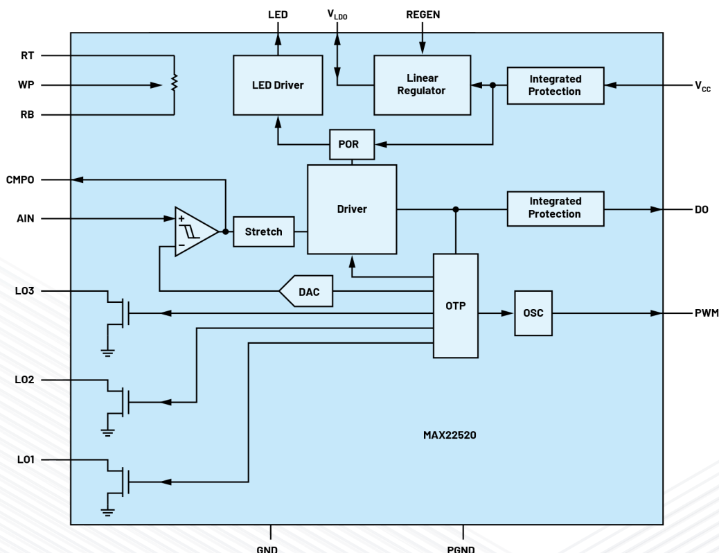
图51. MAX22520 OTP工业传感器输出驱动器
