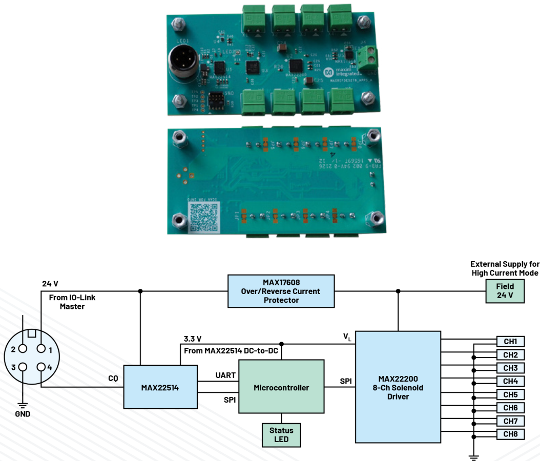
图27. MAXREFDES278电磁阀执行器
