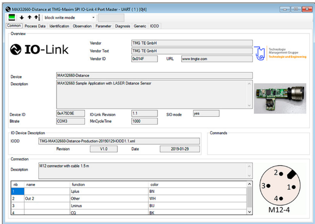
图22. MAXREFDES171 IO-Link从站软件接口
