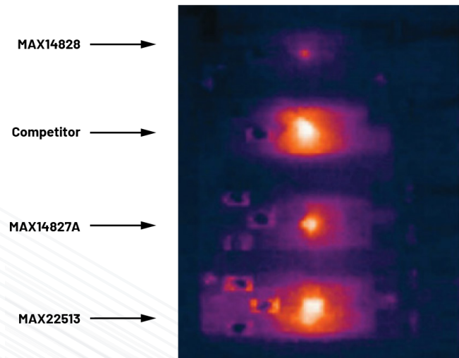
图40. 测试A：每个器件200 mA
