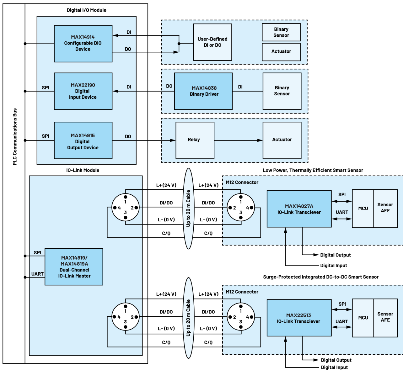
图10. 工业传感器生态系统
