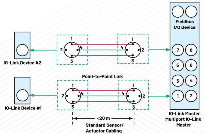
图3. IO-Link主站/从站接口
