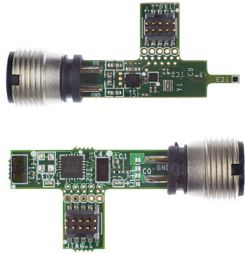
图18. MAXREFDES164温度传感器和MAXREFDES171距离传感器
