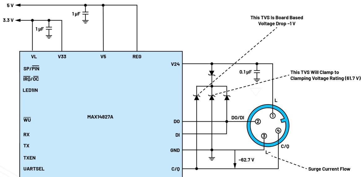
图46. C/O到L+浪涌
