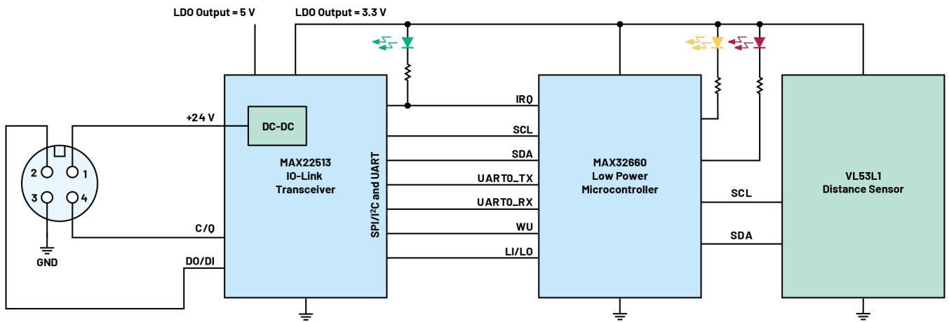
图21. MAXREFDES171 IO-Link从站距离传感器
