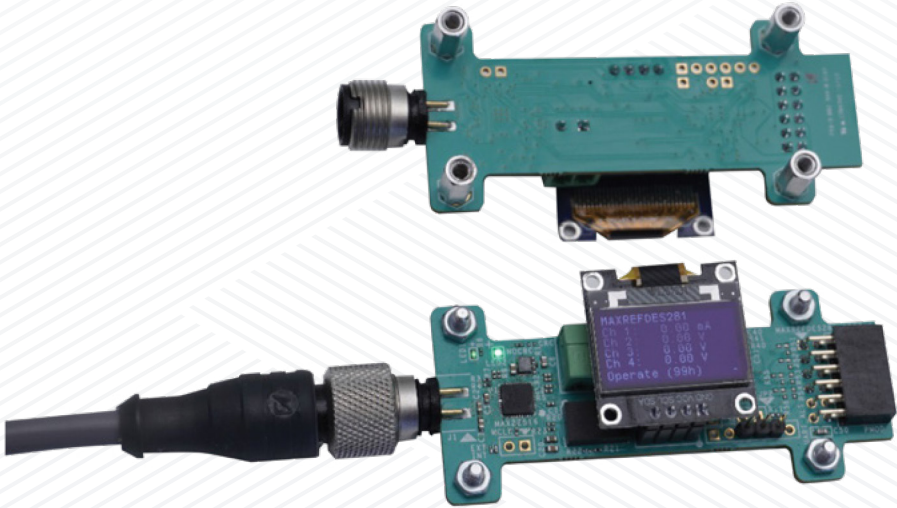
图26. MAXREFDES281#/MAXREFDES284# IO-Link至外设器件
