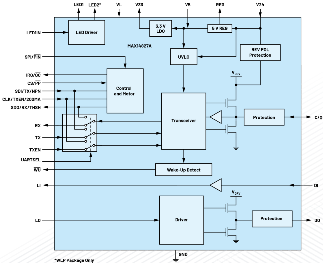
图52. MAX14827A双通道IO-Link收发器
