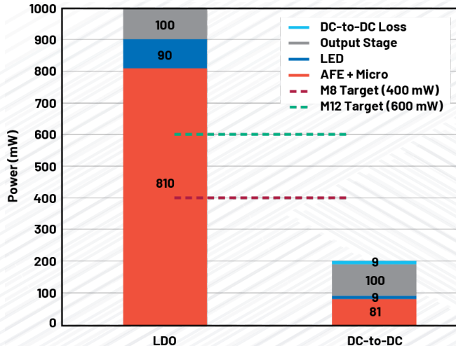
图44. 对于30 mA传感器，使用降压转换器与使用LDO稳压器的功耗降幅对比
