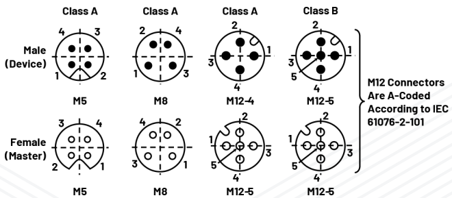
图7. 备选IO-Link连接器
