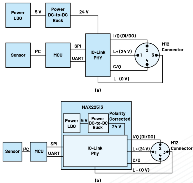
图17. (a) IO-Link传感器的构建模块，(b)高集成度IO-Link传感器的构建模块
