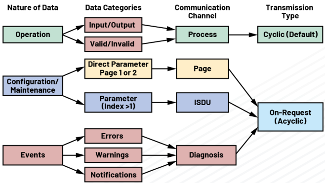
图11. IO-Link传输类型
