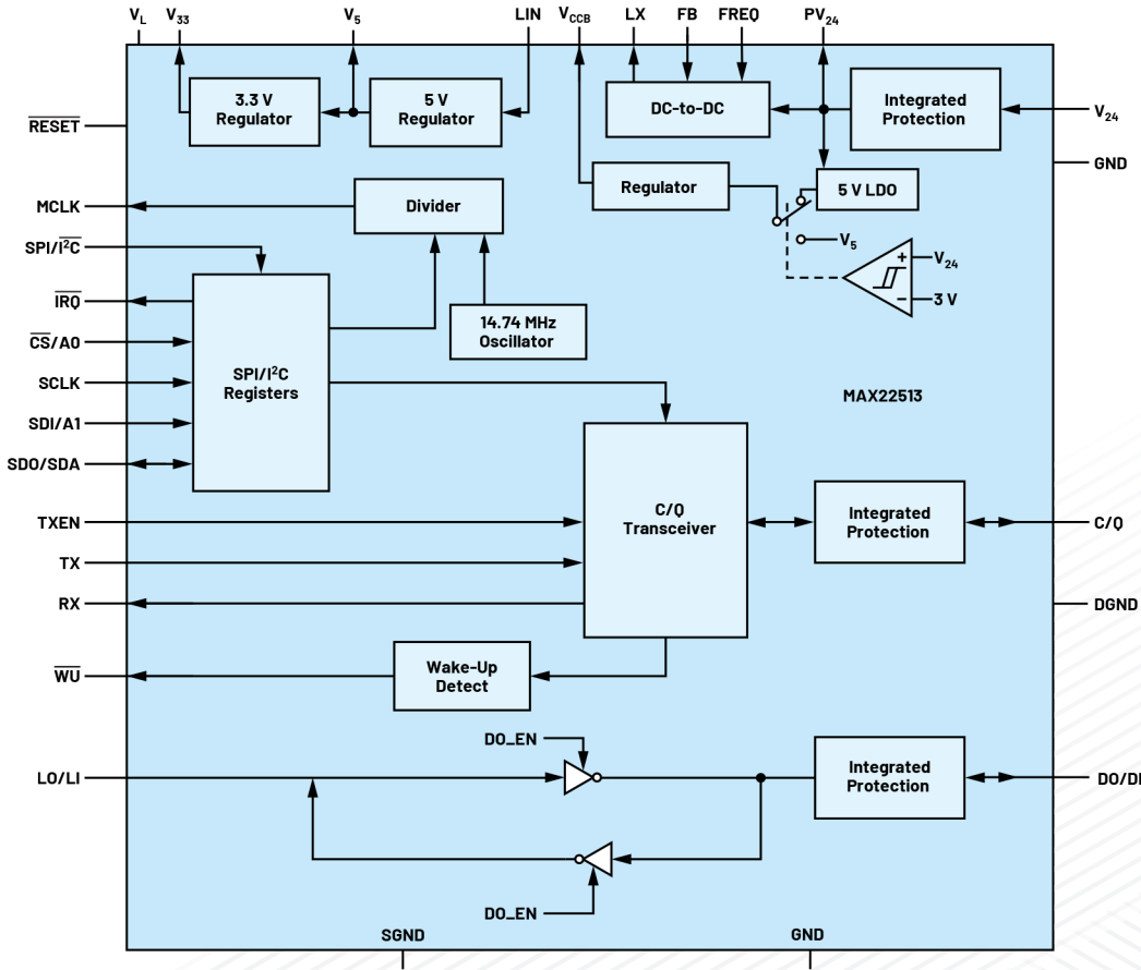
图54. 带DC-DC转换器的MAX22513双通道IO-Link收发器
