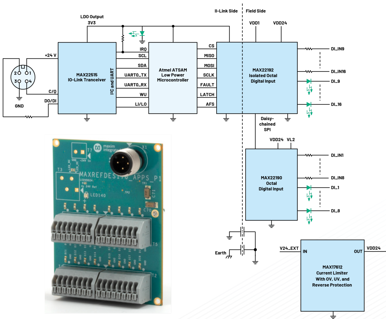
图23. MAXREFDES176数字输入集中器
