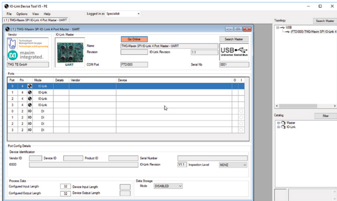
图35. MAXREFDES165 TMG IO-Link从站工具
