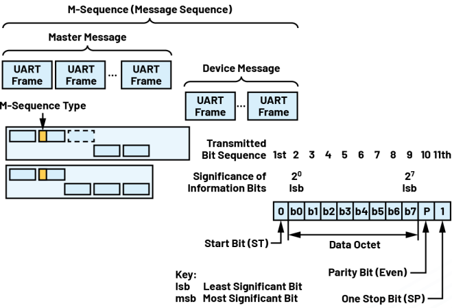
图12. IO-Link主站-从站通信序列
