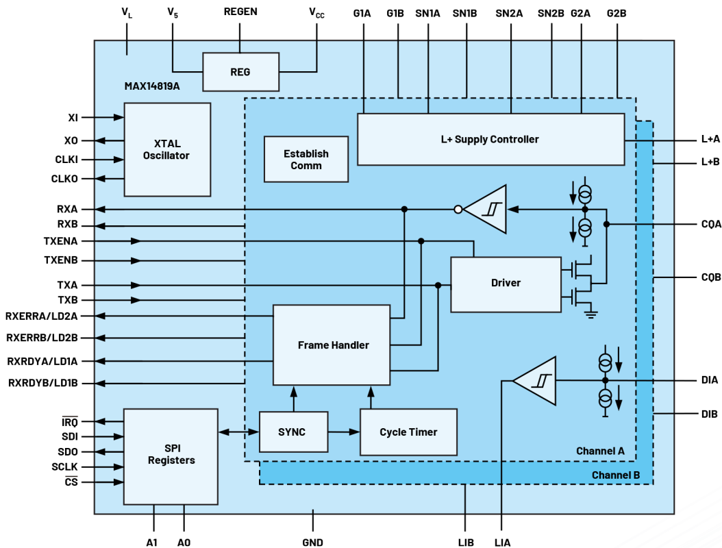
图57. MAX14819A双通道IO-Link主站收发器
