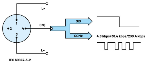
图6. IO-Link引脚定义
