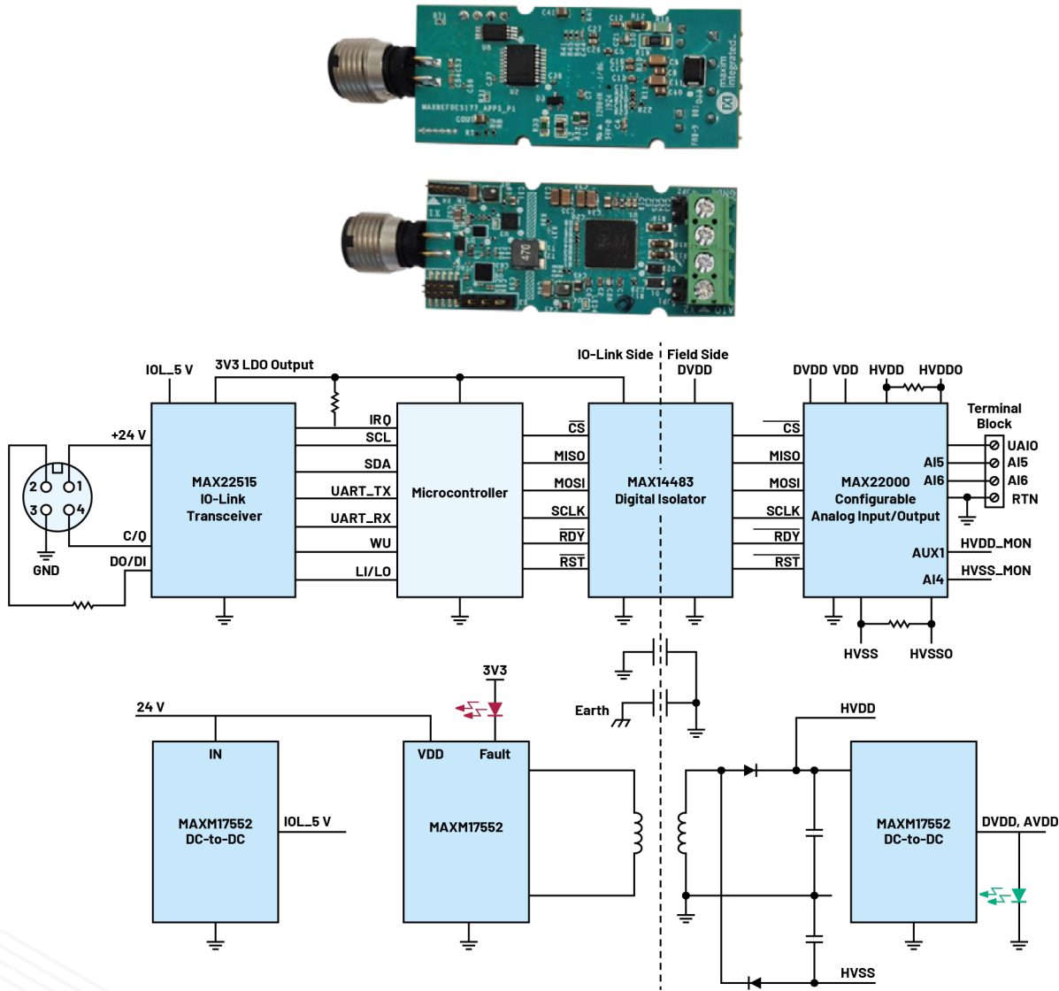
图24. MAXREFDES177通用模拟I/O
