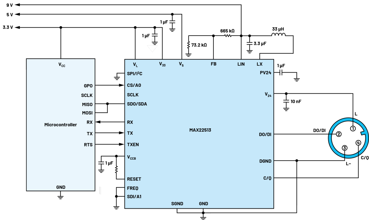
图45. 集成DC-DC转换器的MAX22513 IO-Link收发器
