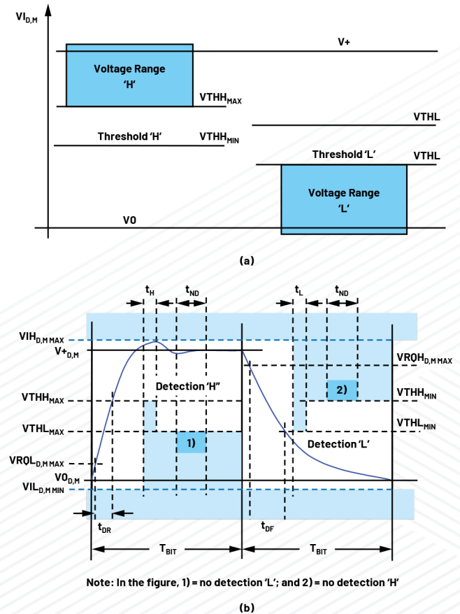
图8. (a) IO-Link信号电气阈值；(b) IO-Link信号电气特性。
