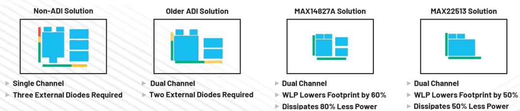
图49. IO-Link收发器解决方案比较
