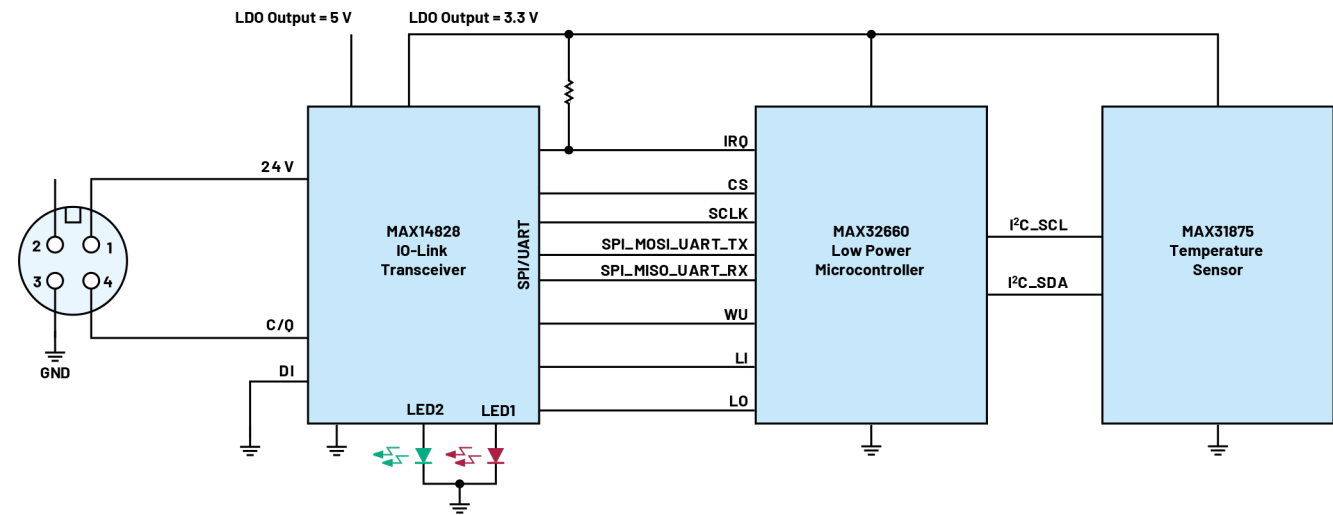
图19. MAXREFDES164 IO-Link温度传感器框图
