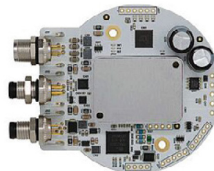
图29. TMCM-1617-GRIP-REF开源硬件参考设计
