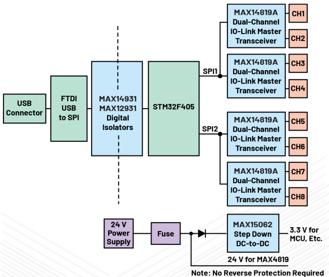
图31. MAXREFDES145 8端口IO-Link主站框图
