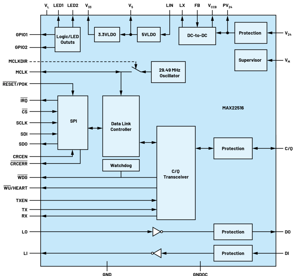
图56. 带收发器和集成DC-DC控制器的MAX22516 IO-Link数据链路控制器
