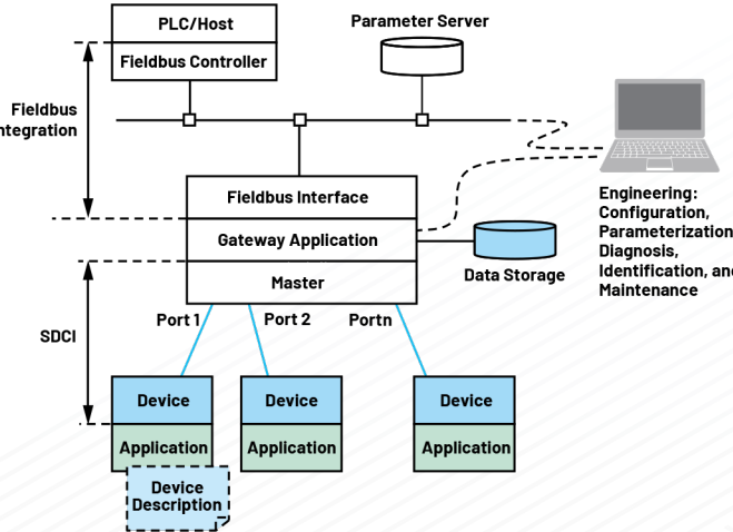
图9. IO-Link现场总线互连
