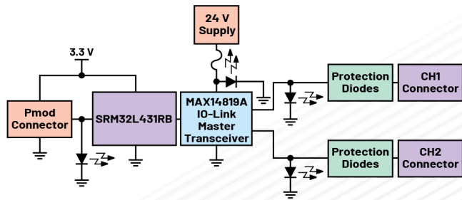
图36. MAXREFDES277#框图
