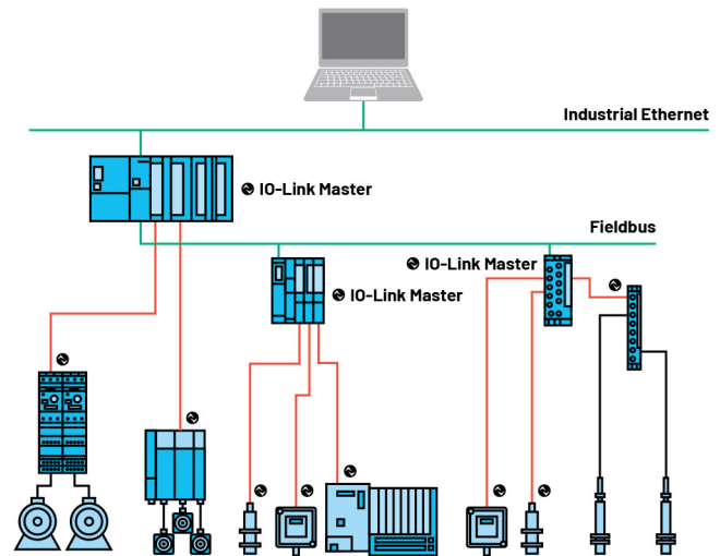
图5. IO-Link与现有行业协议的兼容性
