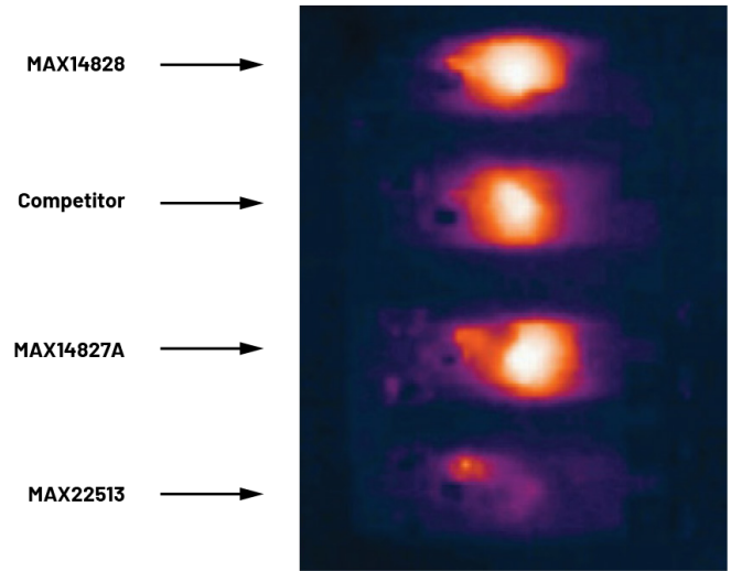
图42. 测试C：5 V LDO稳压器上30 mA负载
