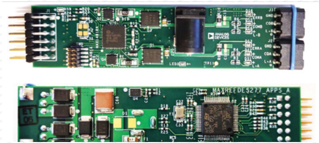
图37. MAXREFDES277# IO-Link至外设器件（顶部和底部）
