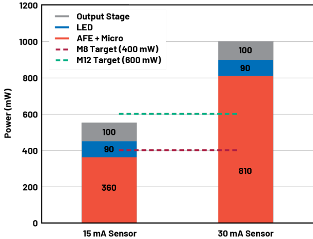
图43. 典型的LDO稳压器供电的IO-Link传感器的功耗预算
