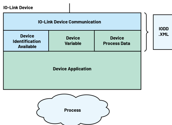
图16. IODD文件
