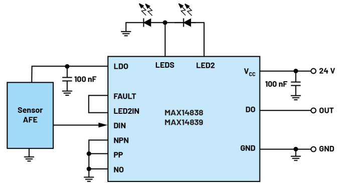
图2. 24 V引脚可配置工业传感器输出驱动器
