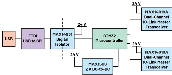
图34. MAXREFDES165参考设计框图
