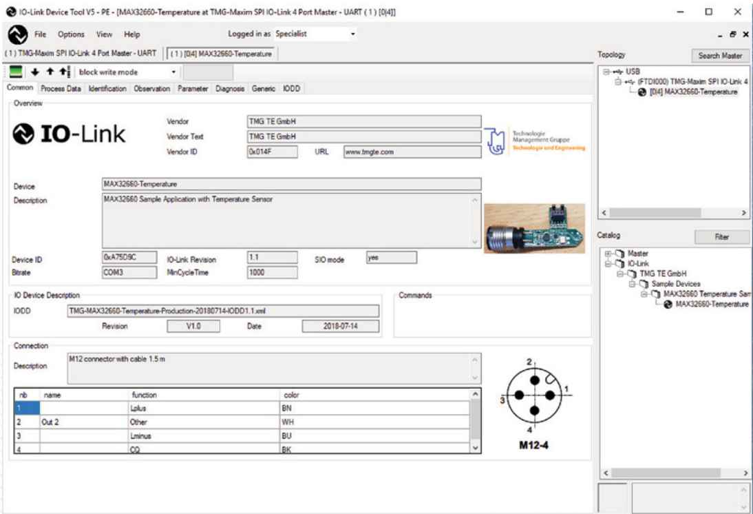
图20. MAXREFDES164 IO-Link从站软件接口
