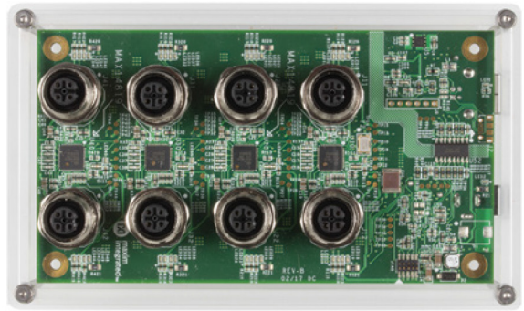
图30. MAXREFDES145 8端口IO-Link主站参考设计
