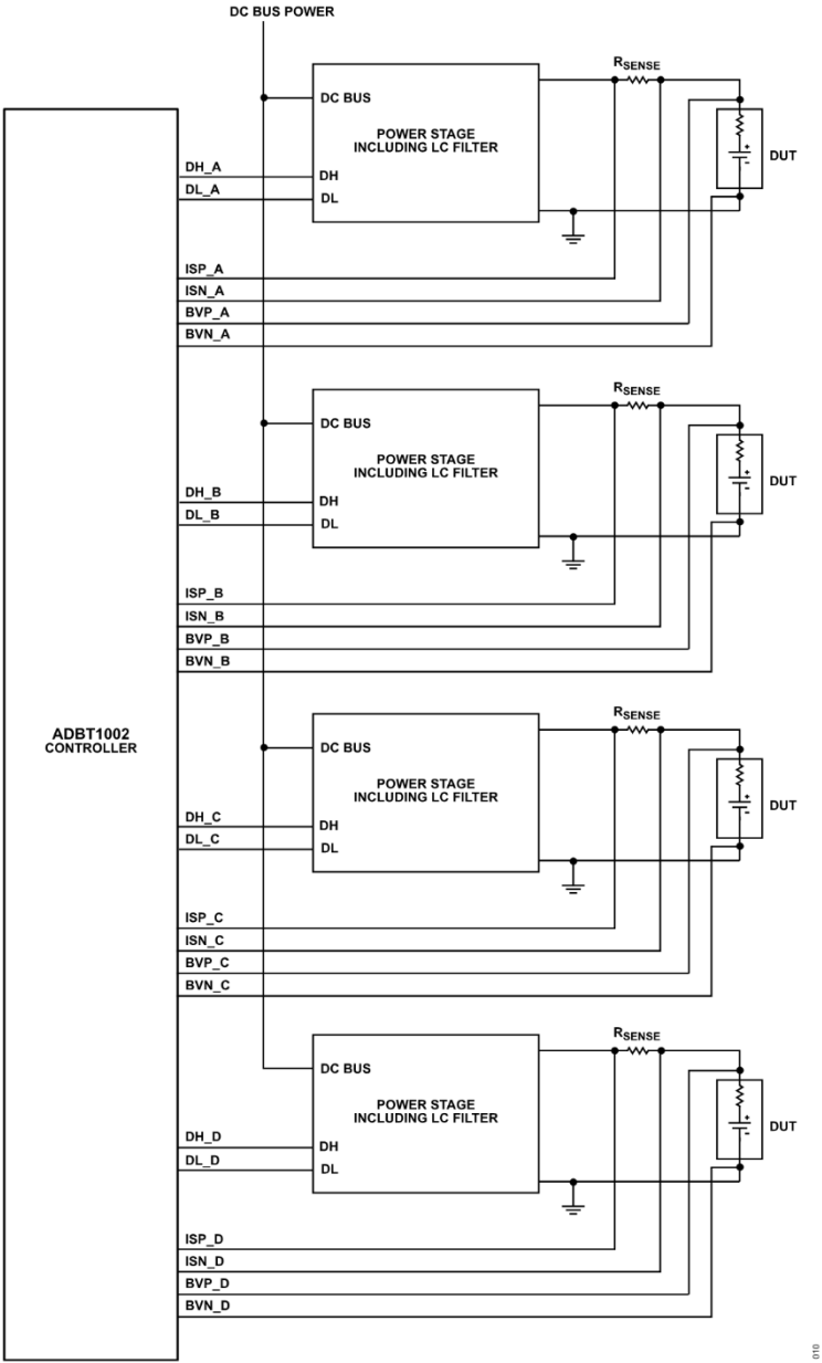
图 10. 四通道独立应用案例
