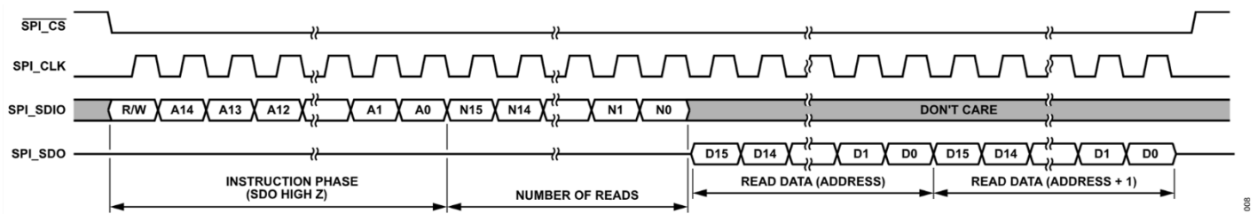
图 8. 基本 4 线读操作
