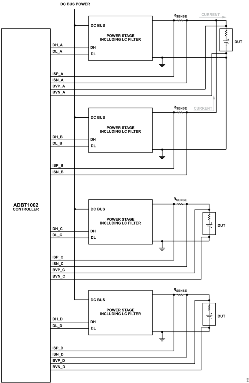
图 11. 两个并联、两个独立通道应用案例
