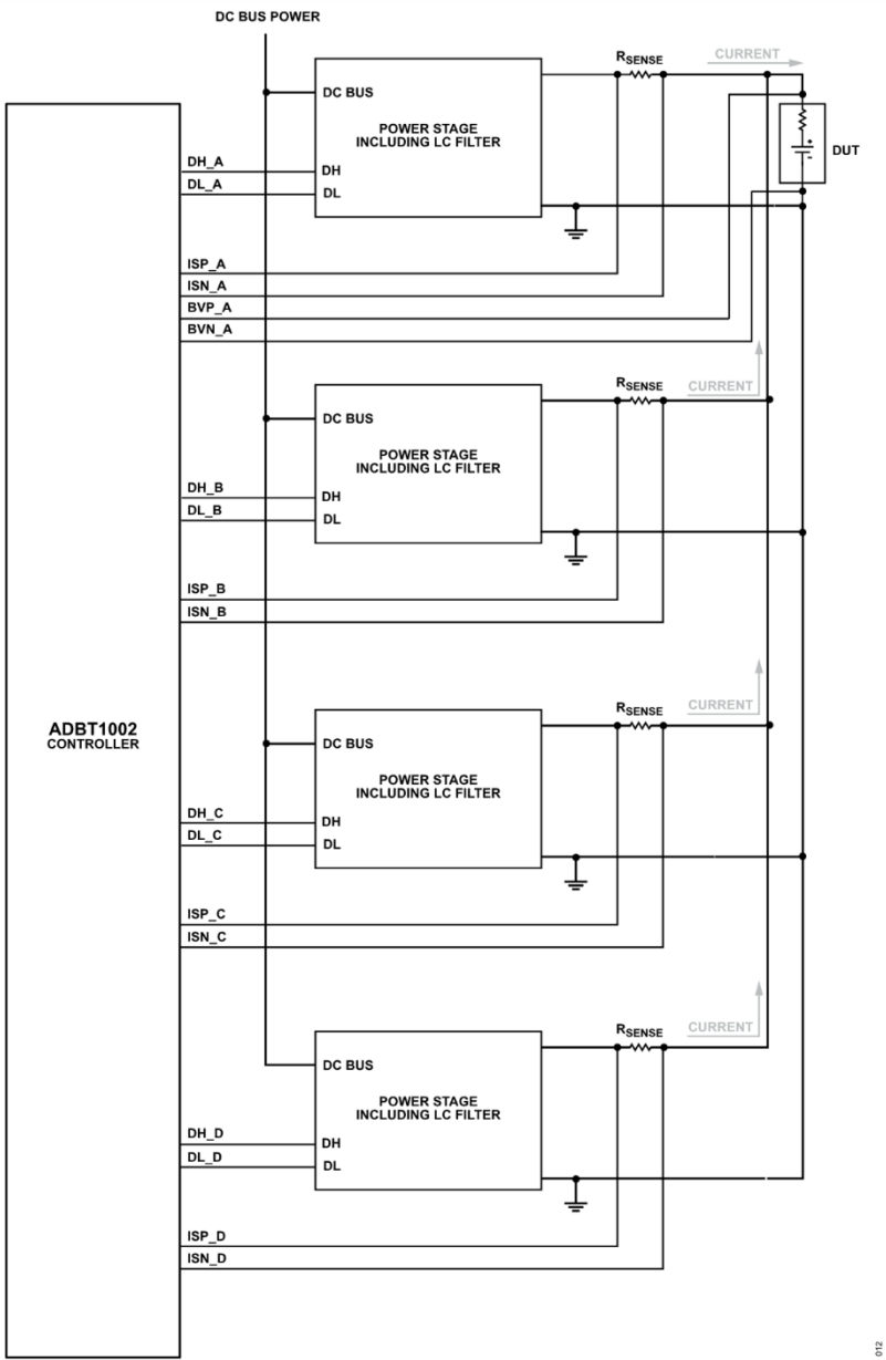
图 12. 四通道并联应用案例
