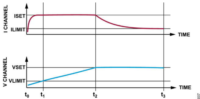
图 7. 恒流至恒压操作
