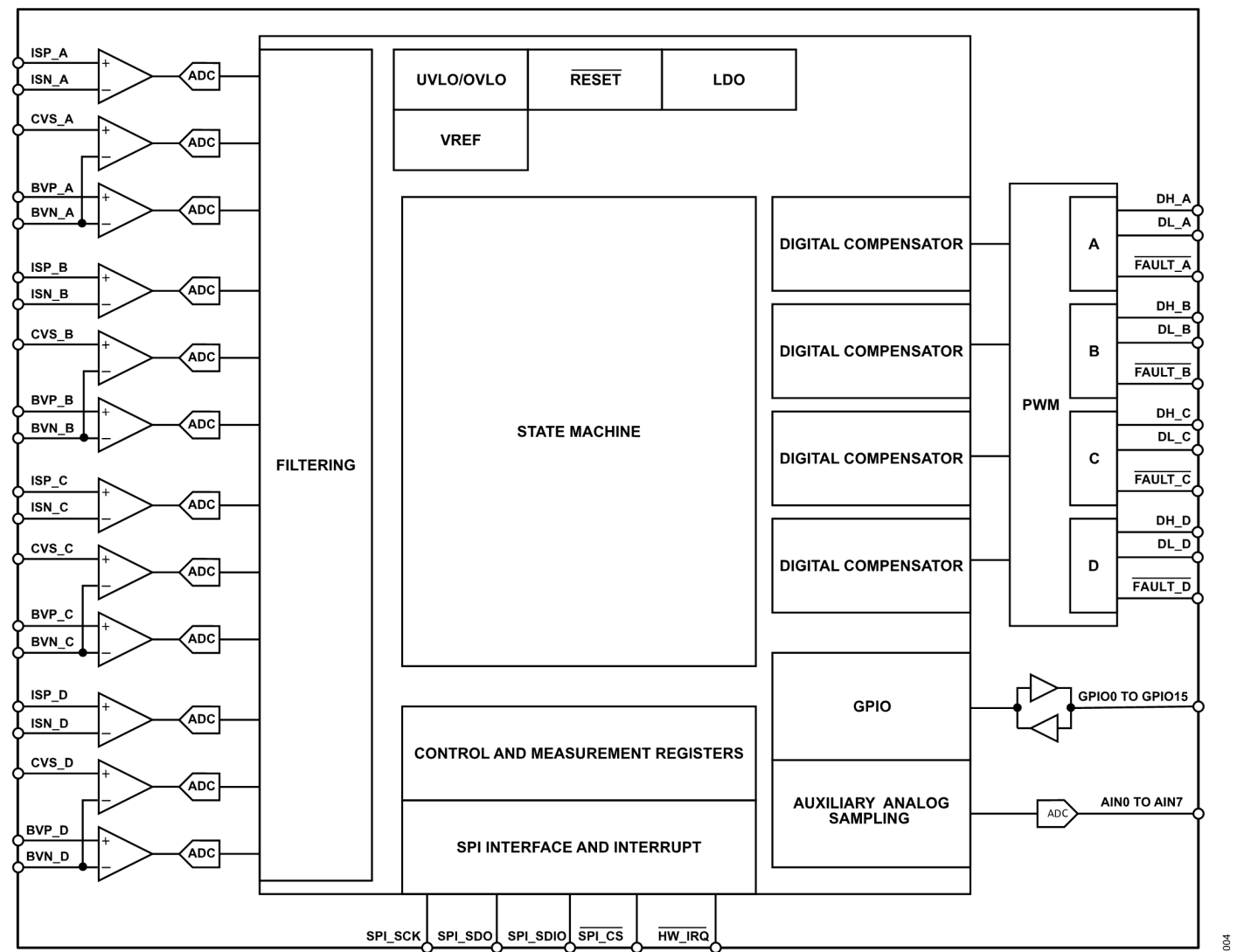
图 4. 功能框图
