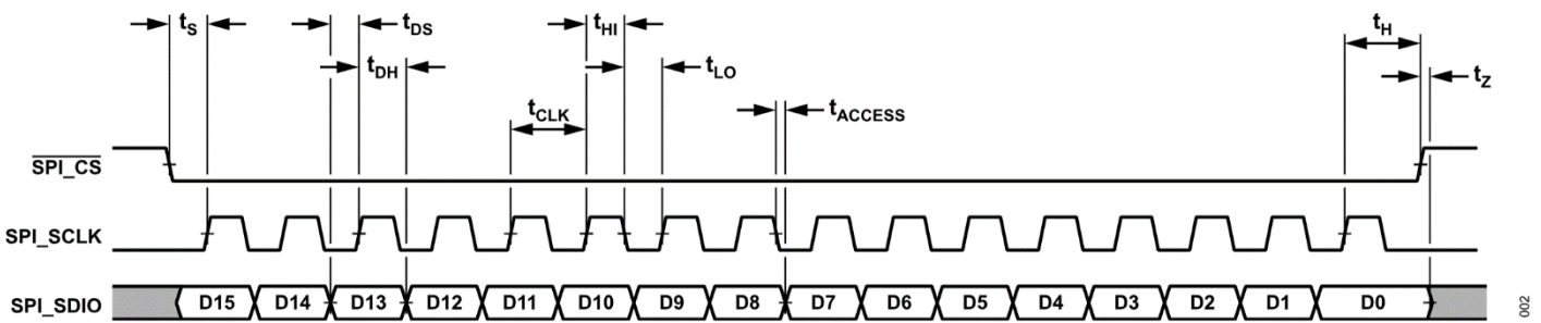
图 2. 三线 SPI 总线时序图
