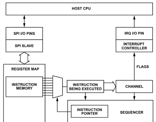
图 6. 自动序列化模式
