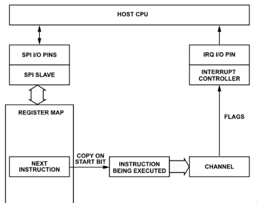
图 5. 手动序列化模式
