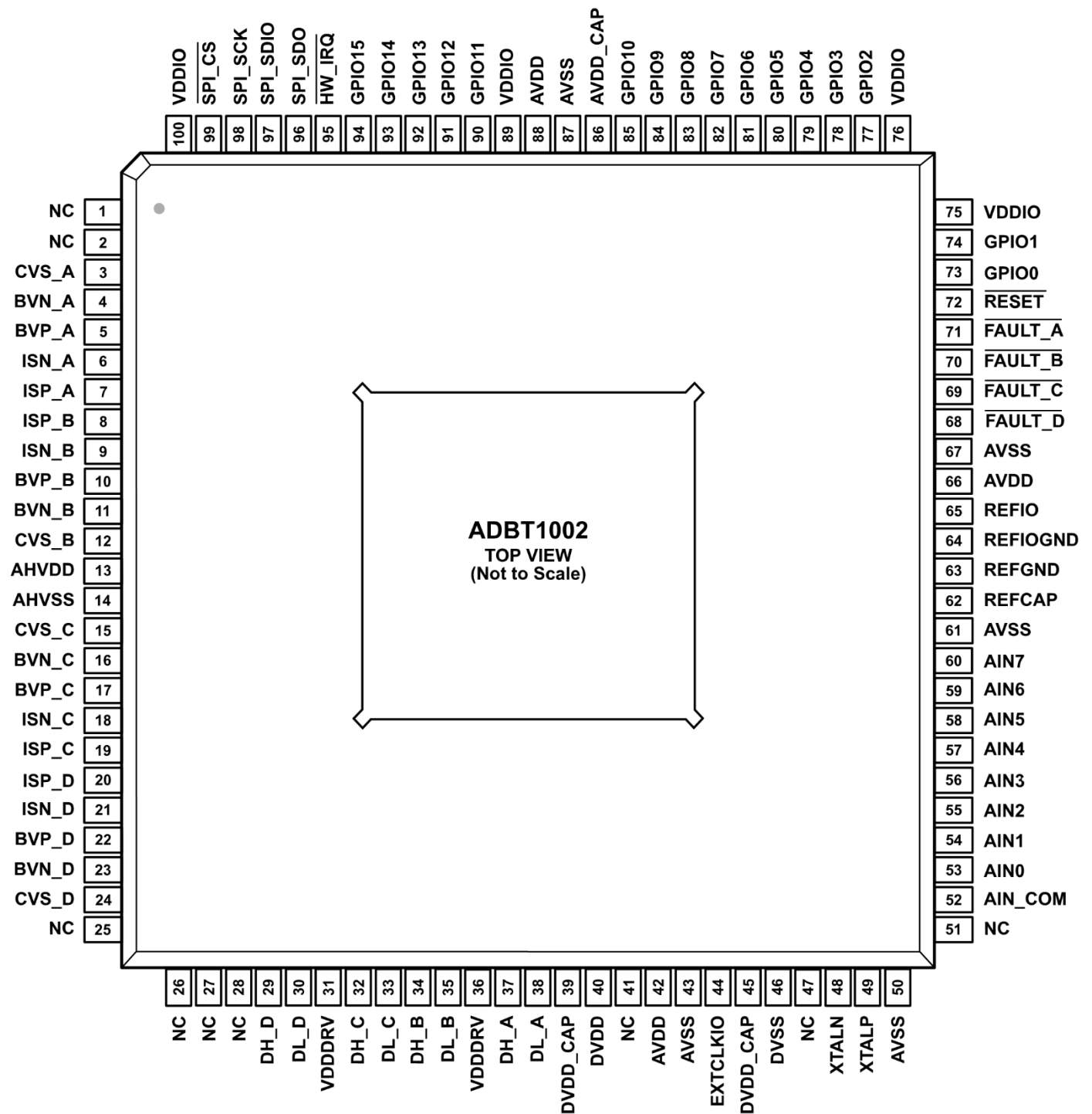
图 3. 引脚配置
