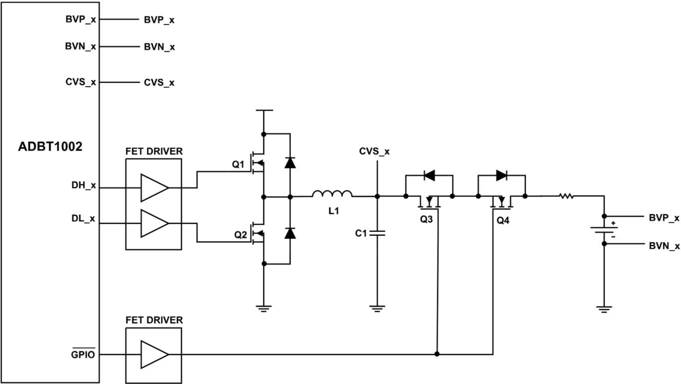
图 13. 预充电功能框图
