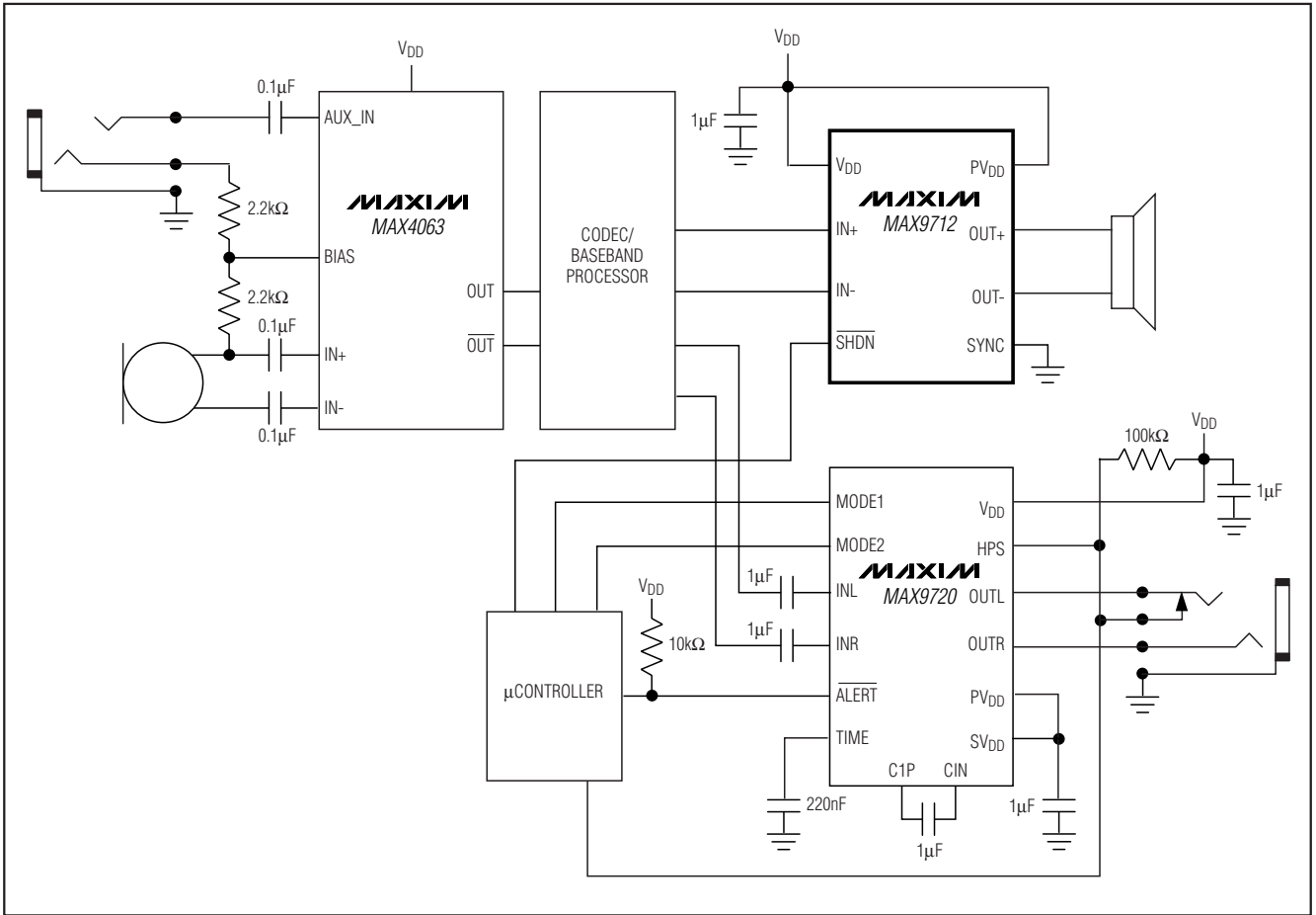
系统原理图
