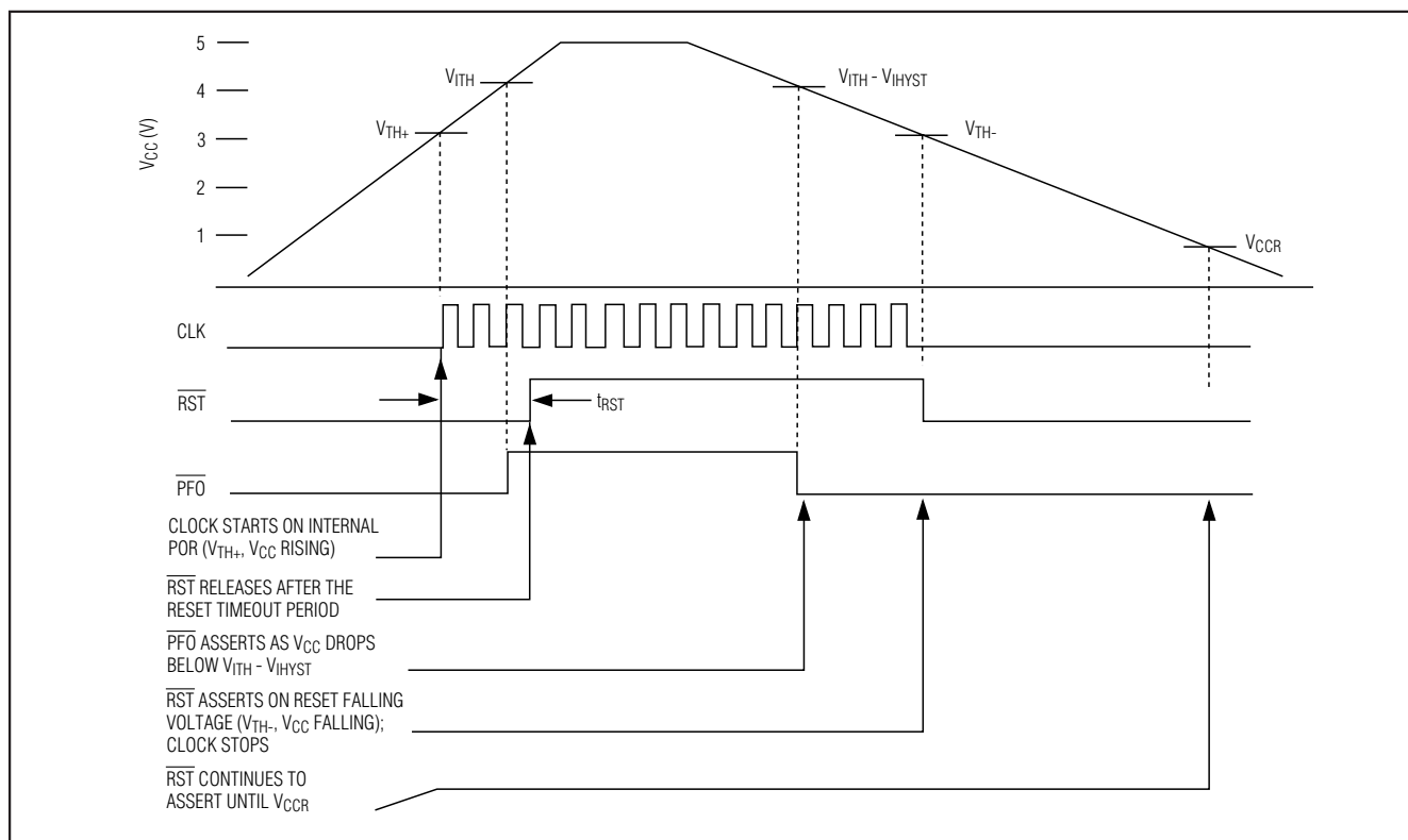
图1. 上电和断电期间的RST/ \overline{\text{RST}} 、 \overline{\text{PFO}} 过程
