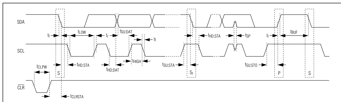
图1. I 2 C串口时序图
