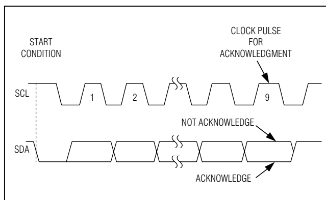
图3. I 2 C应答
