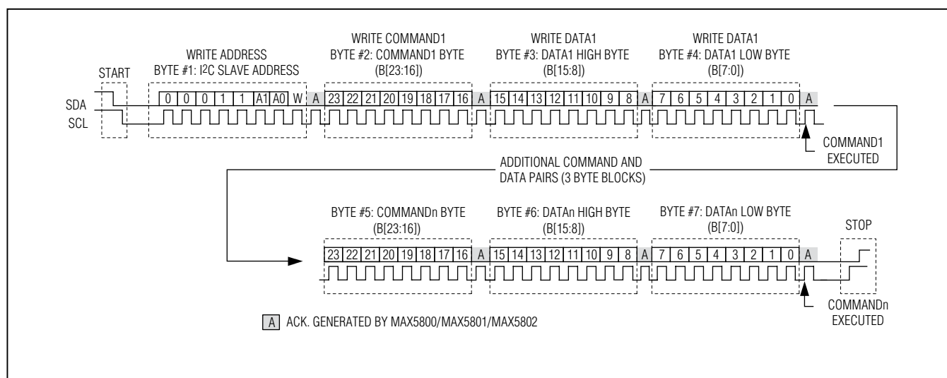
图5. 多个寄存器写序列(标准I 2 C协议)
