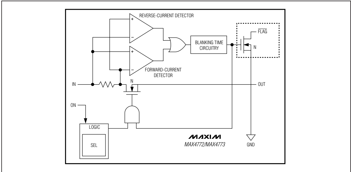
图1. 原理框图
