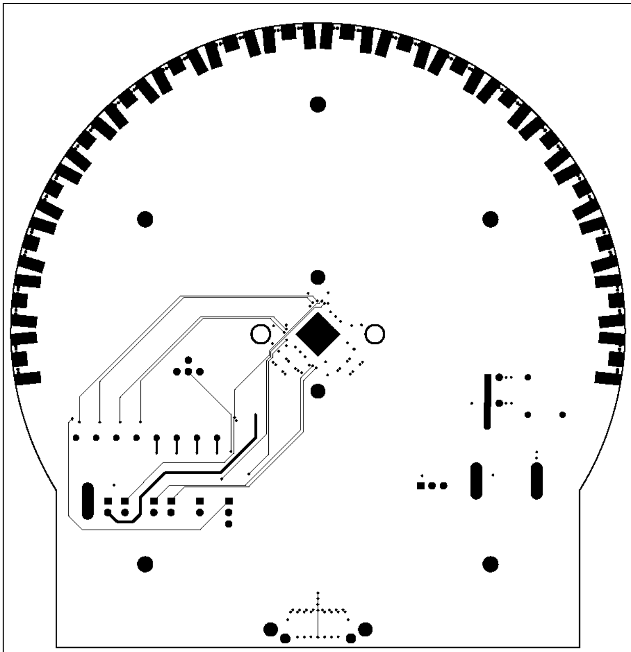
图8. MAX3983 评估板 PC 板布局 —— 底层(信号), 第6层
