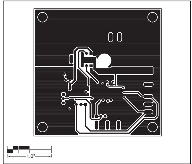
图4. MAX1748评估板PCB布局—焊接层
