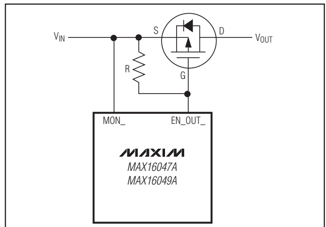
图17. p沟道串联MOSFET的连接
