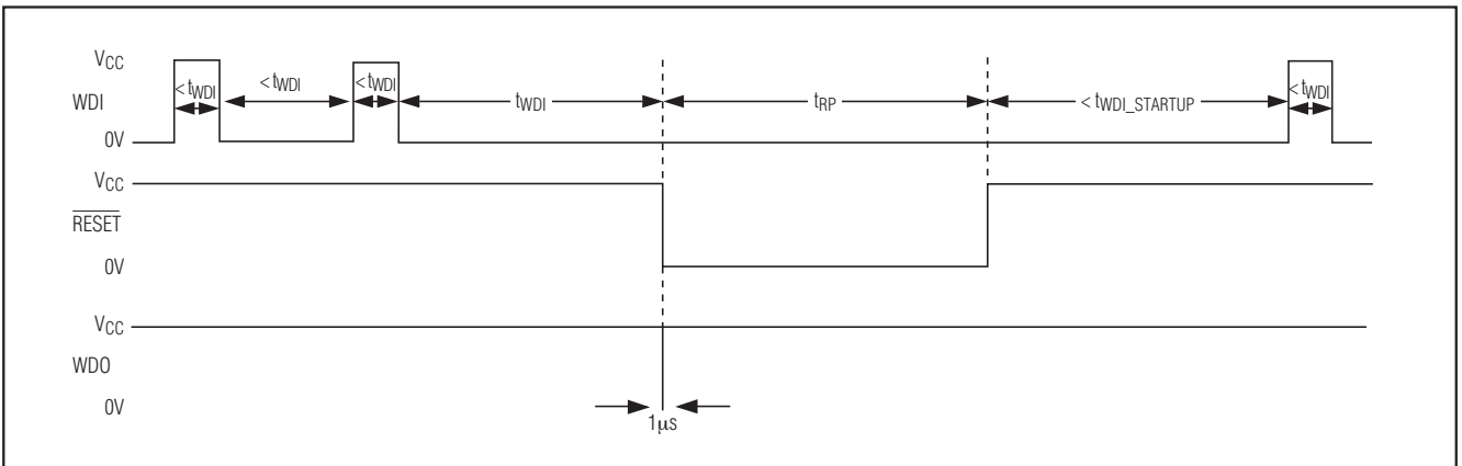
图8. 看门狗启动过程，看门狗RESET输出使能位(i:55h[7])置‘1’
