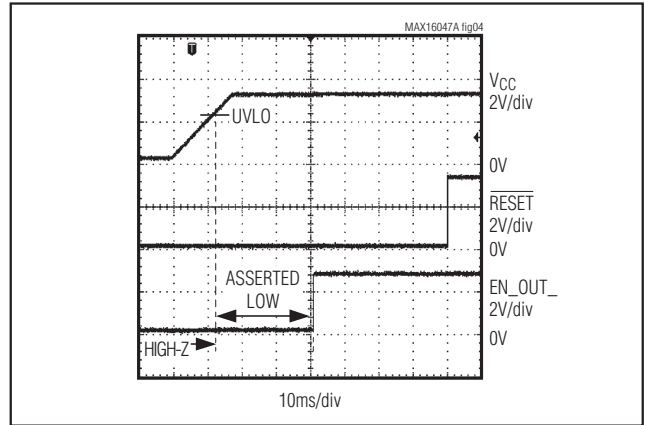
图4. 上电期间的RESET和EN_OUT_，EN_OUT_配置为高电平有效的推挽式输出
