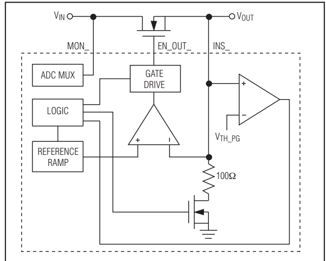
图16. 闭环跟踪
