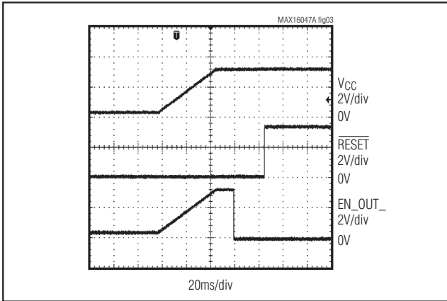
图3. 上电期间的RESET和EN_OUT_，EN_OUT_配置为低电平有效的漏极开路输出
