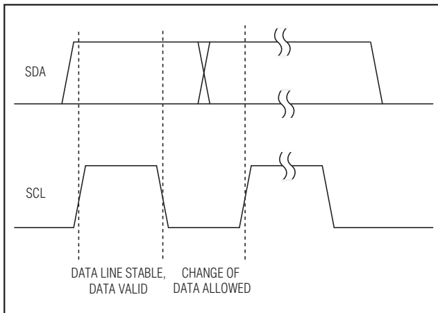
图9. 位传输
