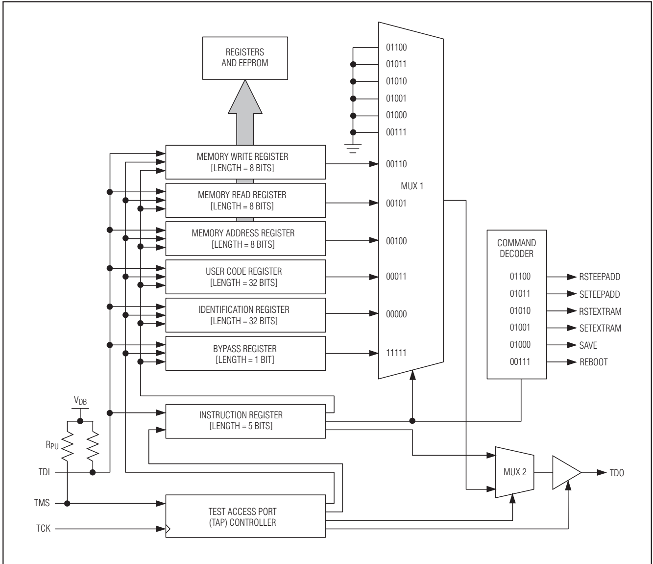
图13. JTAG方框图
