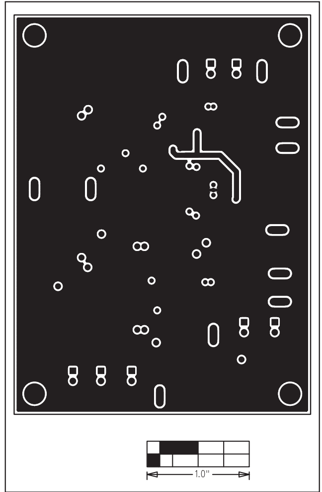
图5. MAX1537评估板PCB布局—第3层
