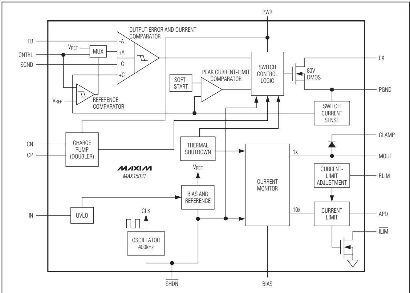
功能框图
