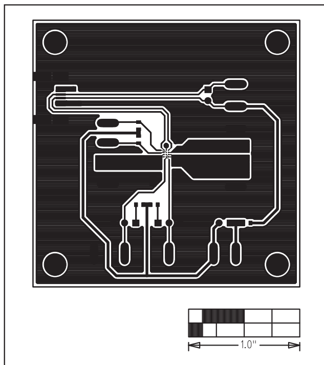
图3. MAX14529E评估板PCB布局—元件层
