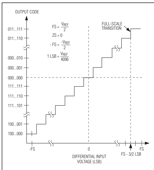
图9. 双极性传输函数(MAX1225)
