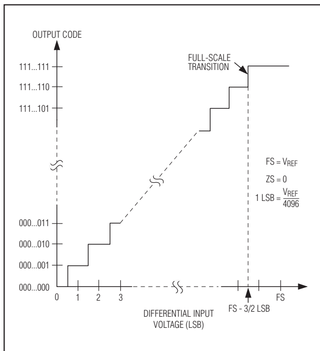
图8. 单极性传输函数(MAX1224)
