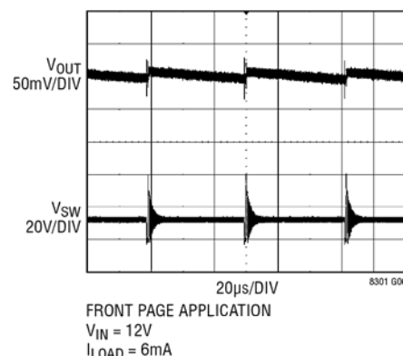
Burst 模式波形
