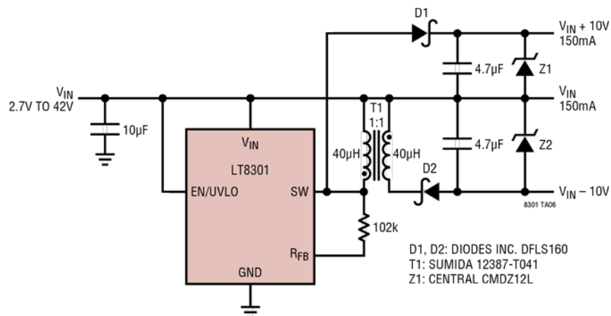
V_{IN} 至 (V_{IN} + 10V)/(V_{IN} - 10V) 微功耗转换器
