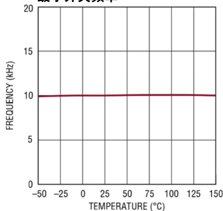
最小开关频率
