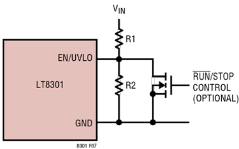
图 7. 欠压闭锁 (UVLO)
