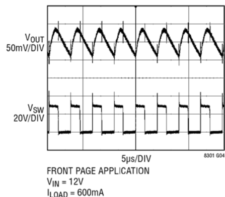
边界模式波形
