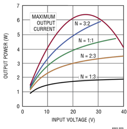
图 2. 5V 输出的输出功率
