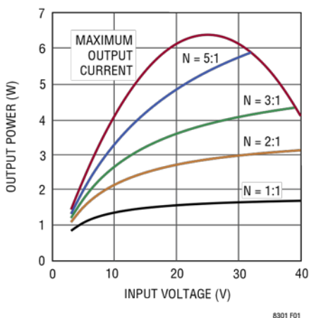
图 1. 3.3V 输出的输出功率
