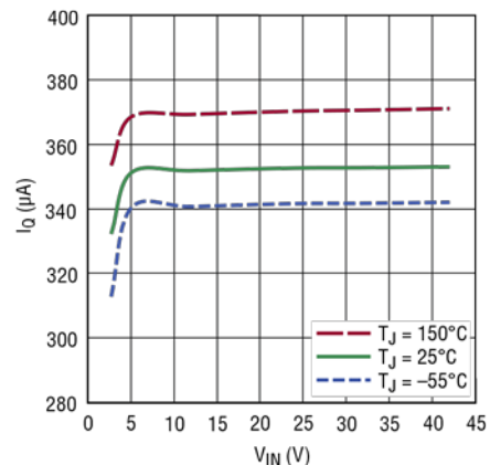
活动模式 V_{IN} 静态电流
