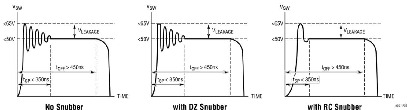
图 5. SW 引脚反激波形的最大电压
