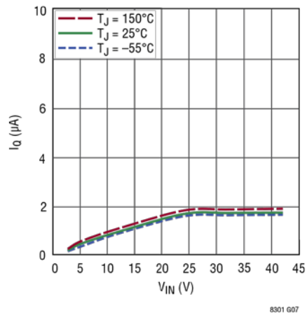
V_{IN} 关断电流
