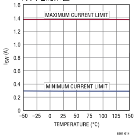
开关电流限值
