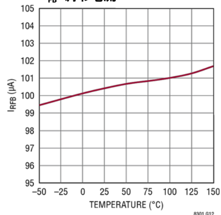
R_{FB} 调节电流
