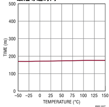
最短导通时间
