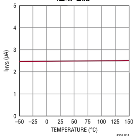
EN/UVLO 迟滞电流
