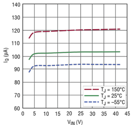
睡眠模式 V_{IN} 静态电流
