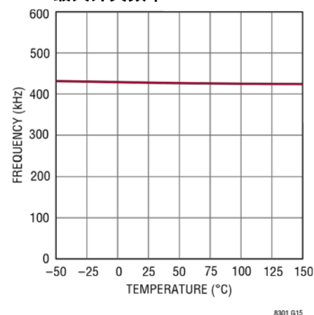
最大开关频率
