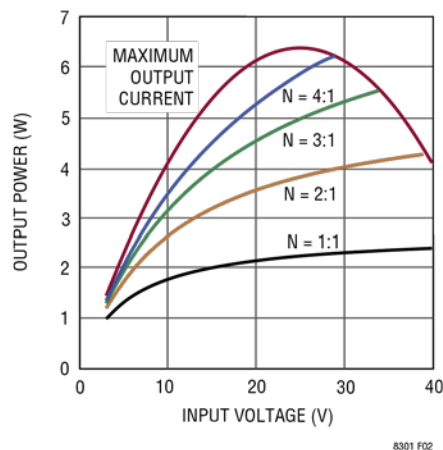
图 3. 12V 输出的输出功率
