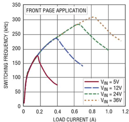
开关频率与负载电流的关系
