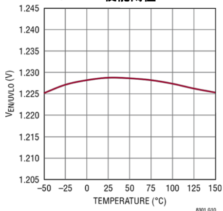
EN/UVLO 使能阈值
