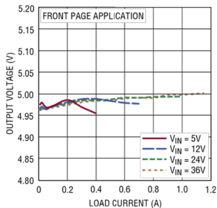
输出负载和电压调整率
