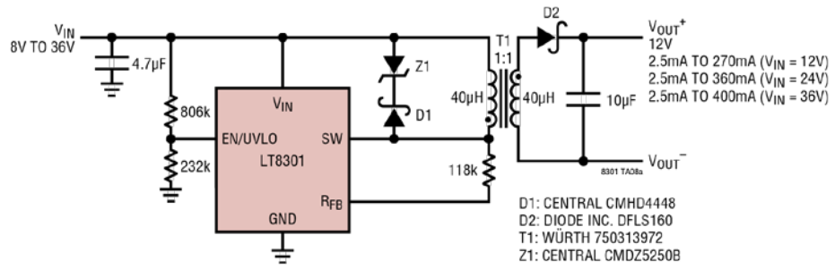
8V 至 36V IN /12V OUT 微功耗隔离型反激式转换器
