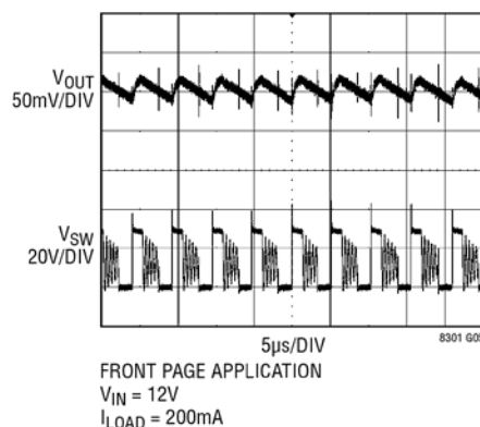
断续模式波形
