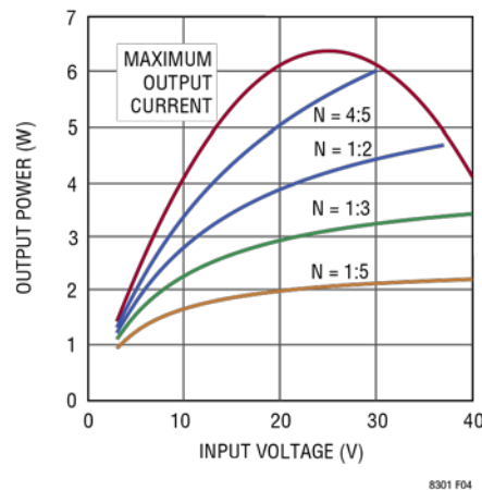
图 4. 24V 输出的输出功率
