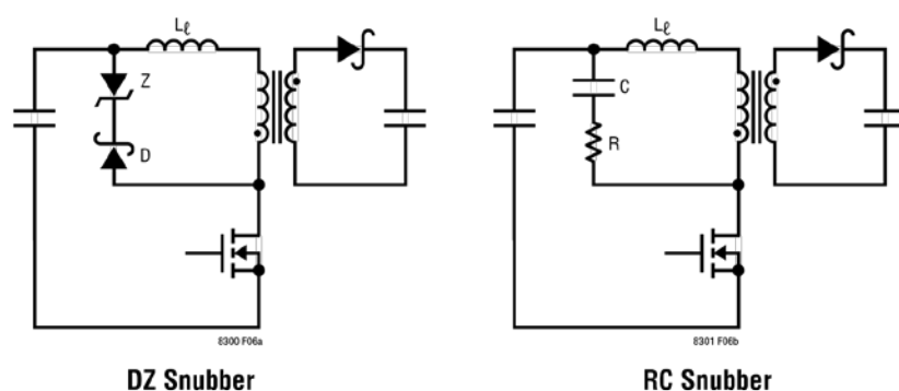
图 6. 缓冲器电路
