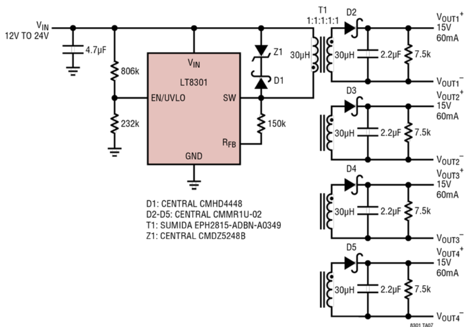
12V 至 24V_{IN} /四路 15V_{OUT} 微功耗隔离型反激式转换器
