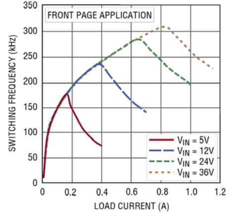
开关频率与负载电流的关系
