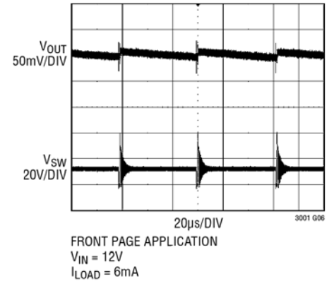
突发模式波形
