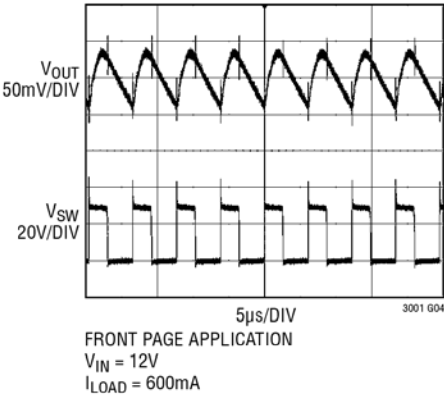
临界模式波形
