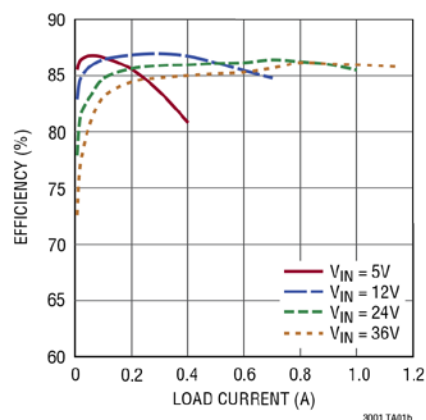
效率与负载电流的关系
