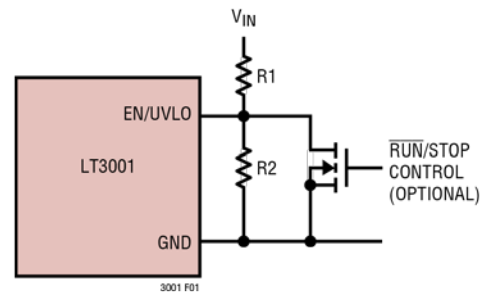
图 1. 欠压闭锁 (UVLO)
