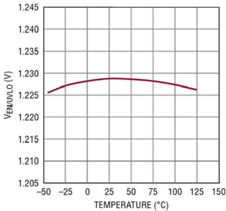
EN/UVLO 使能阈值
