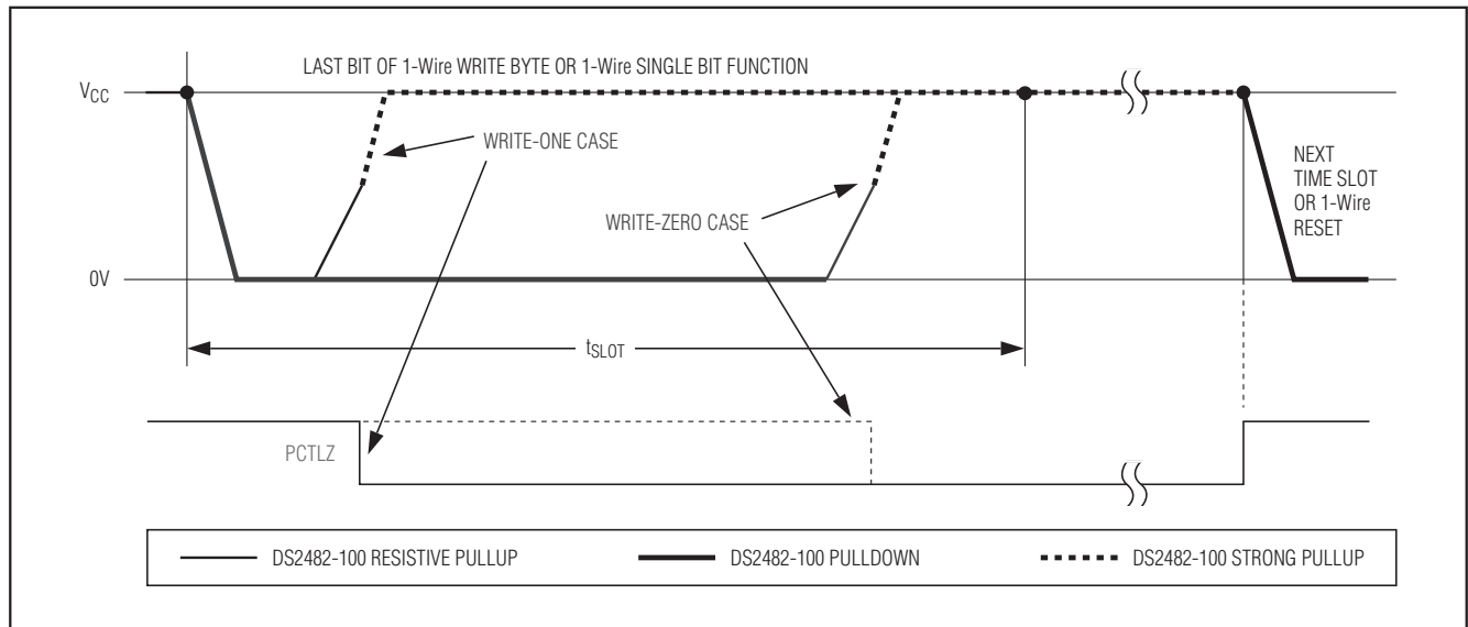
图3. 低电阻上拉时序
