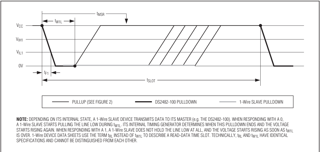
图6. 写1和读数据时隙
