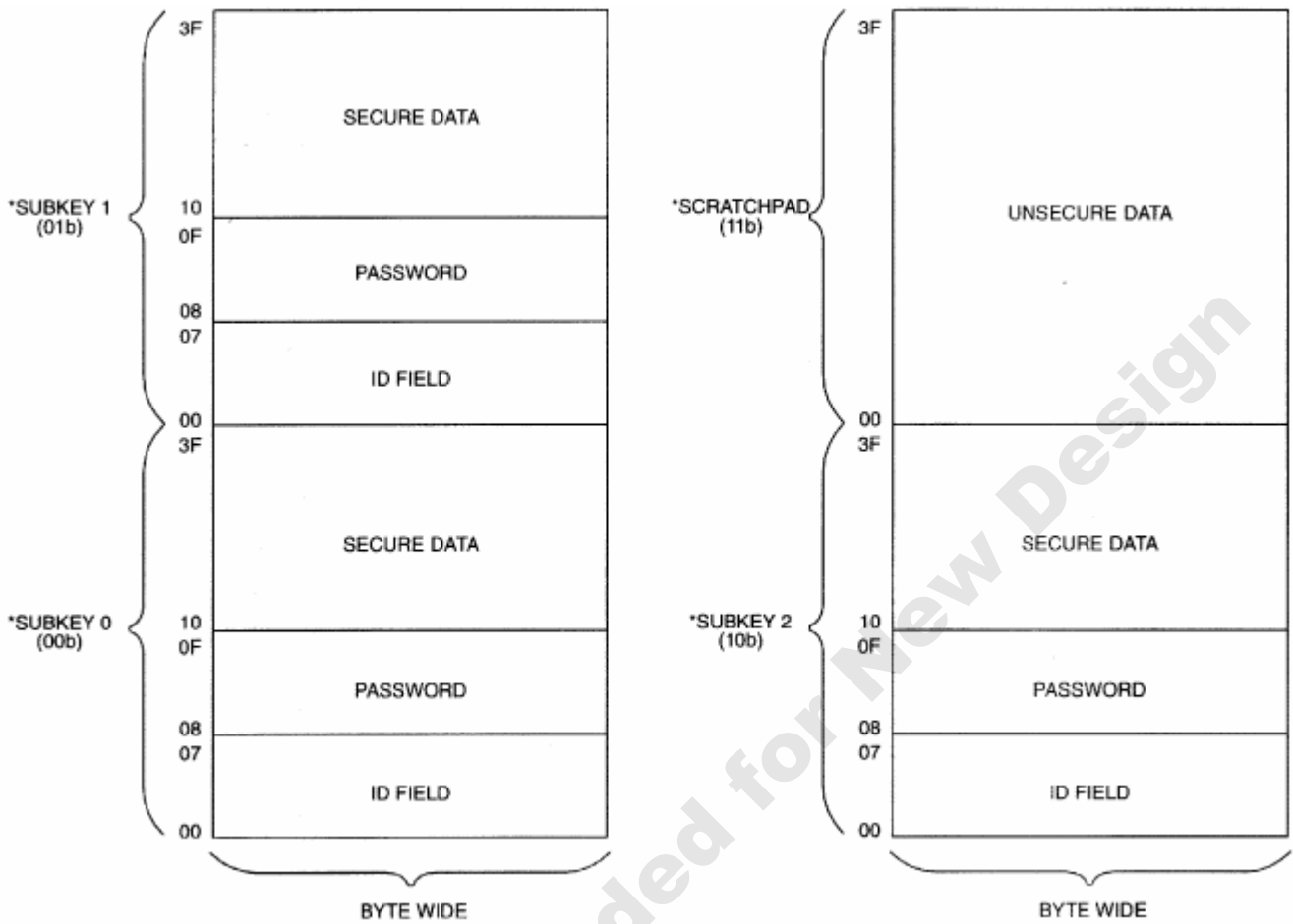
存储器图 图 1
