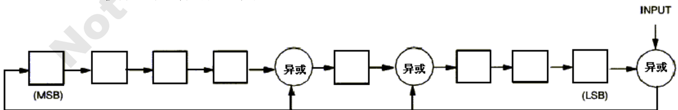
1-Wire CRC 校验码生成器 图 3
