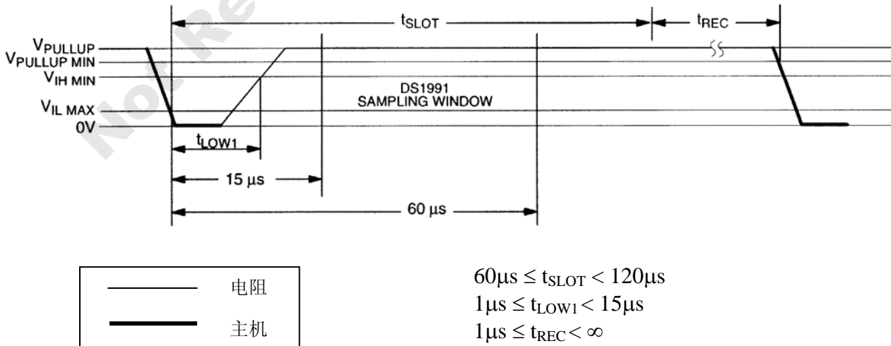
读 / 写时隙图 图 11 写 1 (Write 1) 时隙
