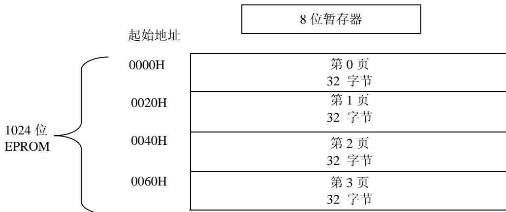
DS1982 存储器结构分配图 图 5
