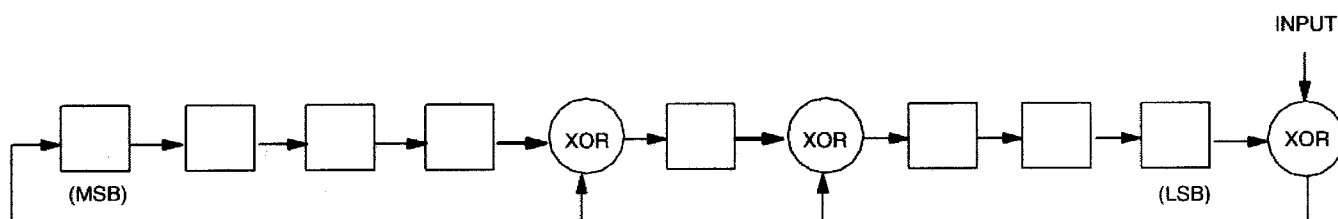
1-Wire CRC 校验码生成器 图 4
