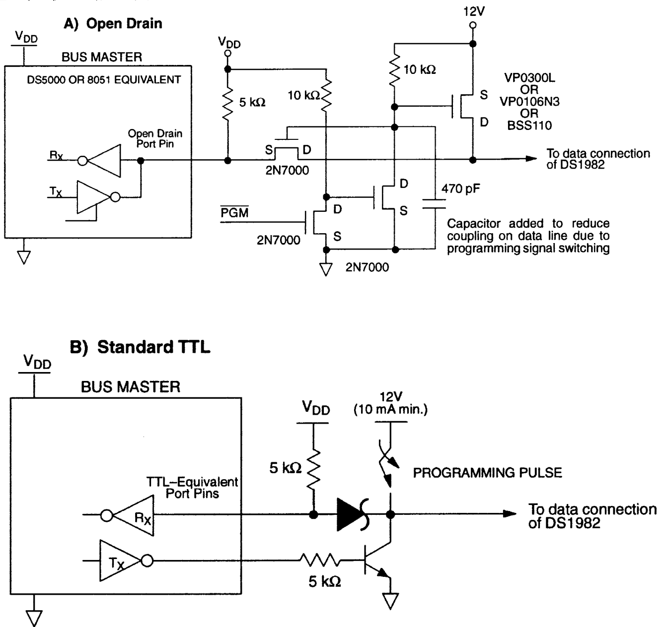
总线主机电路 图 8
