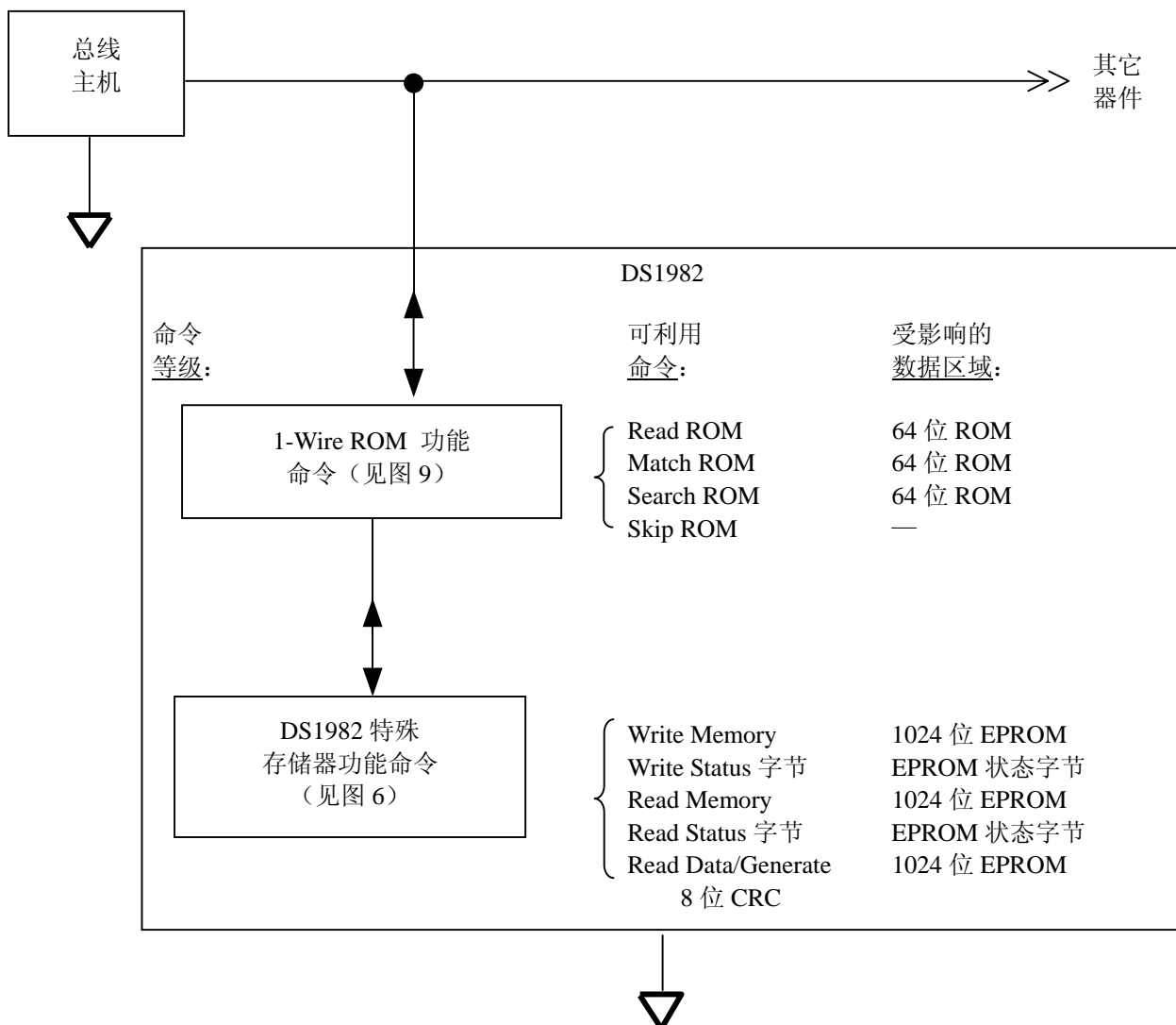
1-Wire 协议的层次结构图 图 2
