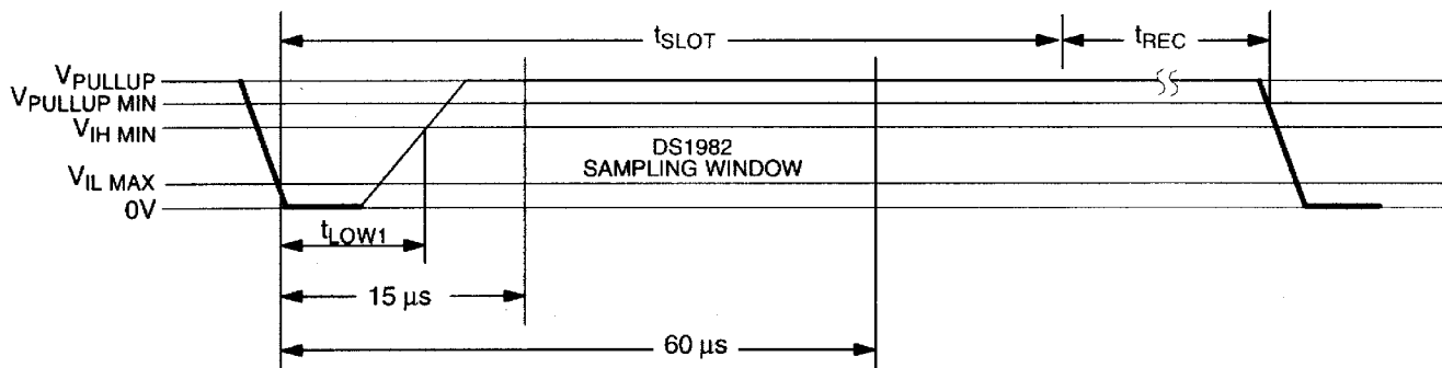
读/写时序图 图 11 写 1 时隙
