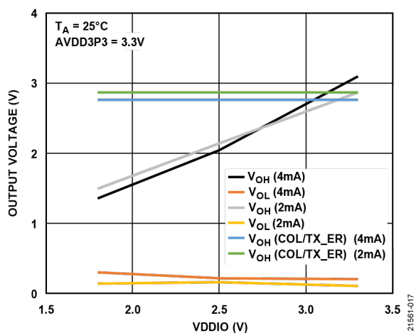
图18. 数字输出三电平与VDDIO的关系
