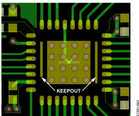
图38. EVAL-ADIN1200FMCZ上的裸露焊盘通过阵列
