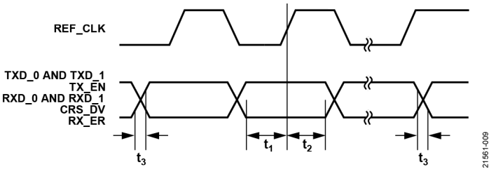
图9. RMII时序
