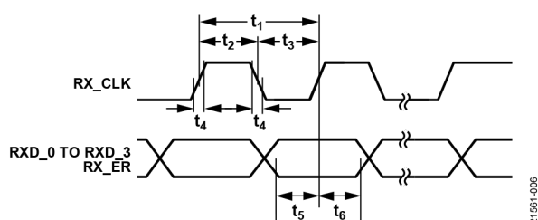
图6. MII接收时序
