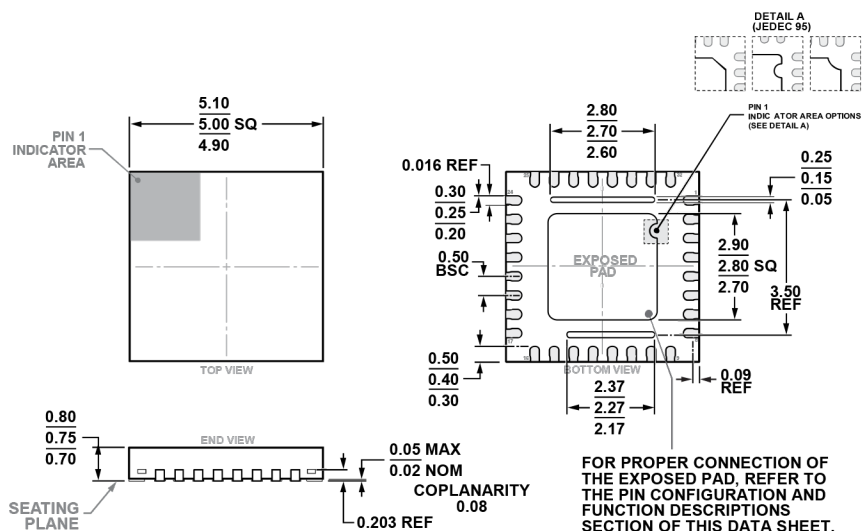
图40. 32引脚引线框芯片级封装[LFCSP]
