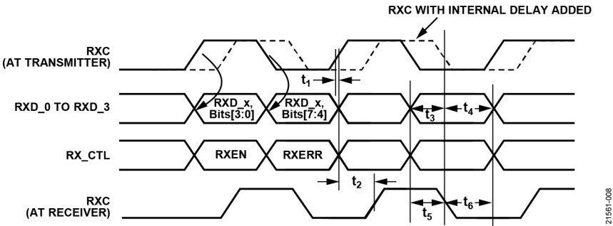
图8. RGMII接收时序
