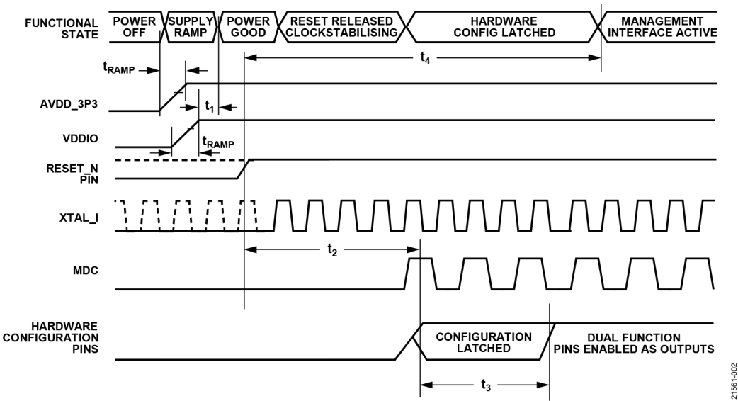
图2. 上电时序
