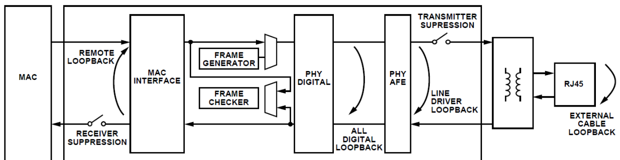
图28. 环回模式
