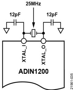
图32. 晶体振荡器连接
