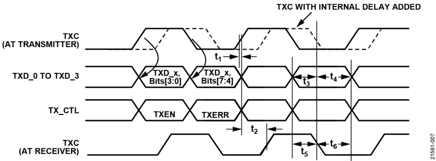
图7. RGMII发送时序
