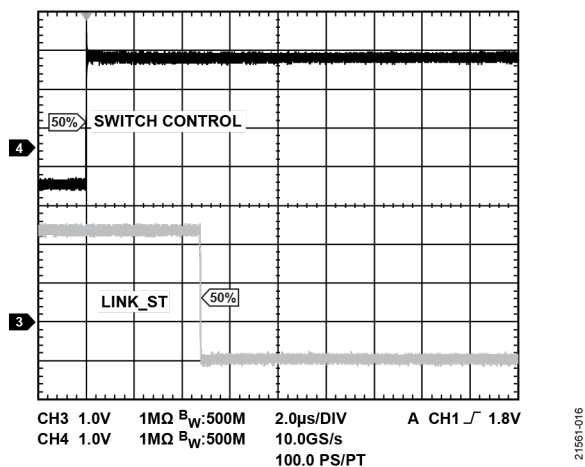
图17. 增强型链路检测100 Mbps、100 m电缆，单线断开
