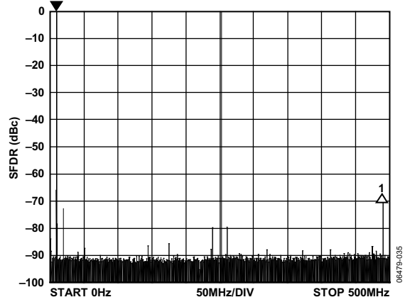
图9. 10 MHz条件下的宽带SFDR, REFCLK = 1 GHz
