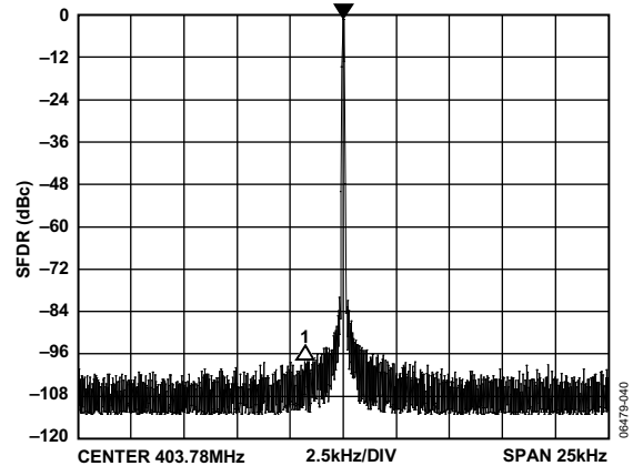
图14. 403.78 MHz条件下的窄带SFDR, REFCLK = 1 GHz
