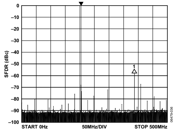
图10. 204 MHz条件下的宽带SFDR, REFCLK = 1 GHz
