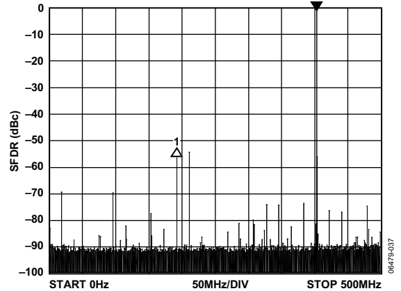
图11. 403 MHz条件下的宽带SFDR, REFCLK = 1 GHz
