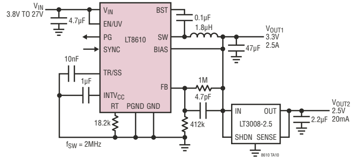
具 LDO 的超低 I_Q 2.5V、3.3V 降压
