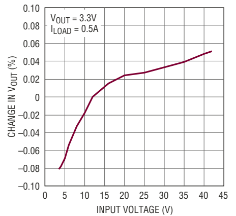
电压调节
