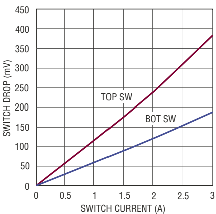
开关压降
