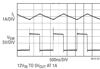
开关波形
