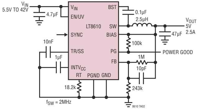
5V 降压型转换器
