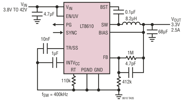
3.3V 降压型转换器
