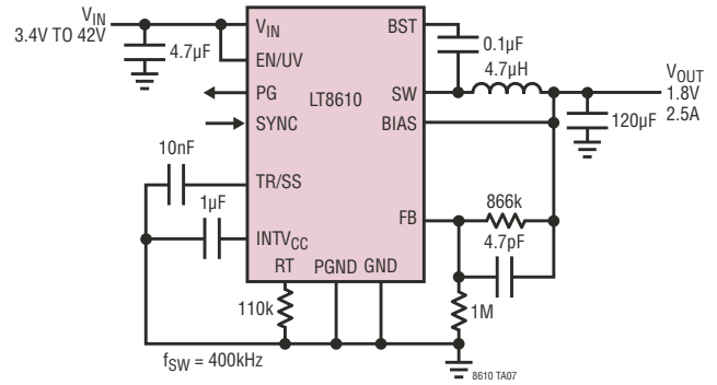
1.8V 降压型转换器
