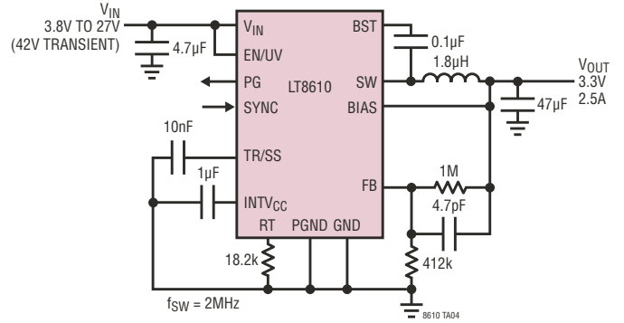
3.3V 降压型转换器
