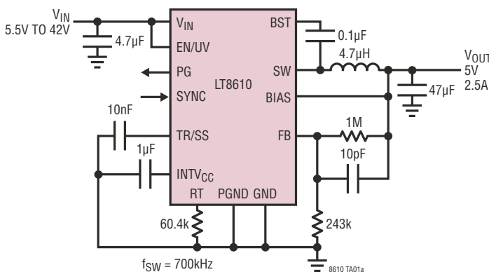
5V、2.5A 降压型转换器
