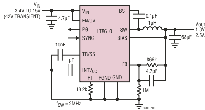
1.8V 2MHz 降压型转换器
