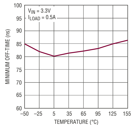
最小断开时间
