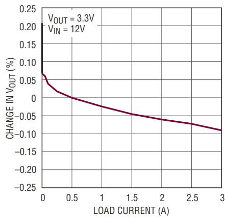
负载调节
