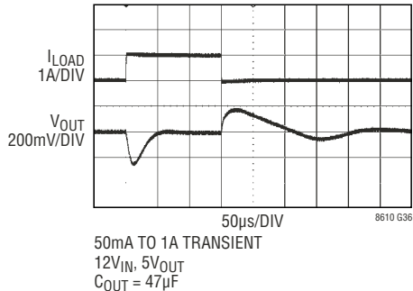
瞬态响应
