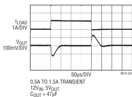
瞬态响应
