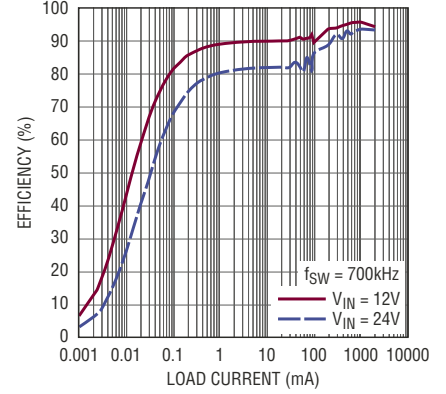
在 5V OUT 时的效率
