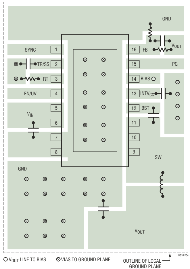
图 4：针对 LT8610 的推荐 PCB 布局
