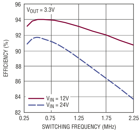
效率与频率的关系
