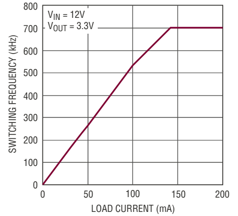
突发频率
