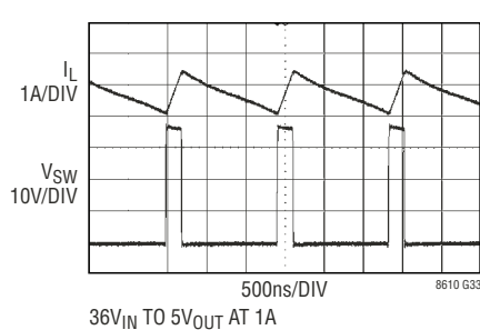
开关波形
