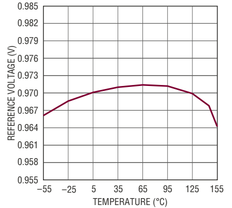
基准电压
