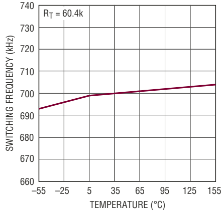
开关频率
