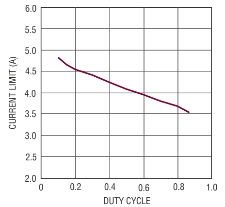
顶端 FET 电流限值与占空比的关系
