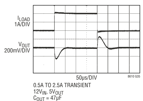
瞬态响应
