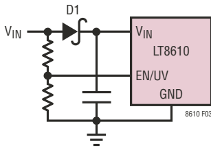
图 3：反向 V_{IN} 保护
