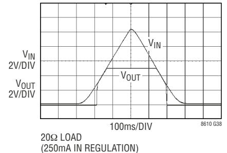
启动压差性能
