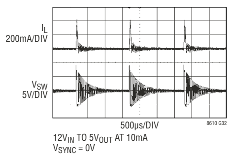
开关波形
