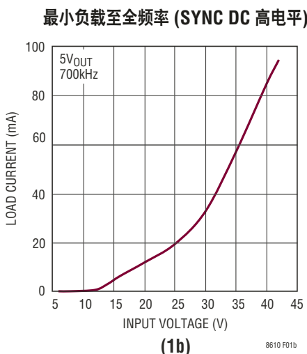
图 1 : SW 频率与负载信息的关系 (1a) 突发模式操作中 (1b) 脉冲跳跃模式中
