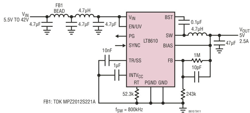
超低 EMI 5V 2.5A 降压型转换器
