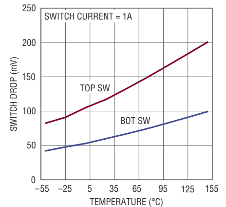
开关压降
