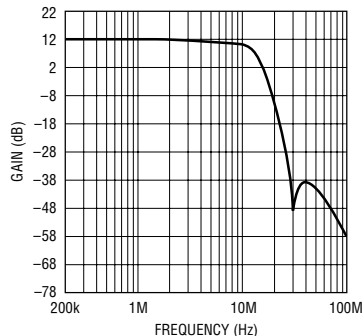
幅度响应
