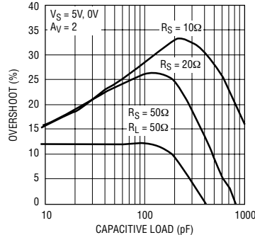
串联输出电阻与容性负载的关系曲线
