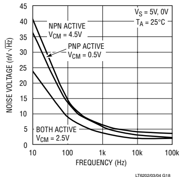
输入噪声电压与频率的关系
