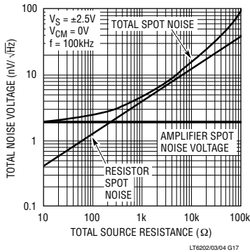
总噪声与总源电阻的关系
