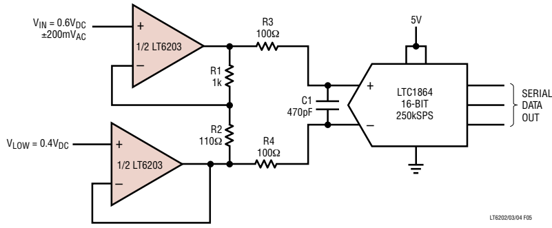
图 5：单电源 16 位 ADC 驱动器
