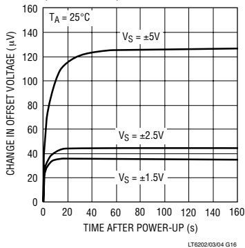
温升漂移与时间的关系曲线 (LT6203S8)
