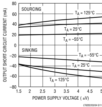
输出短路电流与电源电压的关系曲线
