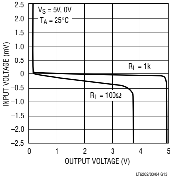
开环增益
