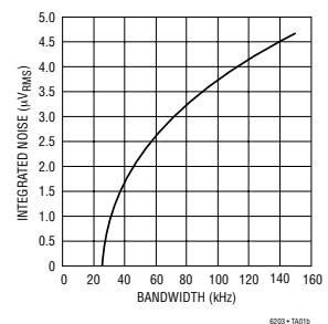
线路接收器积分噪声 (25kHz 至 150kHz)
