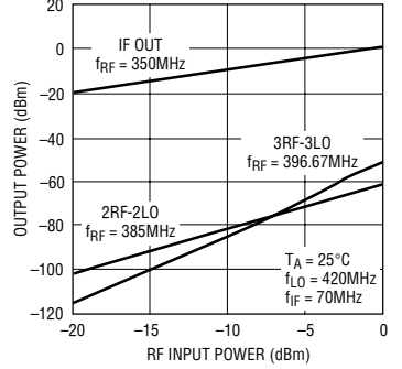
IF OUT 、2×2 和 3×3 寄生噪声与 RF 输入功率的关系
