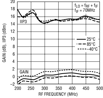
转换增益和 IIP3 与 RF 频率的关系曲线
