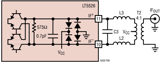
图 9：采用外部匹配的 IF 输出
