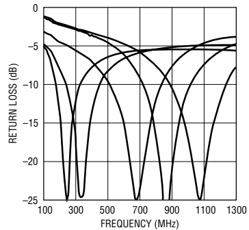
图 6：采用集总元件平衡-不平衡转换器 (元件值取自表 2) 时的输入回程损耗
