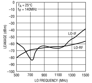
LO-IF 和 LO-RF 泄漏与 LO 输入频率的关系曲线
