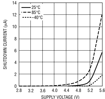
停机电流与电源电压的关系
