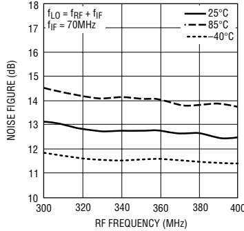
SSB 噪声指数与 RF 频率的关系曲线
