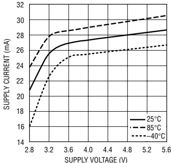
电源电流与电源电压的关系
