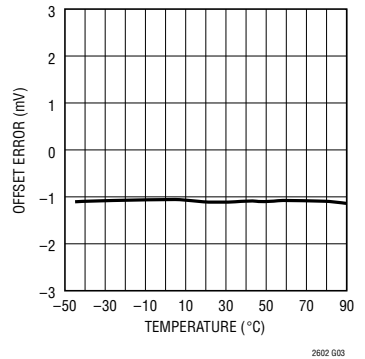
偏移误差与温度的关系曲线
