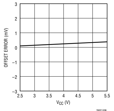
偏移误差与 VCC 的关系曲线
