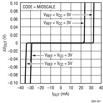
电流限值
