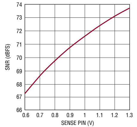
LTC2175-14 : SNR 与 SENSE 的关系曲线, f_{IN} = 5\text{MHz} , -1dB
