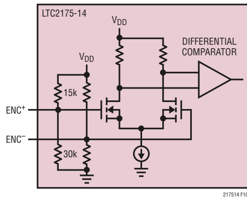
图 10：用于差分编码模式的等效编码输入电路
