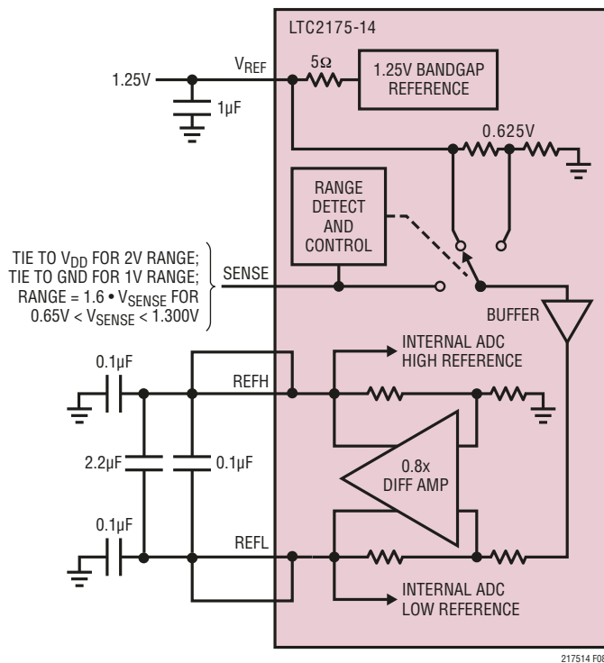
图 8：基准电路
