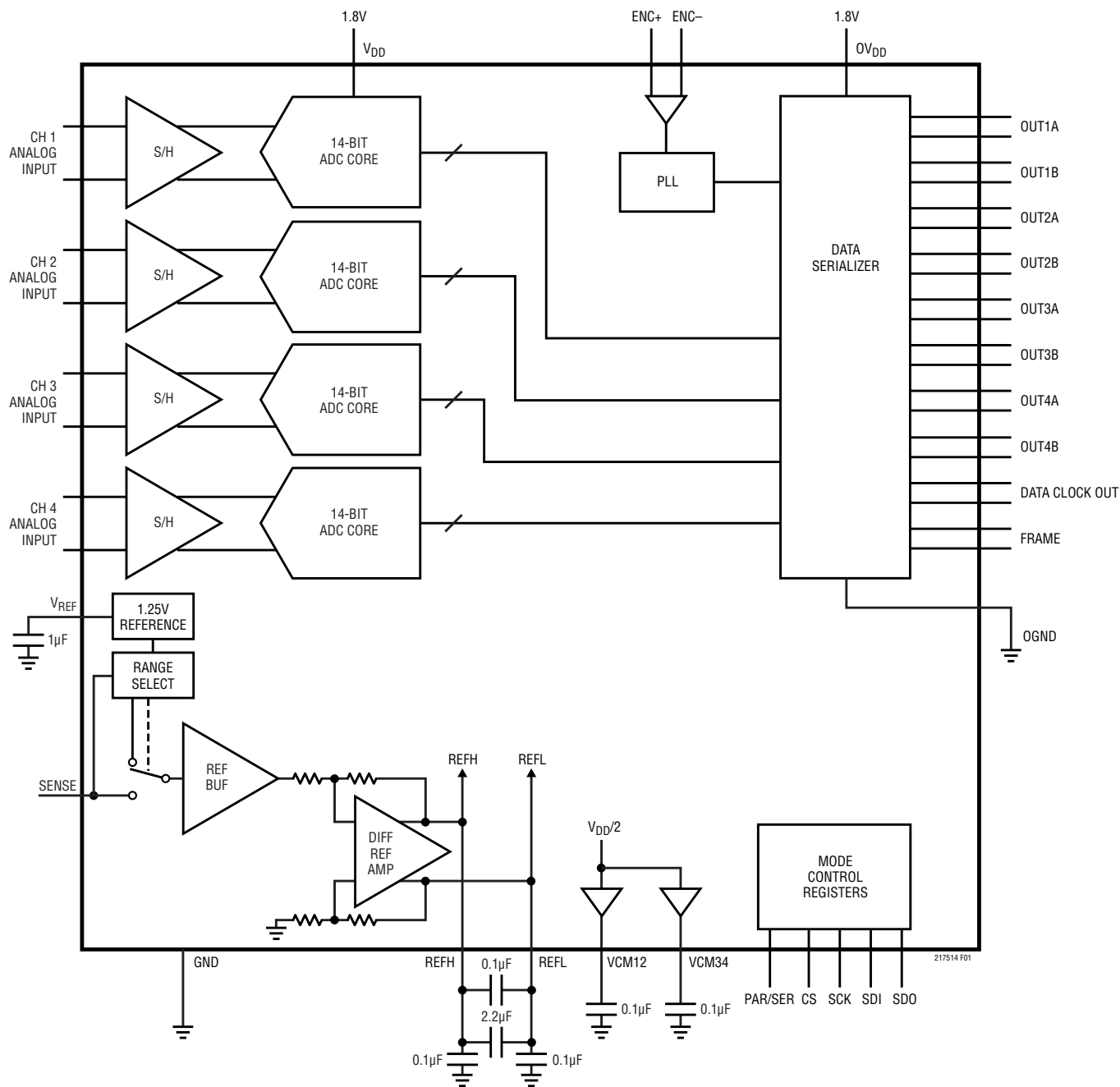
图 1：功能方框图
