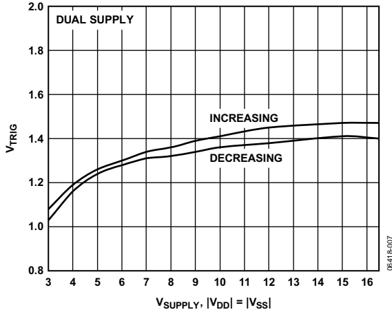
图7 触发电平与双电源电压的函数关系曲线
