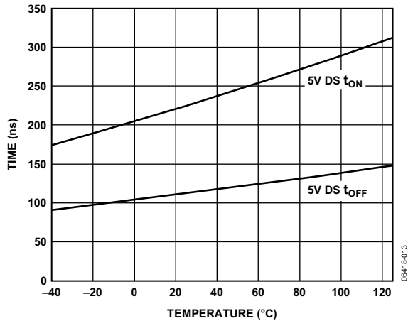
图16 5 V双电源电压下 t_{ON}/t_{OFF} 与温度的关系曲线
