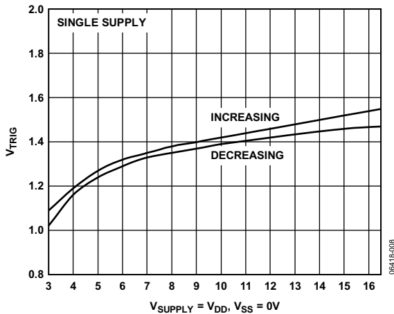
图8 触发电平与单电源电压的函数关系曲线
