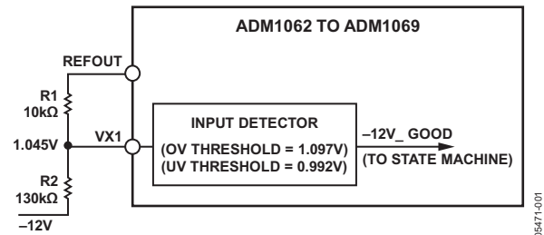
图 1. 通过电阻分压器监控 VX1 引脚上的 -12 V 电源
