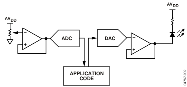
图2. RTD电路图
