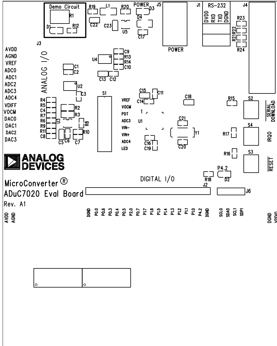
图4. 评估板丝网图
