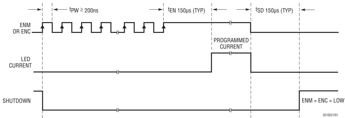
図1. 電流プログラミングのタイミング図
