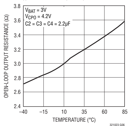
1.5倍モードのチャージポンプの 開ループ出力抵抗と温度 ( (1.5V_{BAT} - V_{CPO})/I_{CPO} )
