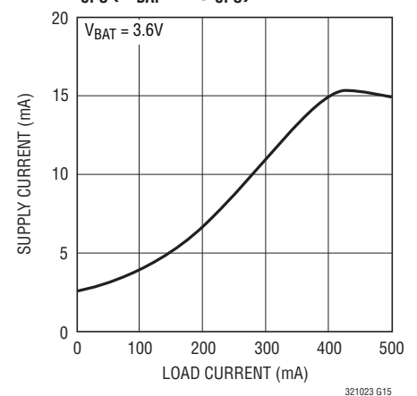
1.5倍モードの消費電流と I_{CP0} ( I_{VBAT} = 1.5I_{CP0} )
