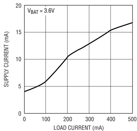
2倍モードの消費電流と I_{CP0} ( I_{VBAT} = 2I_{CP0} )
