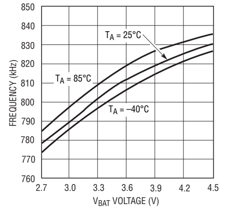
発振器周波数と V_{BAT} の電圧
