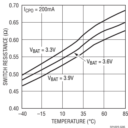
1倍モードのスイッチ抵抗と温度
