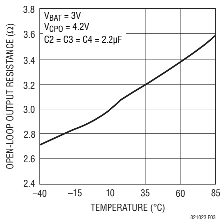
図3. 1.5倍モードの標準的 R_{OL} と温度
