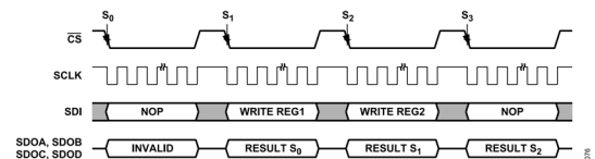
図 77. レジスタの書込み
