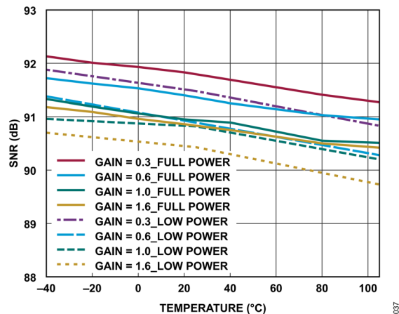
図 37. S/N 比と温度の関係、 f_{IN} = 1\text{kHz}
