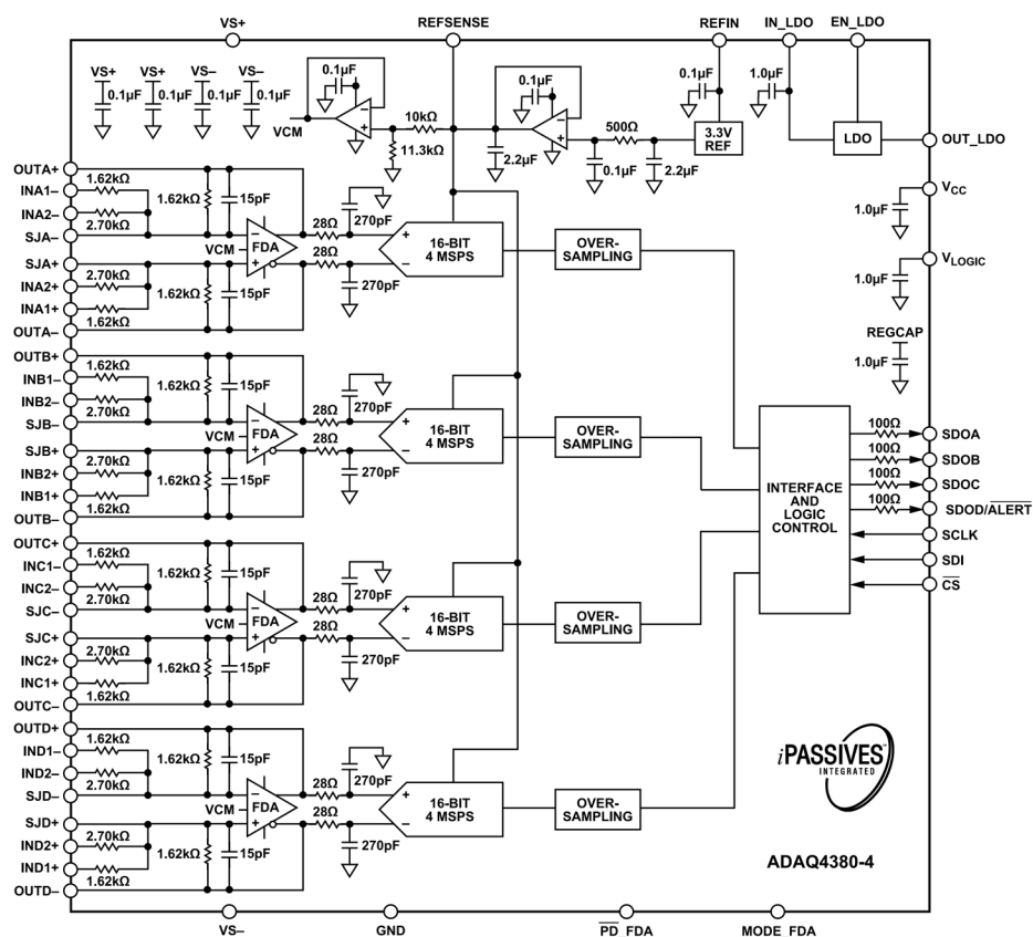
図 46. ADAQ4380-4 μModule の簡略ブロック図
