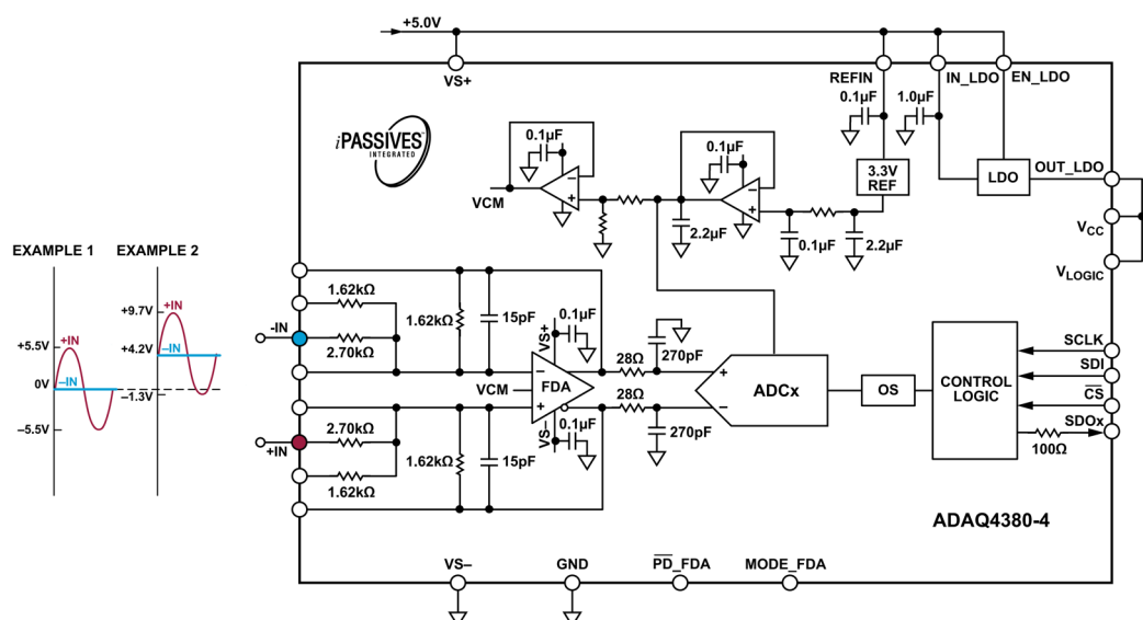
図 53. シングルエンド入力構成、ゲイン = 0.6、 \pm 5.5\text{V} 入力、 V_S = 5\text{V}
