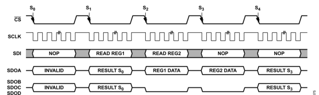
図 76. レジスタ読出し
