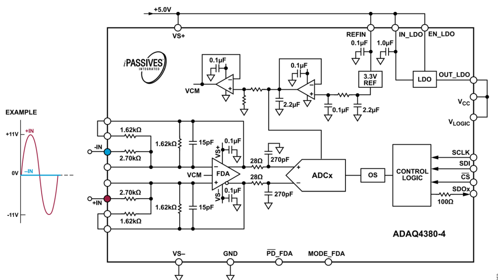
図 52. シングルエンド入力構成、ゲイン = 0.3、 \pm 11\text{V} 入力、 V_S = 5\text{V}
