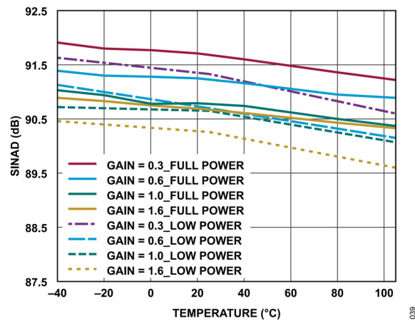
図 39. SINAD と温度の関係、 f_{IN} = 1\text{kHz}
