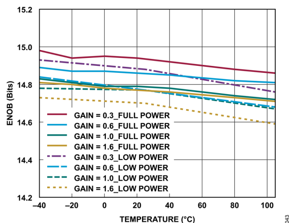
図 43. ENOB と温度の関係、 f_{IN} = 1\text{kHz}
