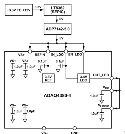
図 65. ADAQ4380-4 の電源に関する推奨
