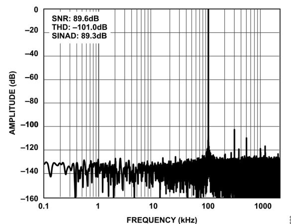
図 33. 100kHz、-0.5dBFS 入力トーン FFT、 ゲイン = 1.6、差動入力、低消費電力モード
