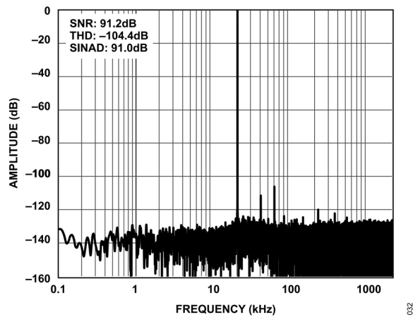
図 32. 20kHz、-0.5dBFS 入力トーン FFT、 ゲイン = 1.0、シングルエンド入力、通常消費電力モード
