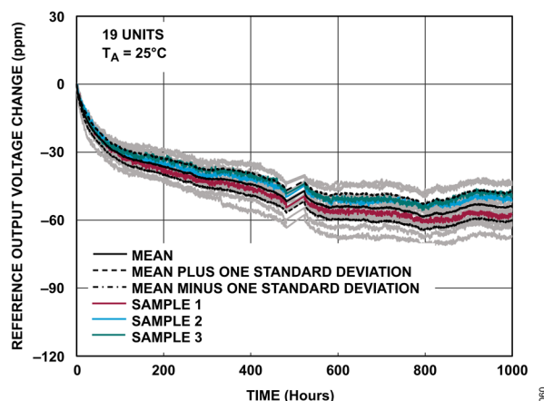
図 61. ADAQ4380-4 内部リファレンスの長期ドリフト
