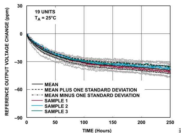
図 62. ADAQ4380-4 内部リファレンスの初期ドリフト
