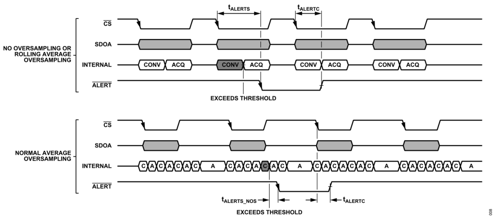
図 8. \overline{ALERT} のタイミング
