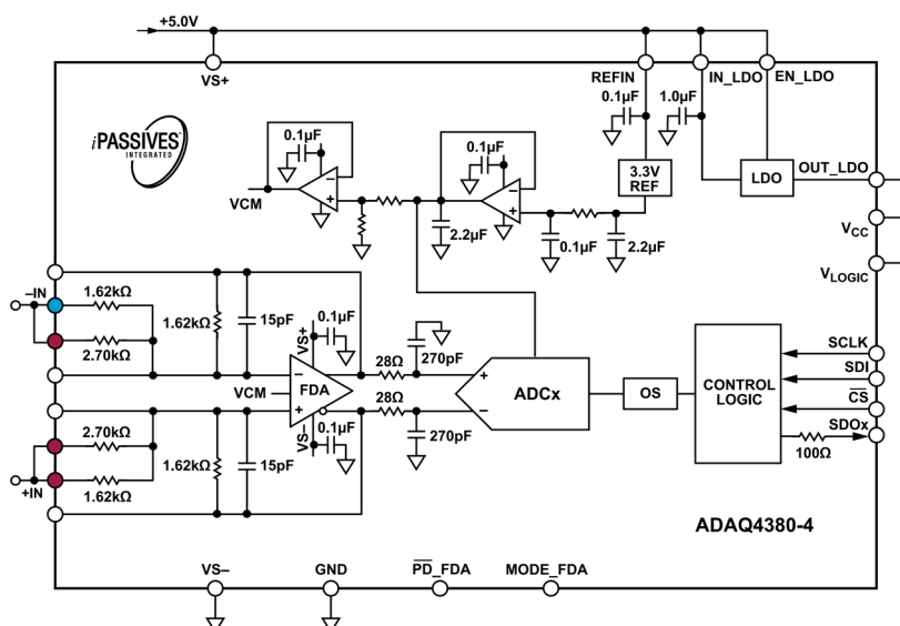
図 55. シングルエンド入力構成、ゲイン = 1.6、 \pm 2.06\text{V} 入力、 V_S = 5\text{V}
