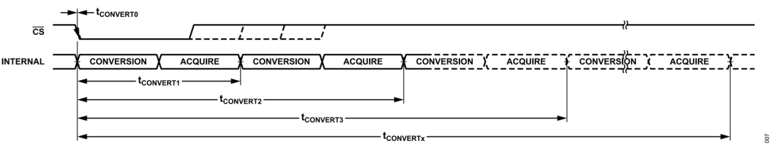
図 7. OS ノーマル・モードでの変換タイミング
