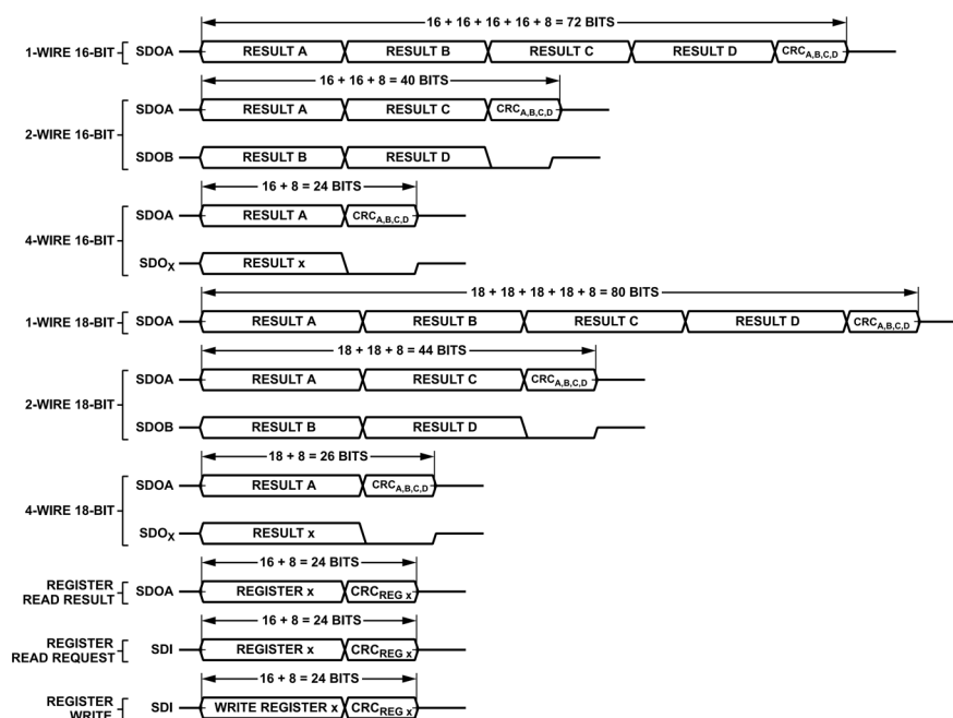
図 78. CRC の動作
