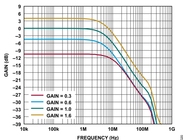
図 20. ADC ドライバのクロードループ・ゲインと周波数の関係
