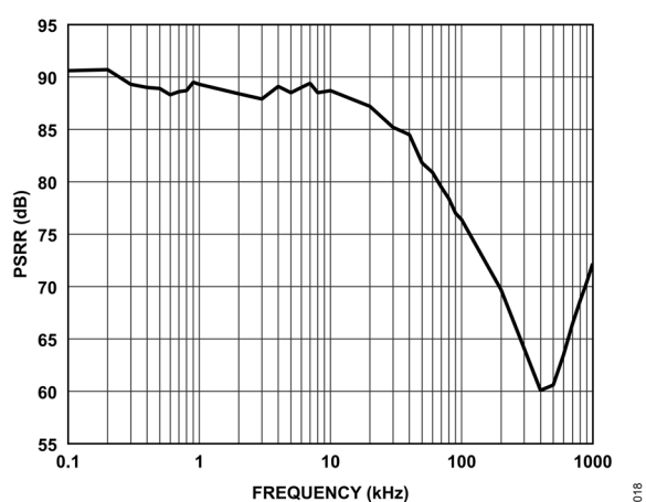
図 18. PSRR と周波数の関係
