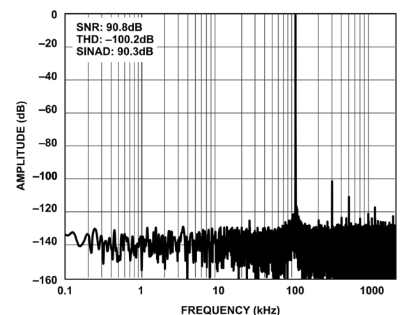
図 27. 100kHz、-0.5dBFS 入力トーン FFT、 ゲイン = 0.3、差動入力、通常消費電力モード
