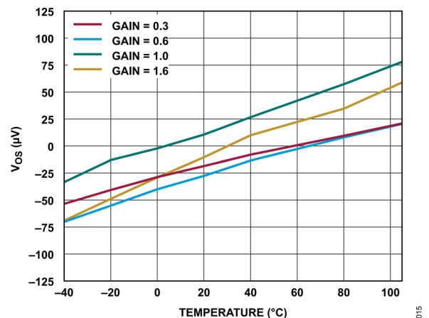
図 15. オフセット誤差と温度の関係
