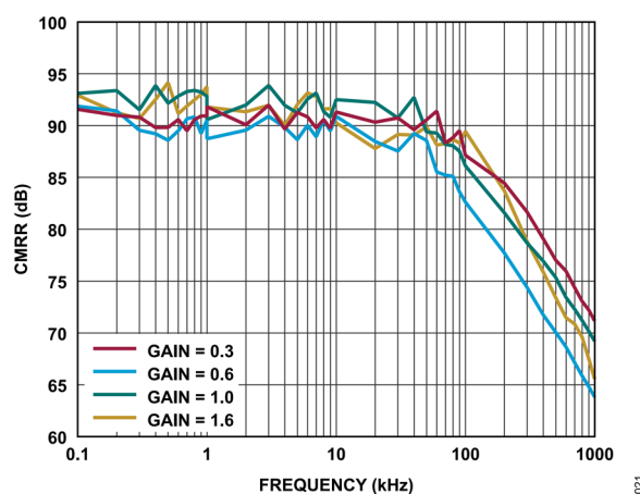
図 21. CMRR と周波数の関係
