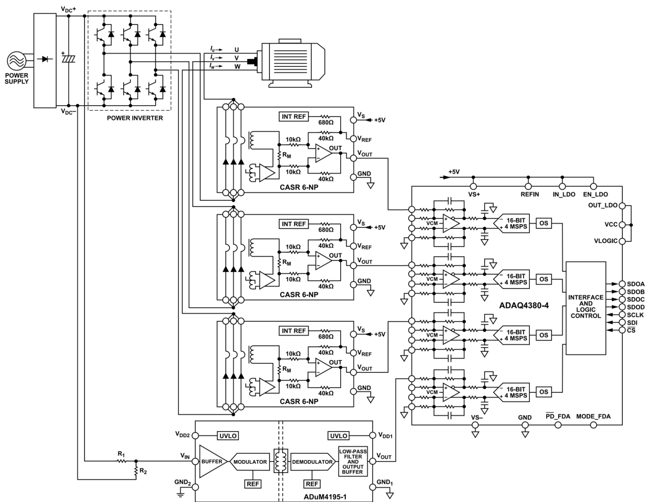
図 1. サーボモータ制御のための高精度電流および電圧センシング
