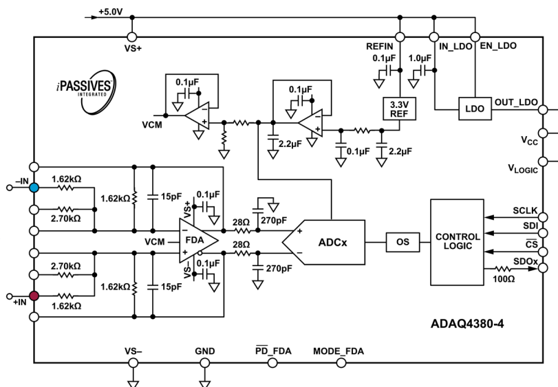
図 54. シングルエンド入力構成、ゲイン = 1.0、 \pm 3.3\text{V} 入力、 V_S = 5\text{V}
