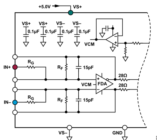
図 58. ADAQ4380-4 の完全差動入力構成
