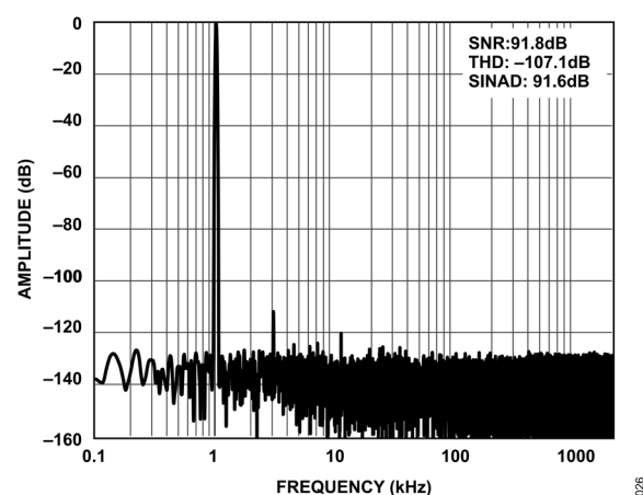
図 26. 1kHz、-0.5dBFS 入力トーン FFT、 ゲイン = 0.3、シングルエンド入力、フルパワー動作モード
