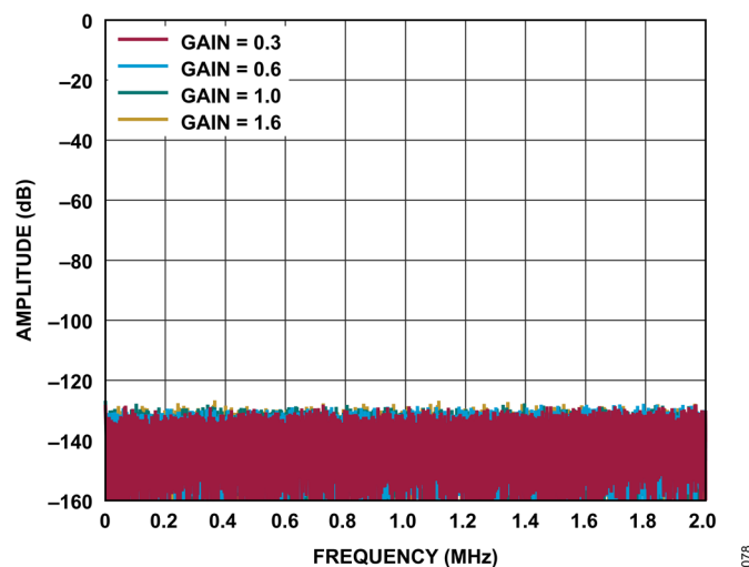
図 79. 入力を短絡したときの FFT
