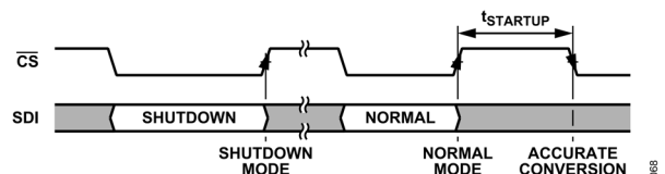
図 69. シャットダウン・モード動作
