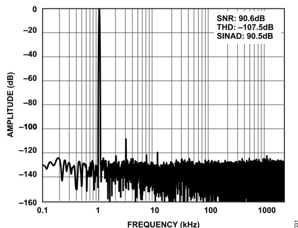
図 31. 1kHz、-0.5dBFS 入力トーン FFT、 ゲイン = 0.6、シングルエンド入力、ローパワー動作モード
