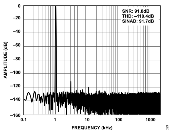
図 23. 1kHz、-0.5dBFS 入力トーン FFT、 ゲイン = 0.3、差動入力、フルパワー動作モード
