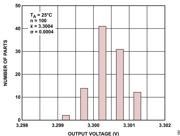
図 60. ADAQ4380-4 の内部リファレンス出力電圧の精度
