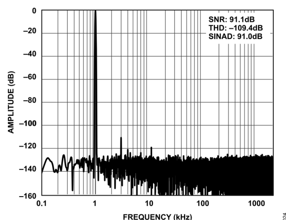
図 24. 1kHz、-0.5dBFS 入力トーン FFT、 ゲイン = 0.3、差動入力、ローパワー動作モード
