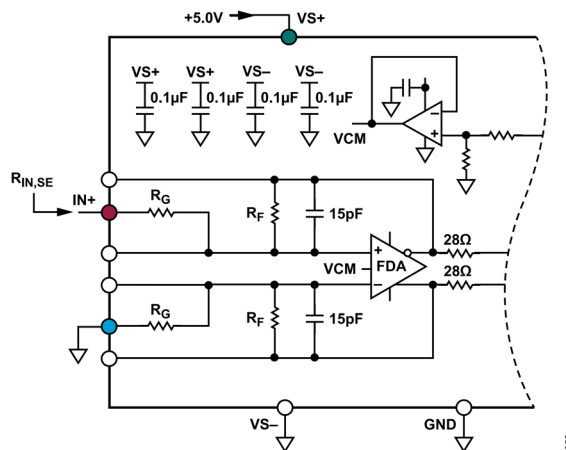
図 59. ADAQ4380-4 のシングルエンド入力構成
