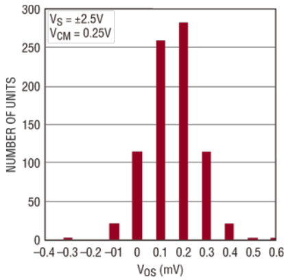
输入失调电压分布
