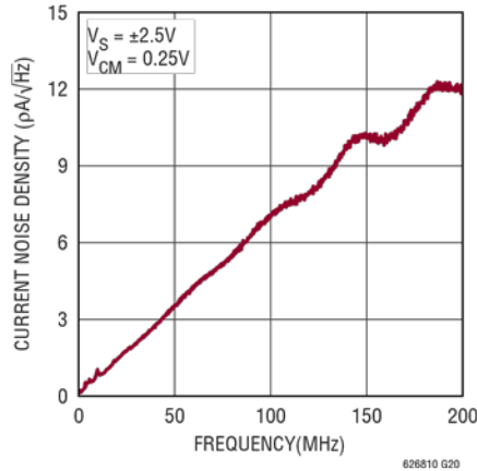
折合到输入端的电流噪声
