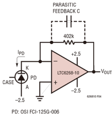
图 4. LTC6268-10 和 402k \Omega TIA 中的低电容光电二极管
