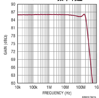
20k \Omega TIA 频率响应
