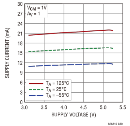
电源电流与电源电压的关系
