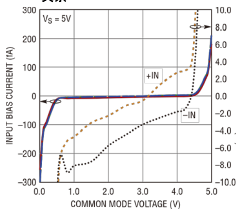
输入偏置电流与共模电压的关系
