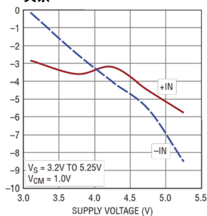
输入偏置电流与电源电压的关系
