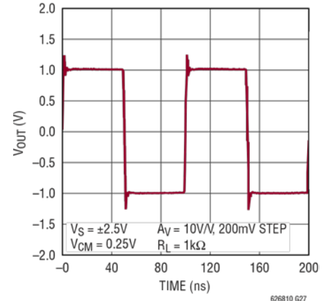
大信号阶跃响应
