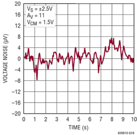
折合到输入端的 0.1Hz 至 10Hz 电压噪声
