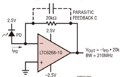
20k \Omega 增益 210MHz 跨阻放大器
