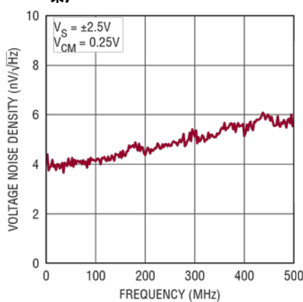
折合到输入端的宽带电压噪声
