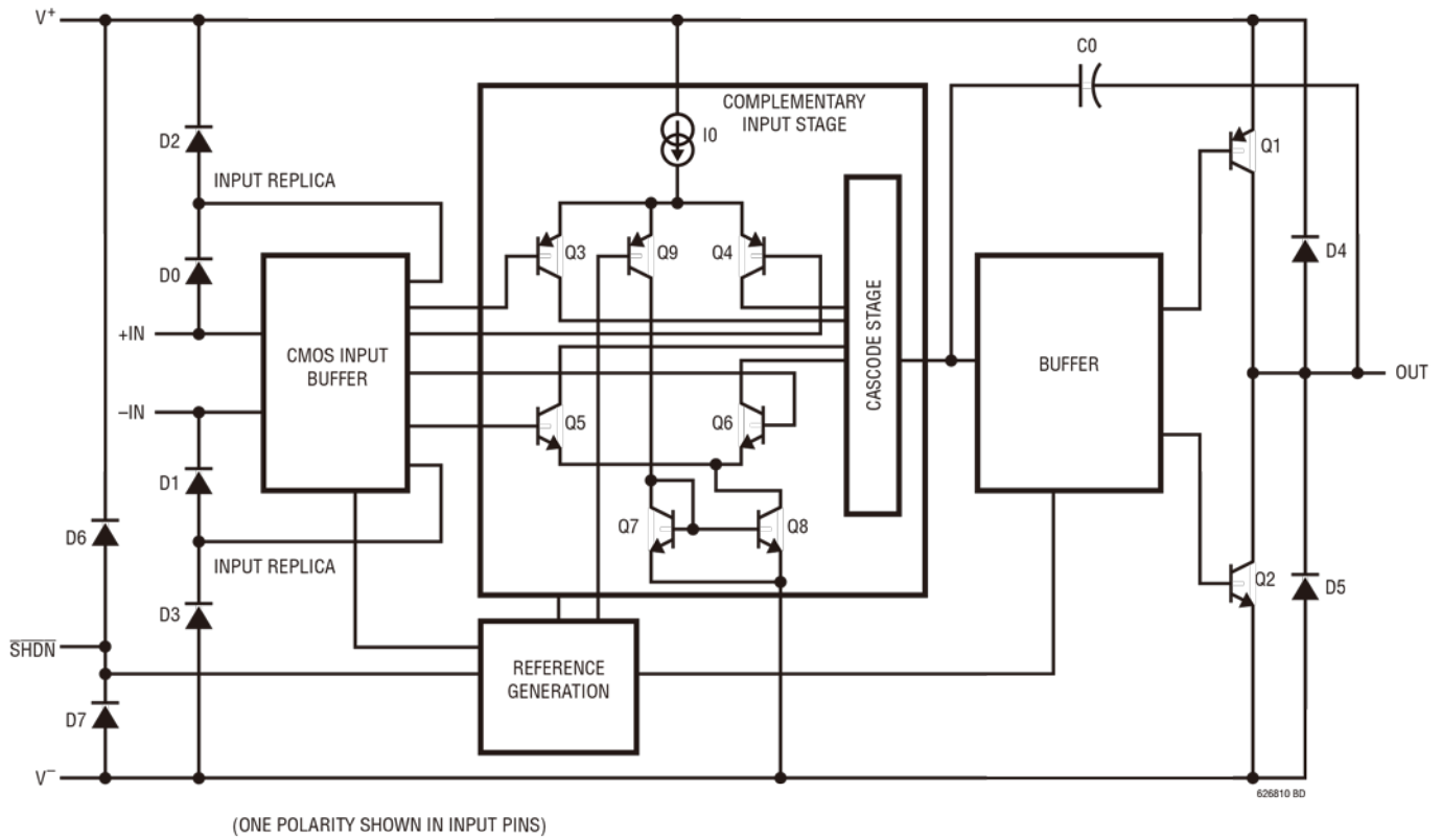
LTC6268-10 原理示意图
