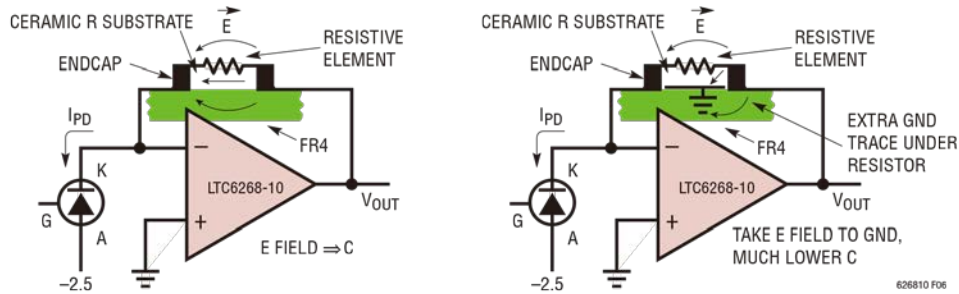
图 6. 左侧是标准布局，右侧是场分流布局。仅仅在反馈电阻下方添加一条接地走线，便可将电场从反馈侧分流，并将其注入接地。请注意，FR4 和陶瓷的介电常数典型值 4，因此大部分电容位于固体中，而不是空气引起的。反馈电容 C 从左侧的 100fF 降低至右侧的 11.6fF
