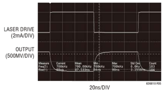
图 5. 402k \Omega TIA 的时域响应，没有付出额外的努力来降低反馈电容。上升时间为 87ns，带宽为 4MHz
