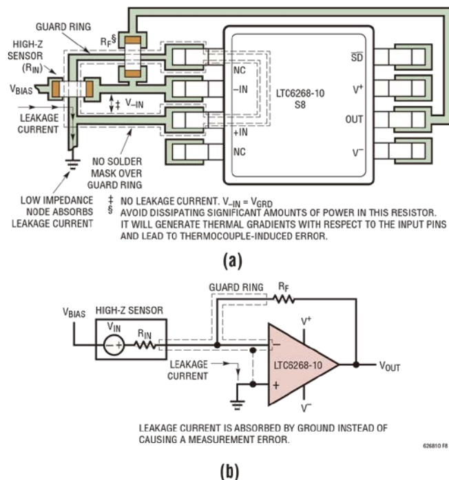
图 8. 带漏电保护环的反相放大器 (或跨阻) 的布局示例
