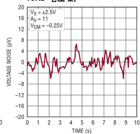
折合到输入端的 0.1Hz 至 10Hz 电压噪声
