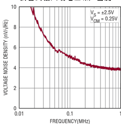
折合到输入端电压噪声密度
