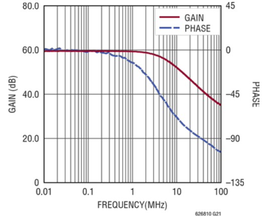
增益/相位与频率的关系
