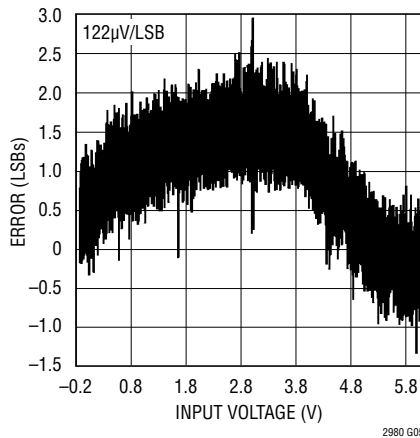
ADC INL
