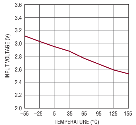
V_{IN} UVLO
