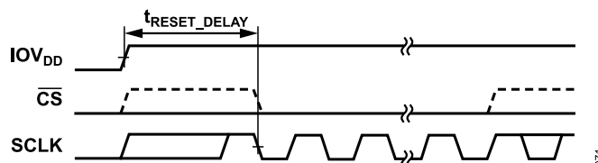
Figure 72. POR Timing Diagram
