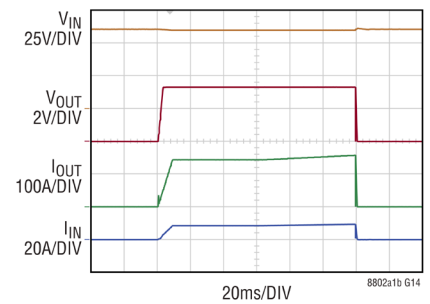
60V IN 時の過電流保護
