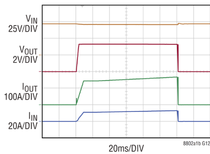
45V IN 時の過電流保護
