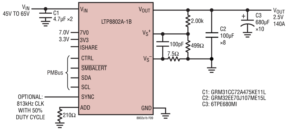
図9. PMBusを使用した2.5V 140A 813kHz 降圧モジュール
