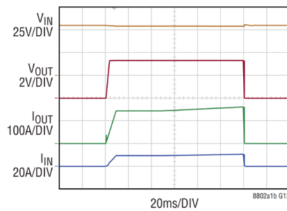
54V IN 時の過電流保護
