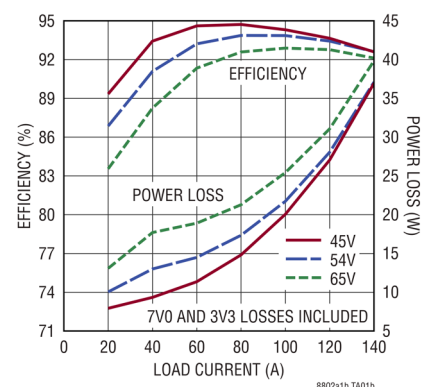
3.3V OUT における効率と電力損失
