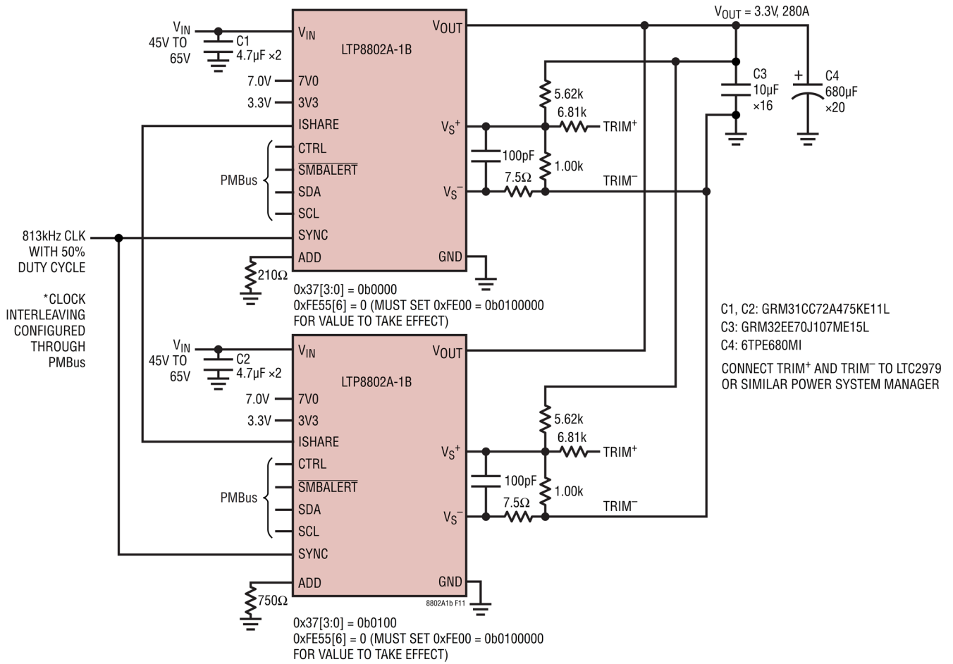
図 11. パワー・システム・マネージメント機能付きの 3.3V/280A を生成する 2 相動作
