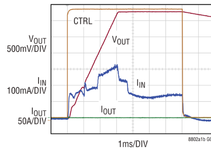
無負荷時のスタートアップと シャットダウン、CTRLによりトリガ
