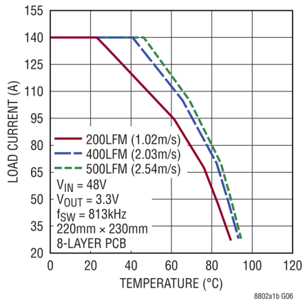
図6. 温度ディレーティング、 48VIN、3.3VOUT、813kHz
