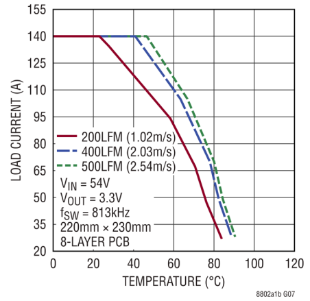
図7. 温度ディレーティング、 54VIN、3.3VOUT、813kHz
