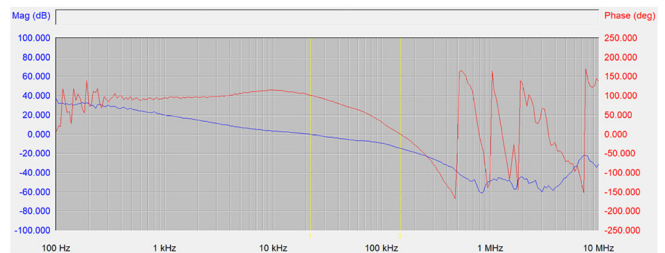
図3. 補償のポールとゼロの調整
