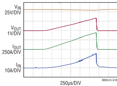
54V IN 、出力短絡時のスタートアップ
