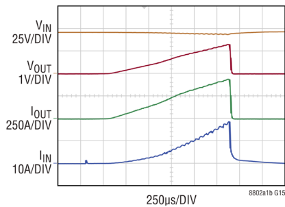
45V IN 、出力短絡時のスタートアップ
