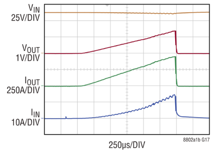
60V IN 、出力短絡時のスタートアップ
