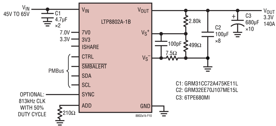
図 10. PMBus を使用した 3.3V 140A 813kHz 降圧モジュール
