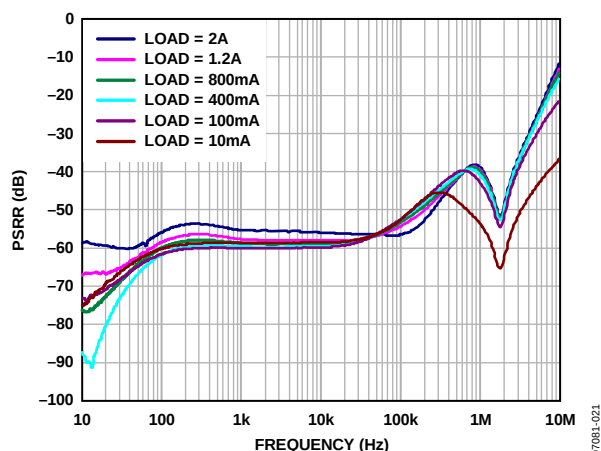
图21. 电源抑制比与频率的关系( V_{OUT} = 1.5 V , V_{IN} = 2.5 V )
