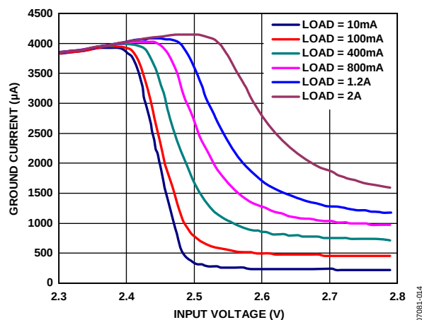
图14. 低压差下接地电流与输入电压的关系( V_{\text{OUT}} = 2.5\text{ V} )
