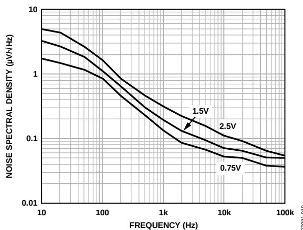
图19. 噪声谱密度与输出电压的关系( I_{LOAD} = 10 mA )
