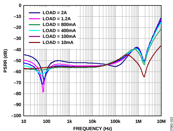
图22. 电源抑制比与频率的关系( V_{OUT} = 2.5 V , V_{IN} = 3.5 V )
