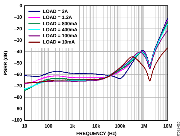
图20. 电源抑制比与频率的关系( V_{OUT} = 0.75 V , V_{IN} = 1.75 V )
