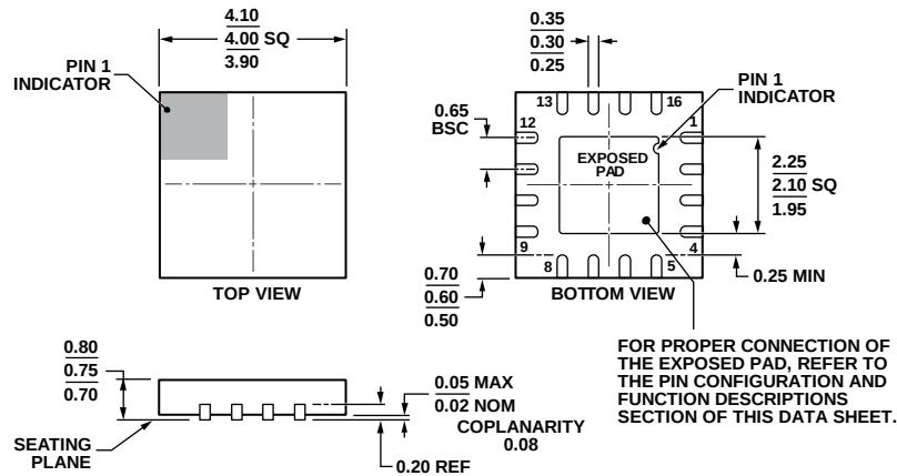
图49. 16引脚引脚架构芯片级封装[LFCSP_WQ] 4 mm × 4 mm, 超薄体 (CP-16-23) 图示尺寸单位: mm
