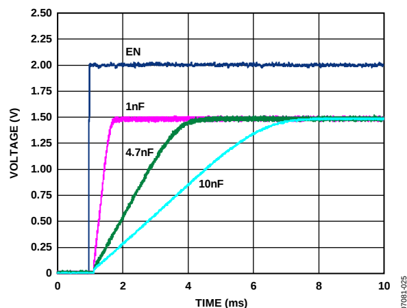
图26. 使用外部软启动电容的V OUT 上斜坡
