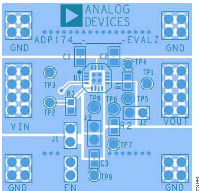
图47. 典型评估板布局布线——顶端
