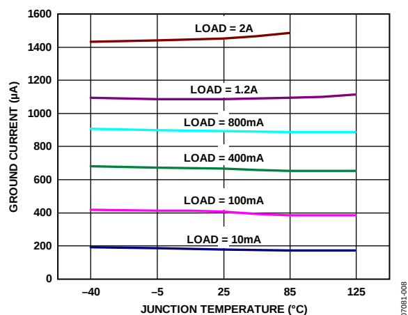
图8. 地电流与结温的关系
