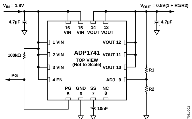
图2. 提供0.75 V至3.3 V可调输出电压的ADP1741
