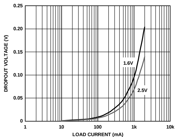
图12. 压差与负载电流的关系( V_{\text{OUT}} = 1.6\text{ V} 、 2.5\text{ V} )
