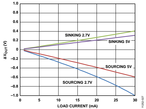
图26. 上裕量/下裕量与负载电流的关系
