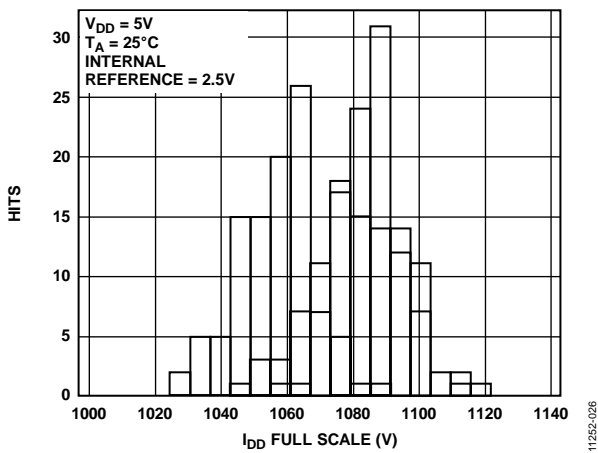
图25. 采用内部基准电压源时的 I_{DD} 直方图 ( V_{REFOUT} = 2.5V , 增益 = 2)
