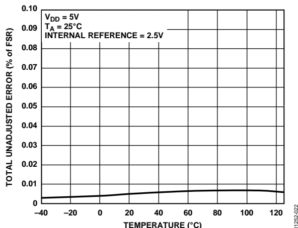
图21. 总不可调整误差与温度的关系
