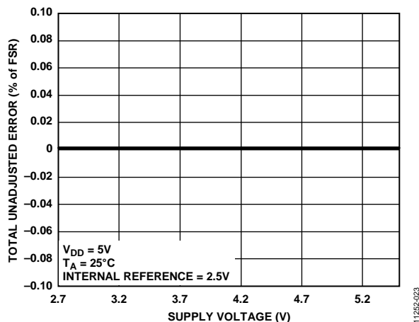
图22. 总不可调整误差与电源电压的关系, 增益 = 1
