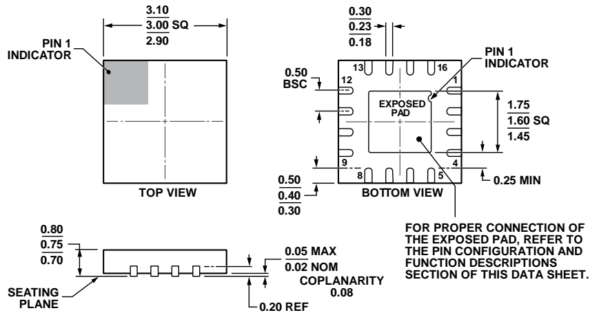
图54. 16引脚脚架构芯片级封装[LFCSP_WQ] 3 mm x 3 mm, 超薄体 (CP-16-22) 尺寸单位: mm
