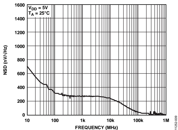
图8. 内部基准电压噪声谱密度与频率的关系
