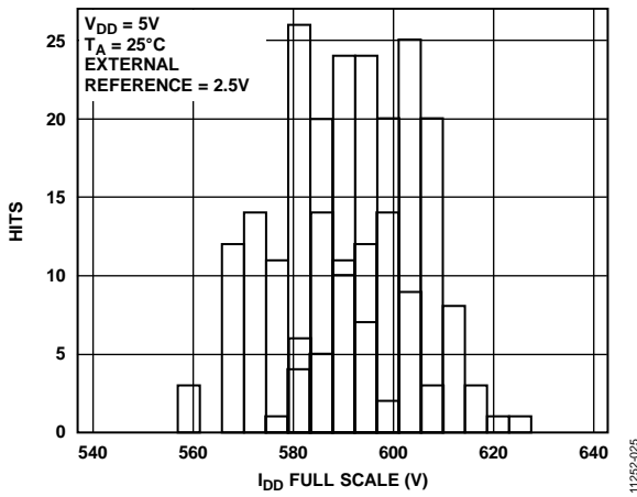
图24. 采用外部基准电压源时的 I_{DD} 直方图
