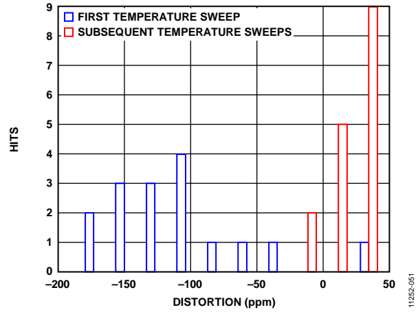
图50. 热滞
