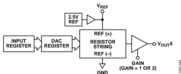
图41. DAC单通道架构框图
