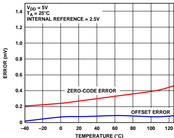
图18. 零代码误差和偏置误差与温度的关系
