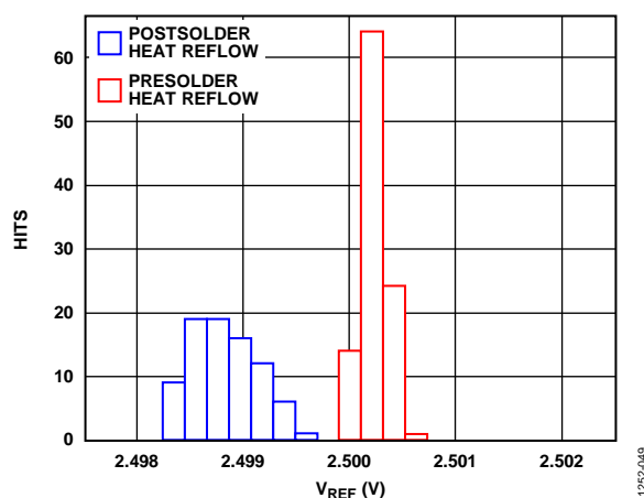
图48. SHR基准电压偏移
