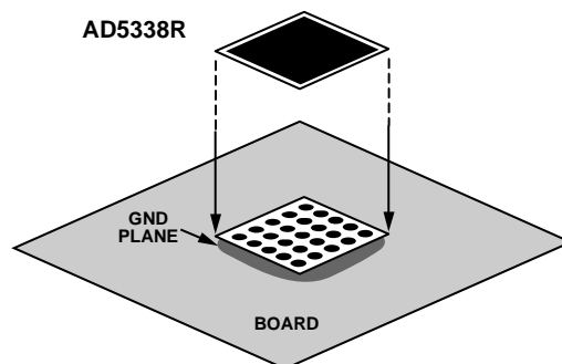
图52. 焊盘与电路板的连接
