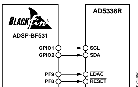
图51. ADSP-BF531与AD5338R接口
