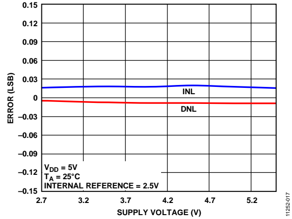
图16. INL误差和DNL误差与电源电压的关系
