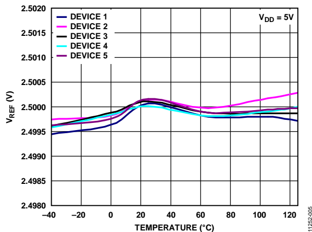
图5. 内部基准电压与温度的关系
