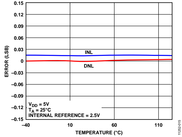
图14. INL误差和DNL误差与温度的关系
