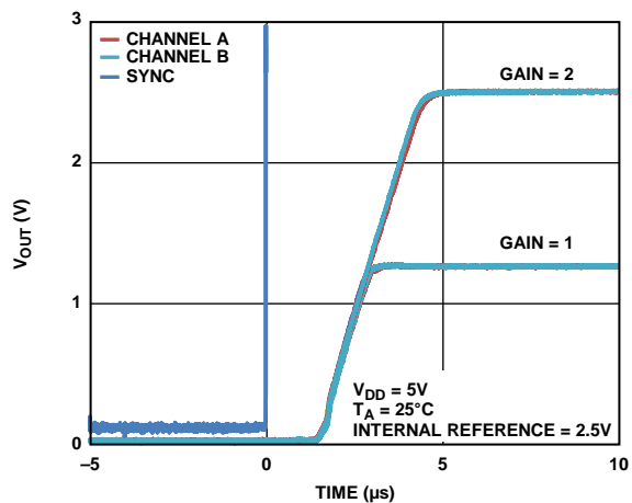
图32. 退出掉电模式进入中间电平
