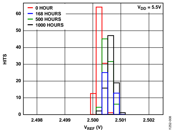
图7. 基准电压源长期稳定性/漂移
