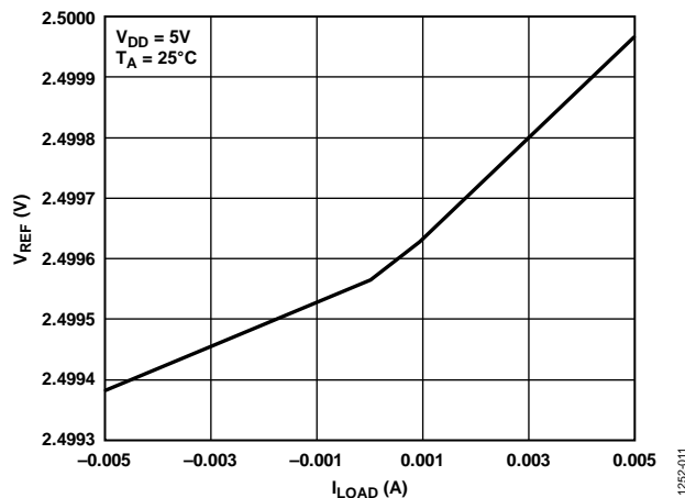
图10. 内部基准电压与负载电流的关系
