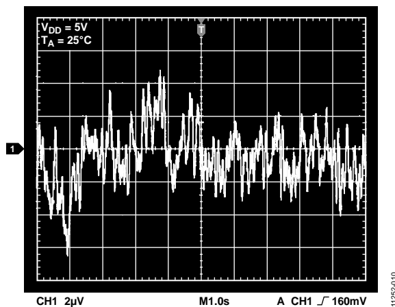
图9. 内部基准电压源噪声(0.1 Hz至10 Hz)
