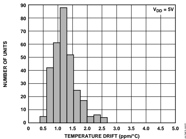
图6. 基准电压输出温度漂移直方图
