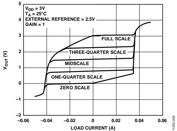
图28. V_{DD} = 3V 时的源电流和吸电流能力
