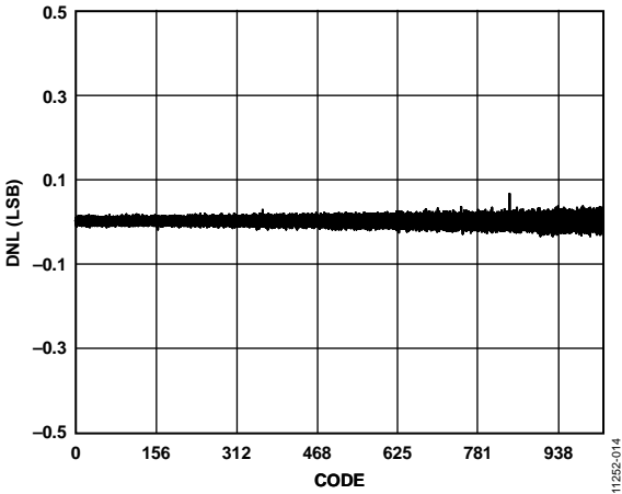
图13. 差分非线性(DNL)
