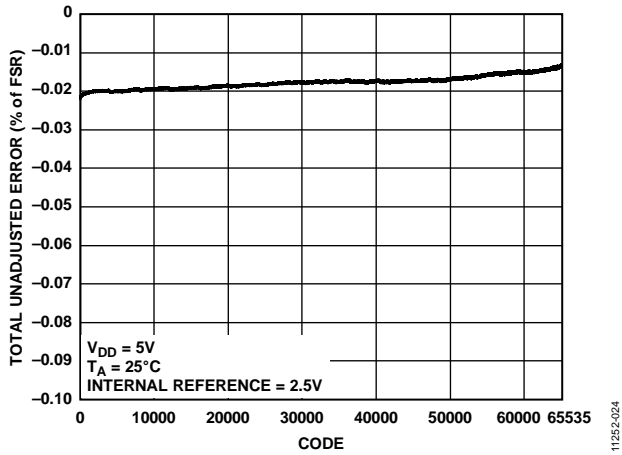
图23. 总不可调整误差与代码的关系
