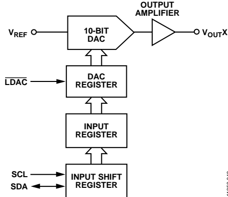
图47. 单个DAC的输入加载电路示意图
