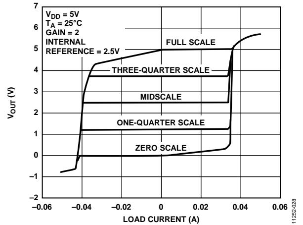
图27. V_{DD} = 5V 时的源电流和吸电流能力
