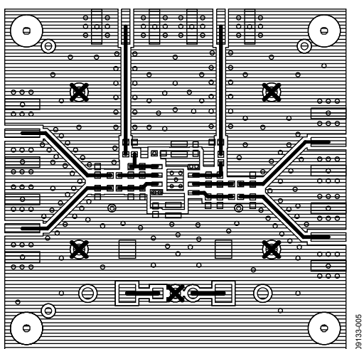
図 5. ボードのレイアウト・パターン—部品面
