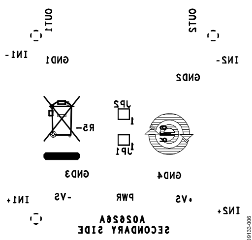
図 6. ボード組立図—回路面
