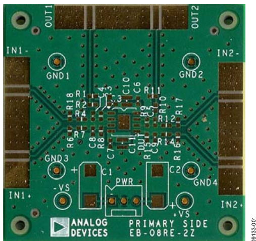
図 1. EB-O8RE-2Z 評価用ボードの部品面
