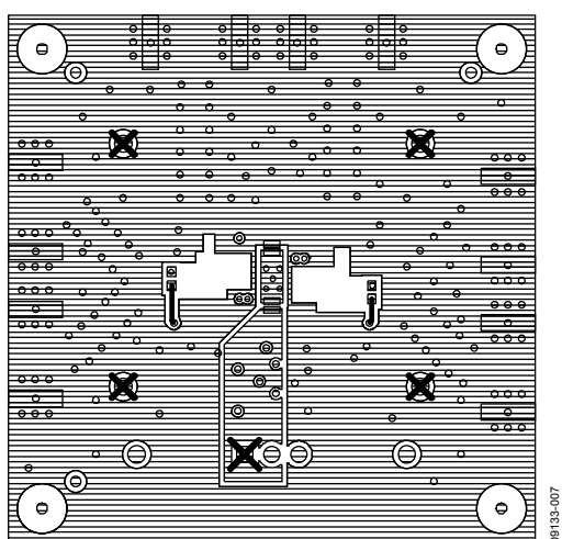
図 7. ボードのレイアウト・パターン—回路面
