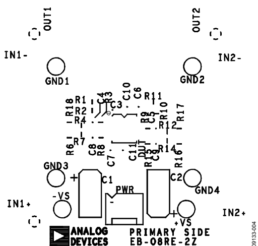
図 4. ボード組立図—部品面
