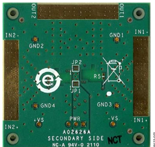
図 2. EB-O8RE-2Z 評価用ボードの回路面
