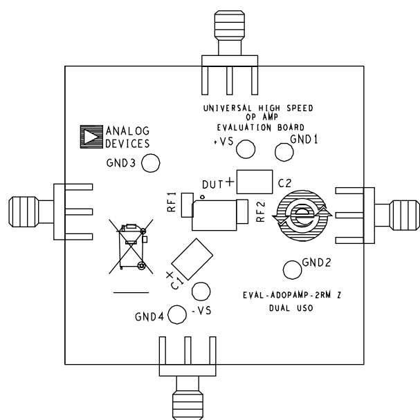
図 4. ボード組立図—部品面
