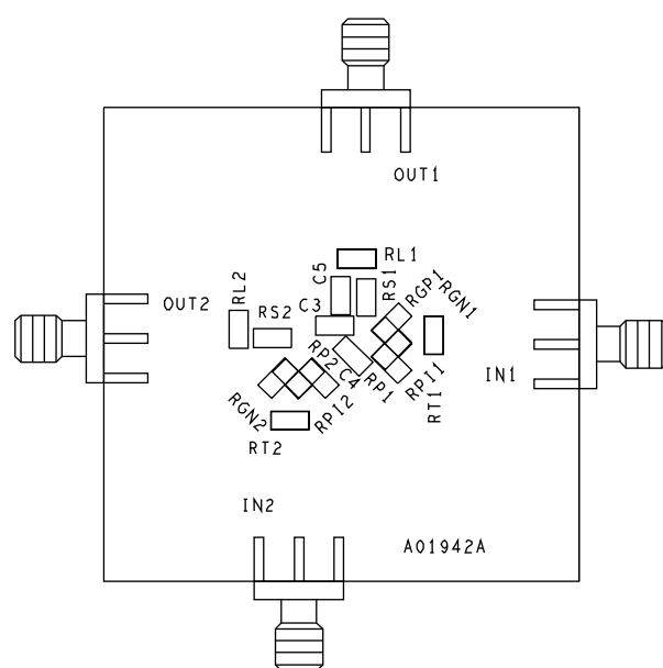
図 6. ボード組立図—回路面
