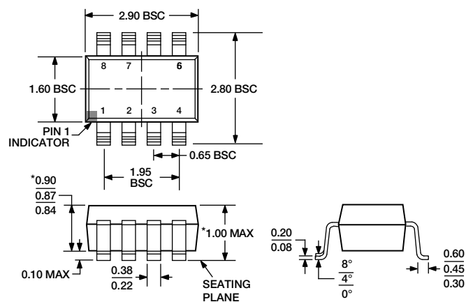
図40. 8ピン薄型スモール・アウトライン・トランジスタ・パッケージ [TSOT] (UJ-8)
