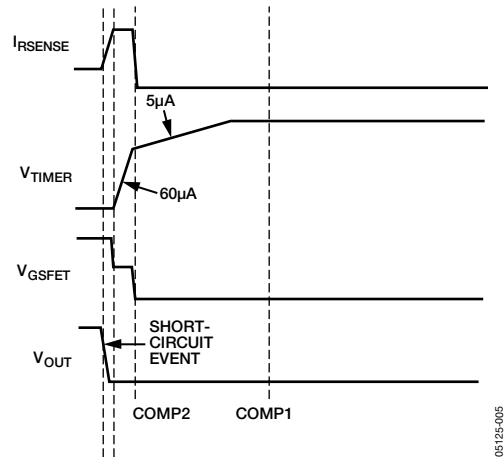
図39. 過電流障害後のADM1171-2のラッチオフ
