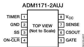
図3. ピン配置 (2AUJモデル)
