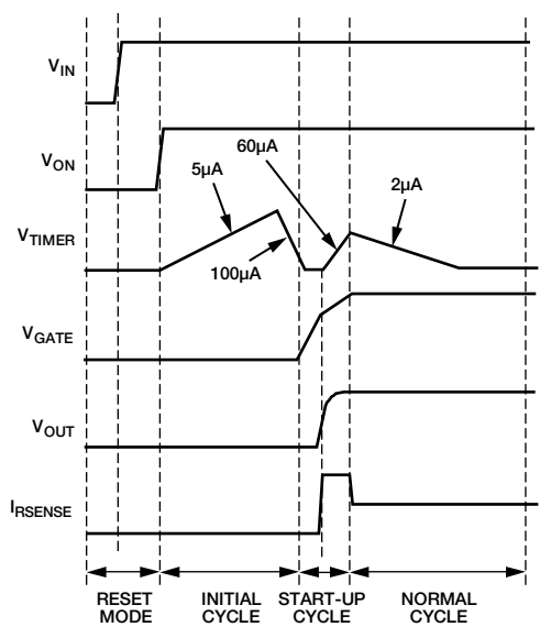
図37. コンデンサのパワーアップ
