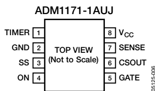
図2. ピン配置 (1AUJモデル)
