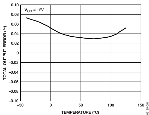
図34. CSOUTの合計出力誤差の温度特性
