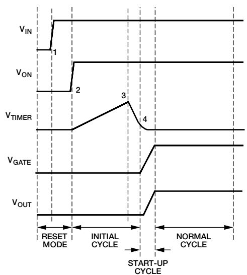
図36. パワーアップのタイミング
