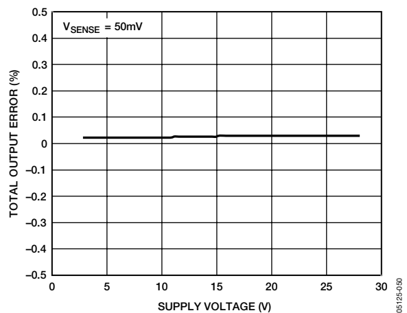
図33. 電源電圧 対 CSOUTの合計出力誤差
