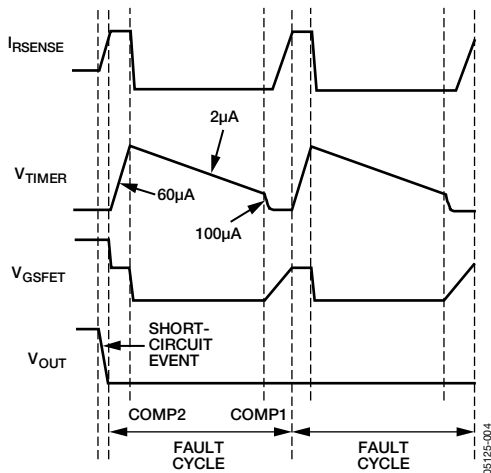
図38. 過電流障害時のADM1171-1の自動再試行
