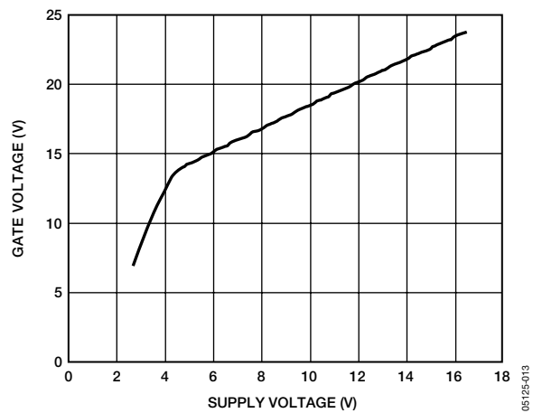
図8. 電源電圧 対 GATE電圧
