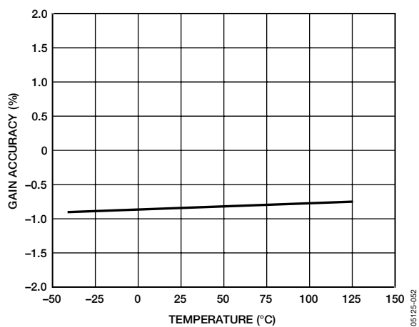
図35. CSOUTのゲイン精度の温度特性
