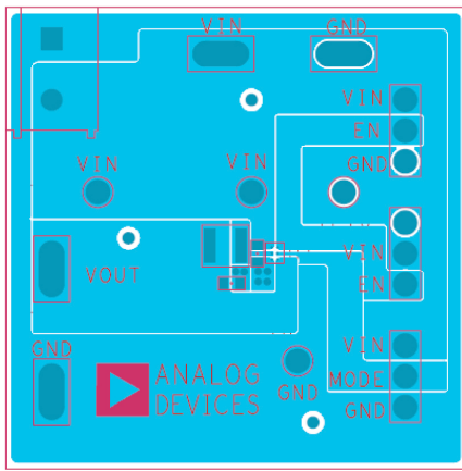
Figure 37. Top Layer
