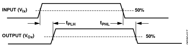
图17. 传播延迟参数
