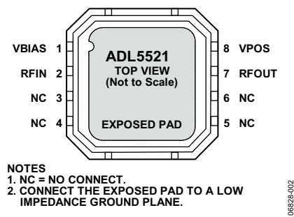
图2. 引脚配置
