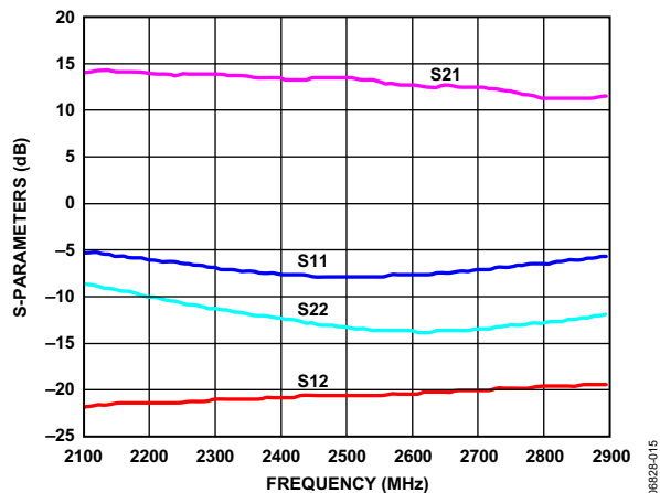
图15. 典型S参数，对数幅度
