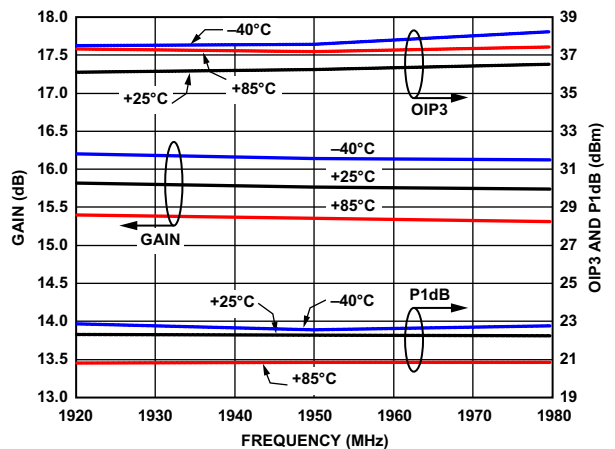
图13. 增益、OIP3和P1dB与温度的关系
