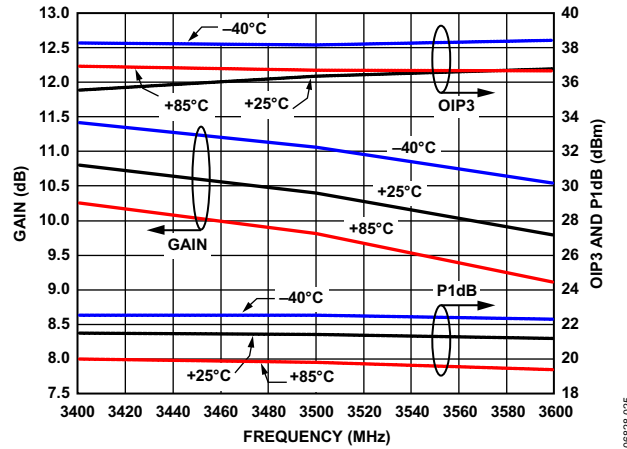
图25. 增益、OIP3和P1dB与温度的关系
