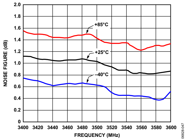
图47. 噪声系数与温度的关系
