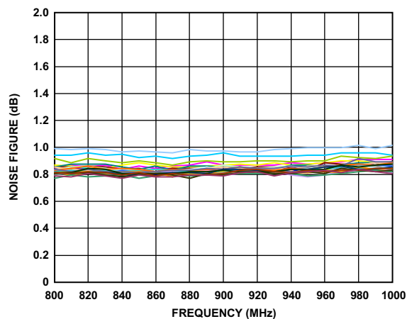
图6. 噪声系数与频率的关系(25°C, 多器件)
