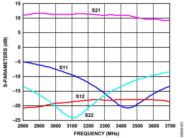
图21. 典型S参数，对数幅度
