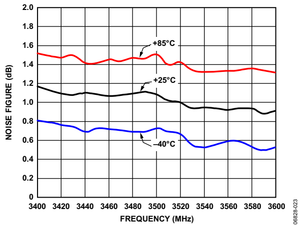
图23. 噪声系数与温度的关系
