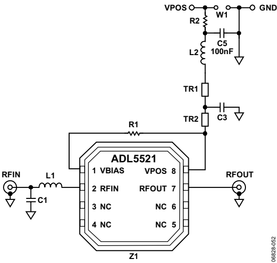
图53. ADL5521基本连接
