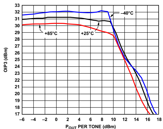
图44. OIP3与输出功率( P_{OUT} )和温度的关系
