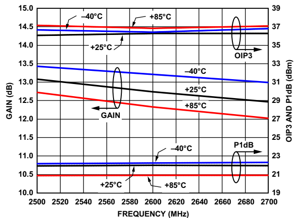
图19. 增益、OIP3和P1dB与温度的关系
