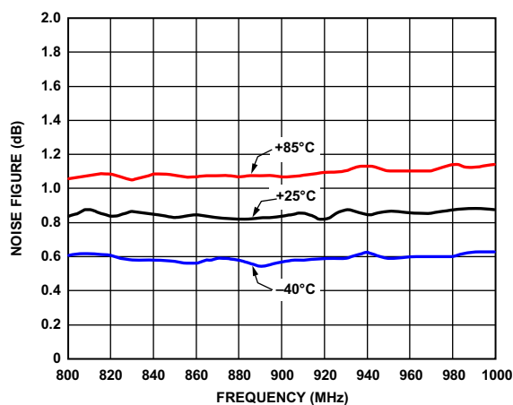
图29. 噪声系数与温度的关系
