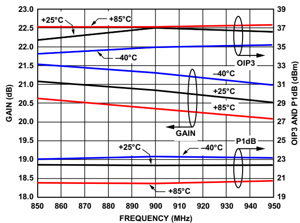
图7. 增益、OIP3和P1dB与温度的关系
