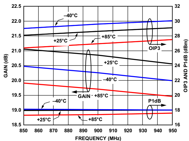
图31. 增益、OIP3和P1dB与温度的关系
