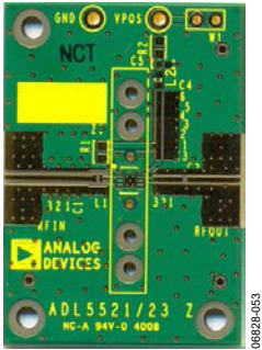
图55. 评估板布局(顶视图)
