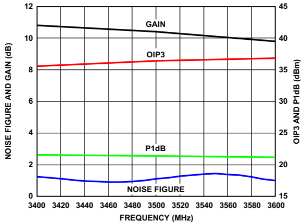
图22. 噪声系数、增益、OIP3和P1dB与频率的关系
