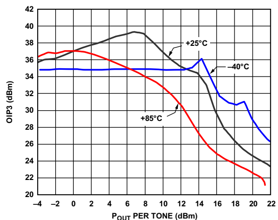
图8. OIP3与输出功率(P OUT )和温度的关系
