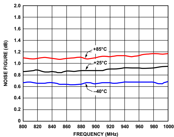
图5. 噪声系数与温度的关系
