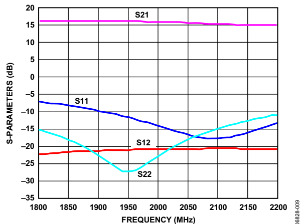
图9. 典型S参数，对数幅度
