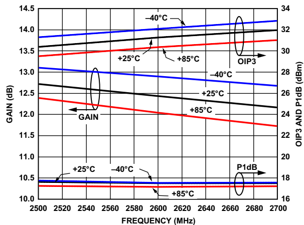
图43. 增益、OIP3和P1dB与温度的关系
