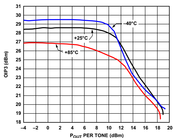
图32. OIP3与输出功率( P_{OUT} )和温度的关系
