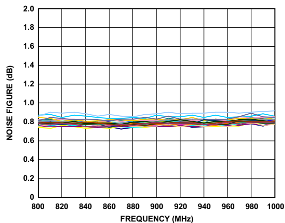
图30. 噪声系数与频率的关系(25°C, 多器件)
