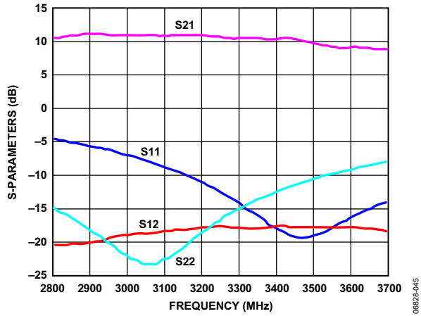
图45. 典型S参数，对数幅度
