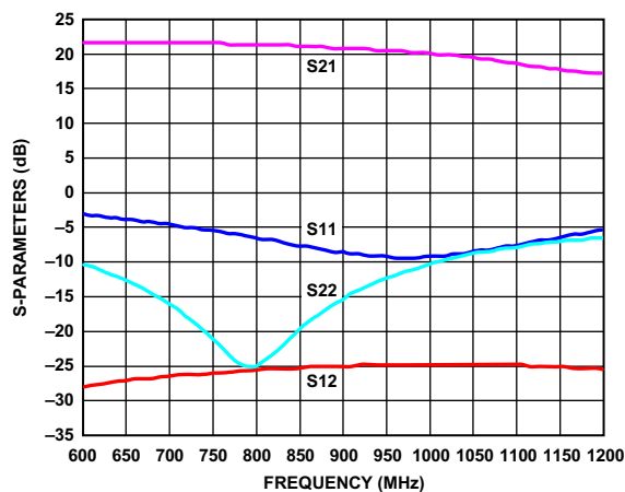
图3. 典型S参数, 对数幅度
