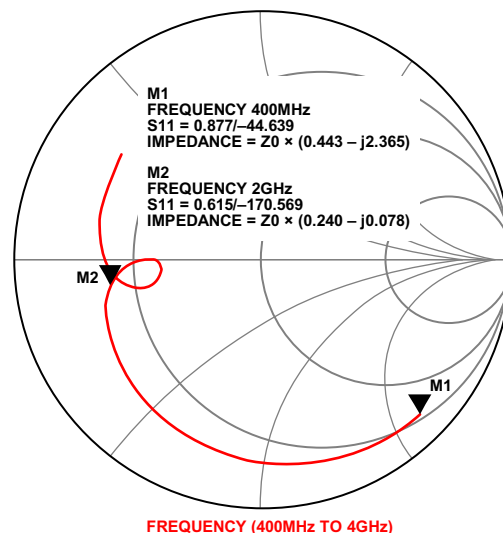
图63. ADL5521的S11(S22为2 GHz匹配)
