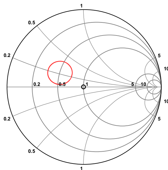
图61. ADL5521的最佳噪声匹配区域
