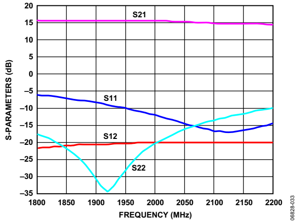
图33. 典型S参数，对数幅度
