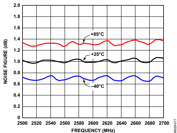
图17. 噪声系数与温度的关系
