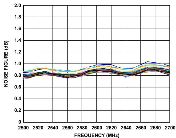
图42. 噪声系数与频率的关系(25°C, 多器件)
