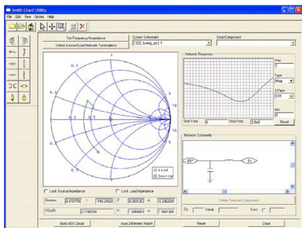
图62. \Gamma_{OPT} 的串联电感、分流电容匹配网络示例
