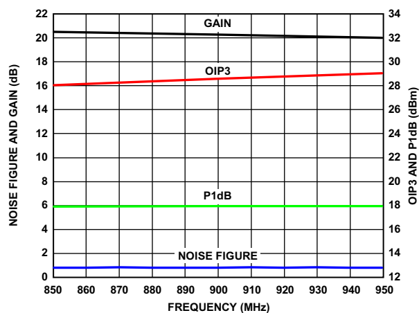
图28. 噪声系数、增益、OIP3和P1dB与频率的关系
