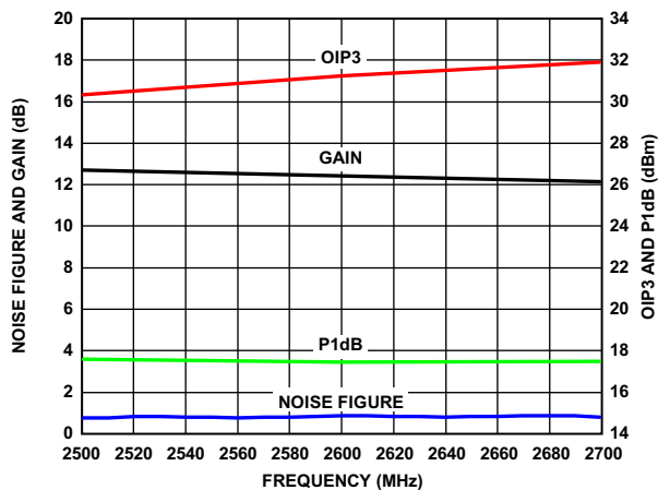
图40. 噪声系数、增益、OIP3和P1dB与频率的关系
