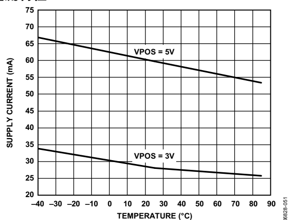
图51. 电源电流与温度的关系(3 V和5 V)
