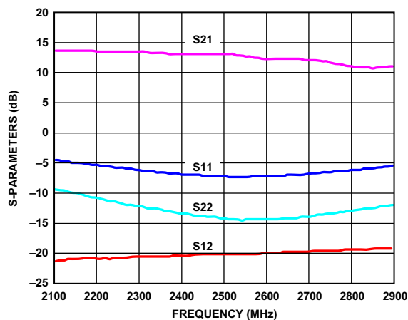
图39. 典型S参数, 对数幅度
