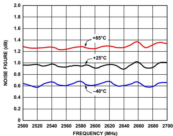
图41. 噪声系数与温度的关系
