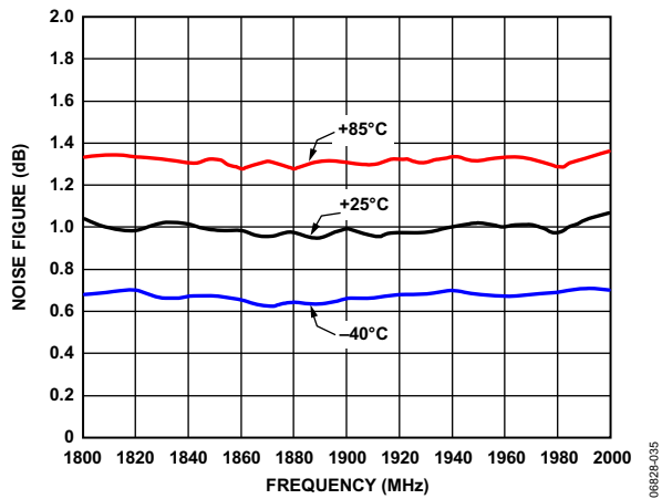
图35. 噪声系数与温度的关系
