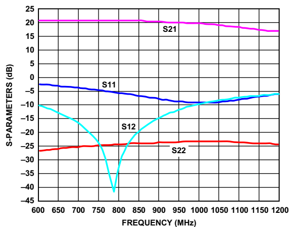
图27. 典型S参数，对数幅度
