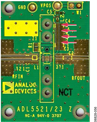
图58. LNA评估板的PCB布局(注意偏置线路上针对S22调谐的滑块和电容放置，图中标出箭头)
