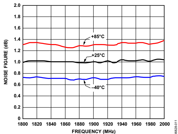
图11. 噪声系数与温度的关系
