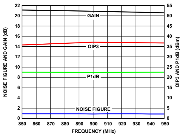
图4. 噪声系数、增益、OIP3和P1dB与频率的关系
