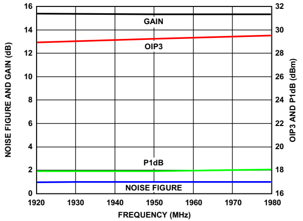
图34. 噪声系数、增益、OIP3和P1dB与频率的关系
