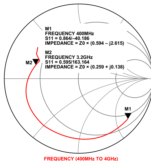
图64. ADL5521的S11(S22为3.2 GHz匹配)
