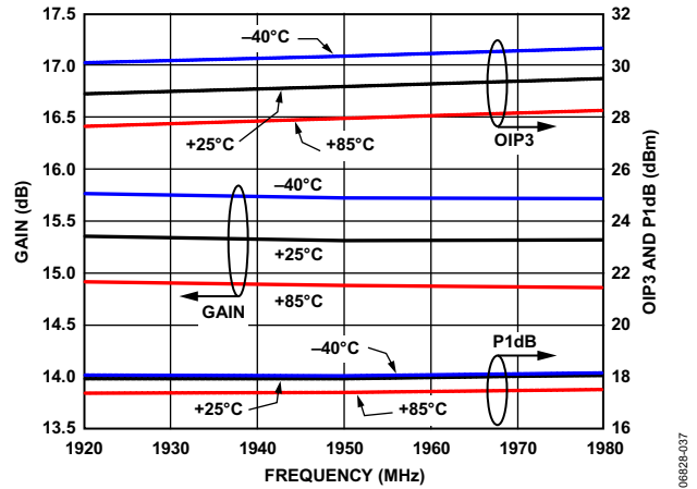
图37. 增益、OIP3和P1dB与温度的关系
