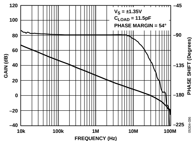
图50. 开环增益和相位与频率的关系
