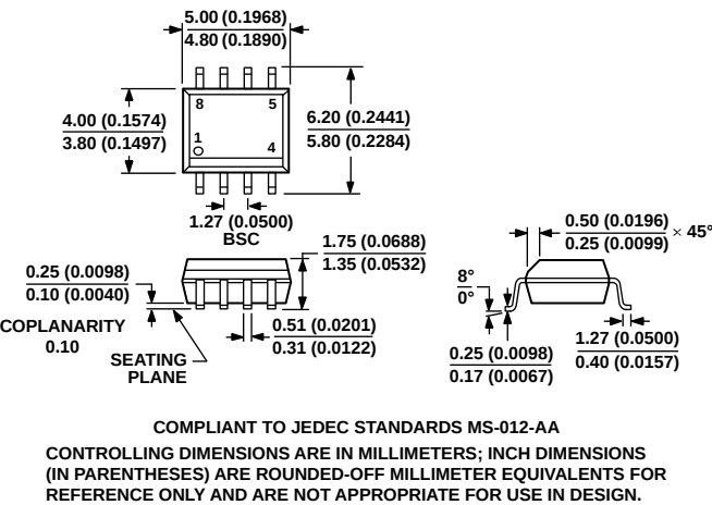
图61. 8引脚标准小型封装[SOIC_N] 窄体(R-8) 图示尺寸单位: mm和(inch)
