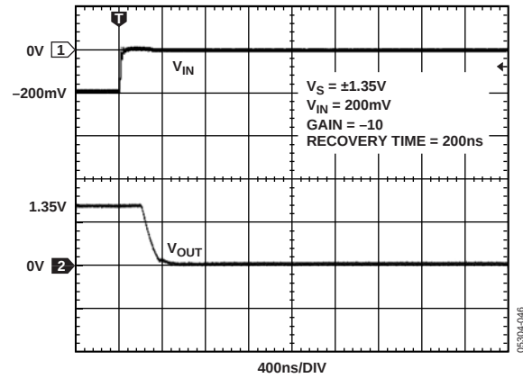
图46. 正过载恢复时间
