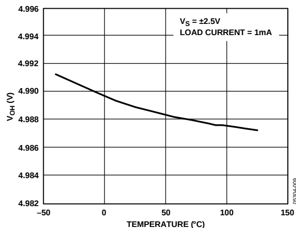
图14. 输出电压高摆幅与温度的关系
