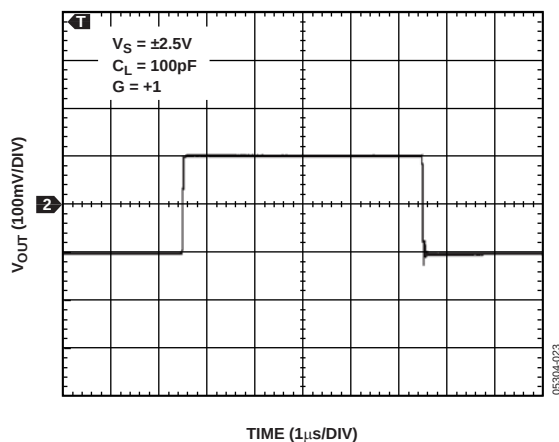
图28. 小信号响应
