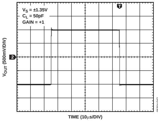
图42. 大信号响应
