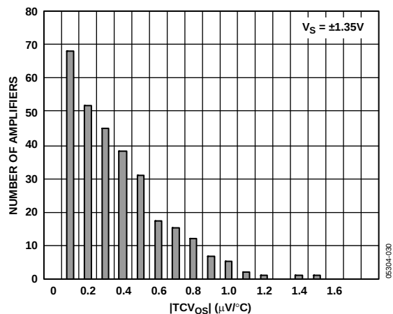
图35. |TCV_{OL}| 的分配
