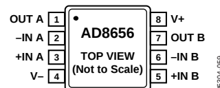
图2. AD8656 8 引脚 MSOP(RM-8)
