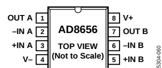
图4. AD8656 8 引脚 SOIC (R-8)
