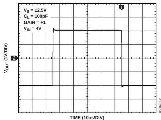
图27. 大信号响应
