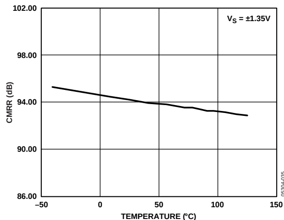
图48. 大信号CMRR与温度的关系
