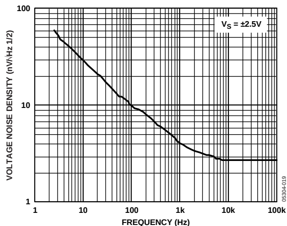
图20. 电压噪声密度与频率的关系
