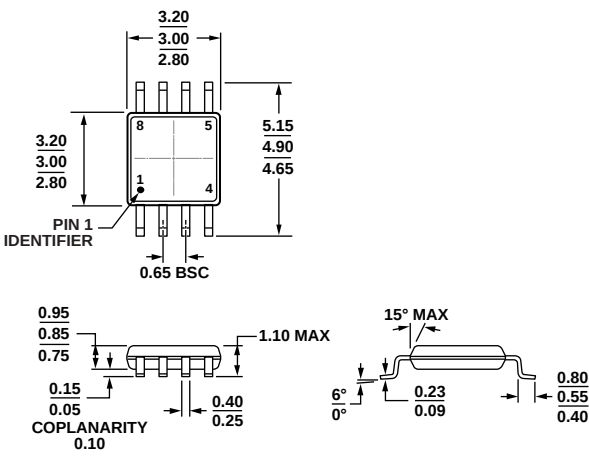
图62. 8引脚超小型MSOP封装 (RM-8) 图示尺寸单位: mm
