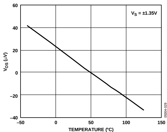
图34. 输入失调电压与温度的关系
