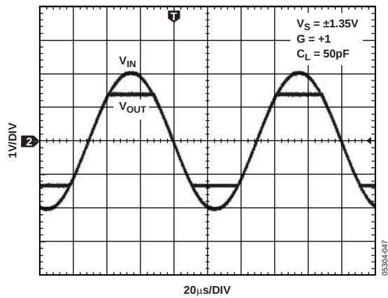
图41. 无相位反转
