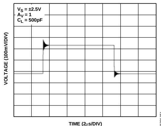
图56. 无补偿驱动高容性负载
