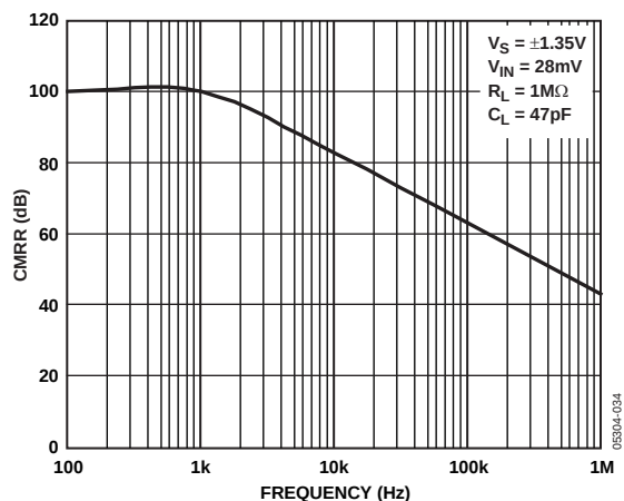
图47. CMRR与频率的关系
