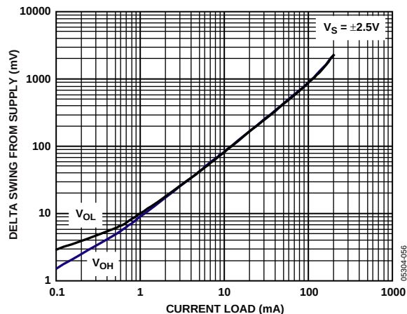
图13. AD8656输出摆幅与电流负载的关系
