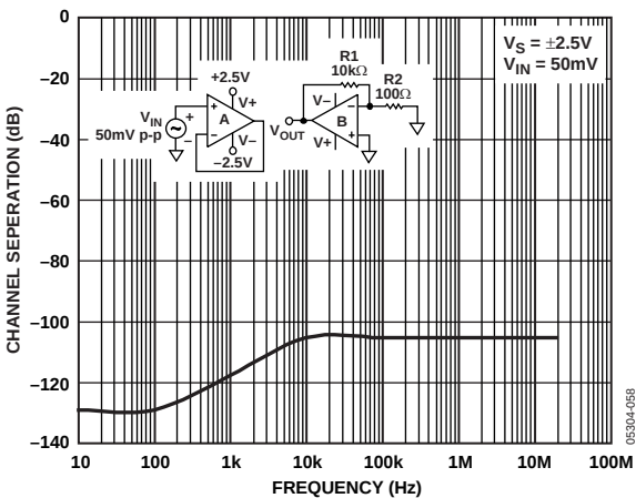
图55. 通道隔离与频率的关系
