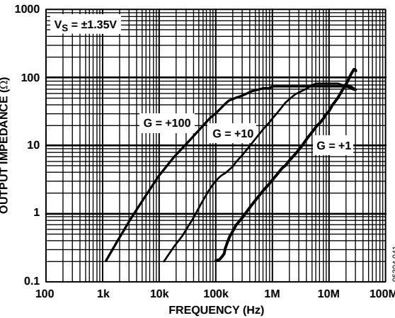
图54. 输出阻抗与频率的关系
