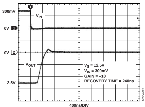
图30. 负过载恢复时间
