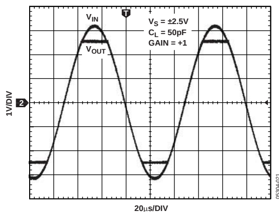
图22. 无相位反转
