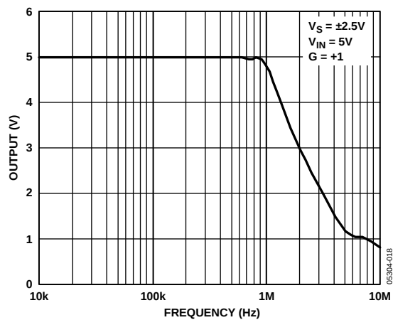
图26. 最大输出摆幅与频率的关系
