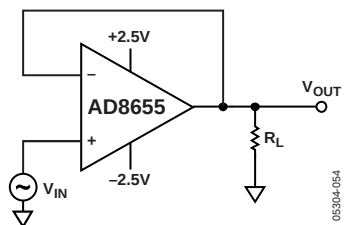
图59. THD + N测试电路
