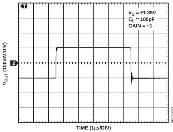
图43. 小信号响应
