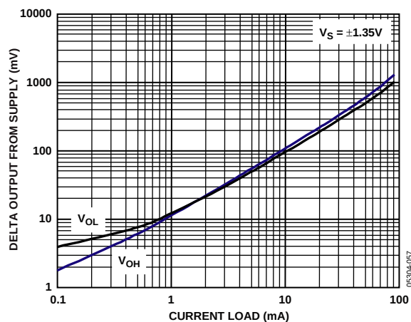
图38. AD8656输出摆幅与电流负载的关系
