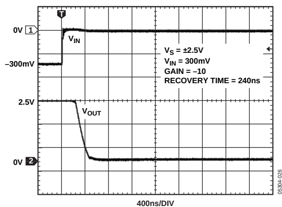
图31. 正过载恢复时间
