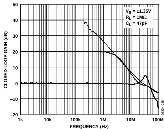
图52. 闭环增益与频率的关系
