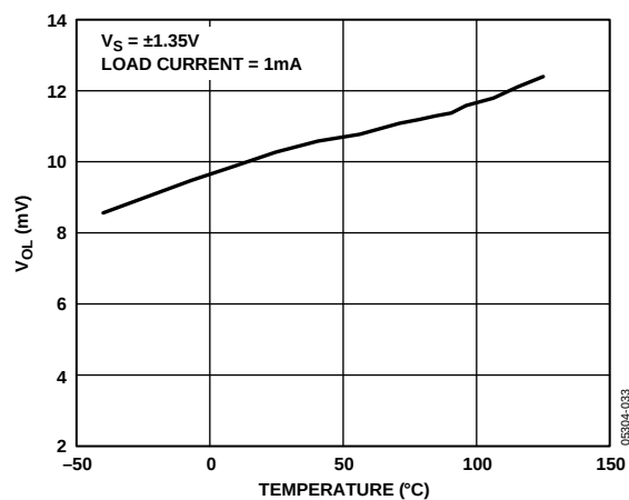
图40. 输出电压低摆幅与温度的关系
