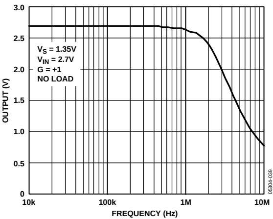
图53. 最大输出摆幅与频率的关系
