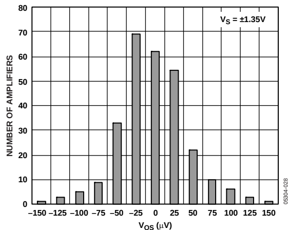
图33. 输入失调电压分布图
